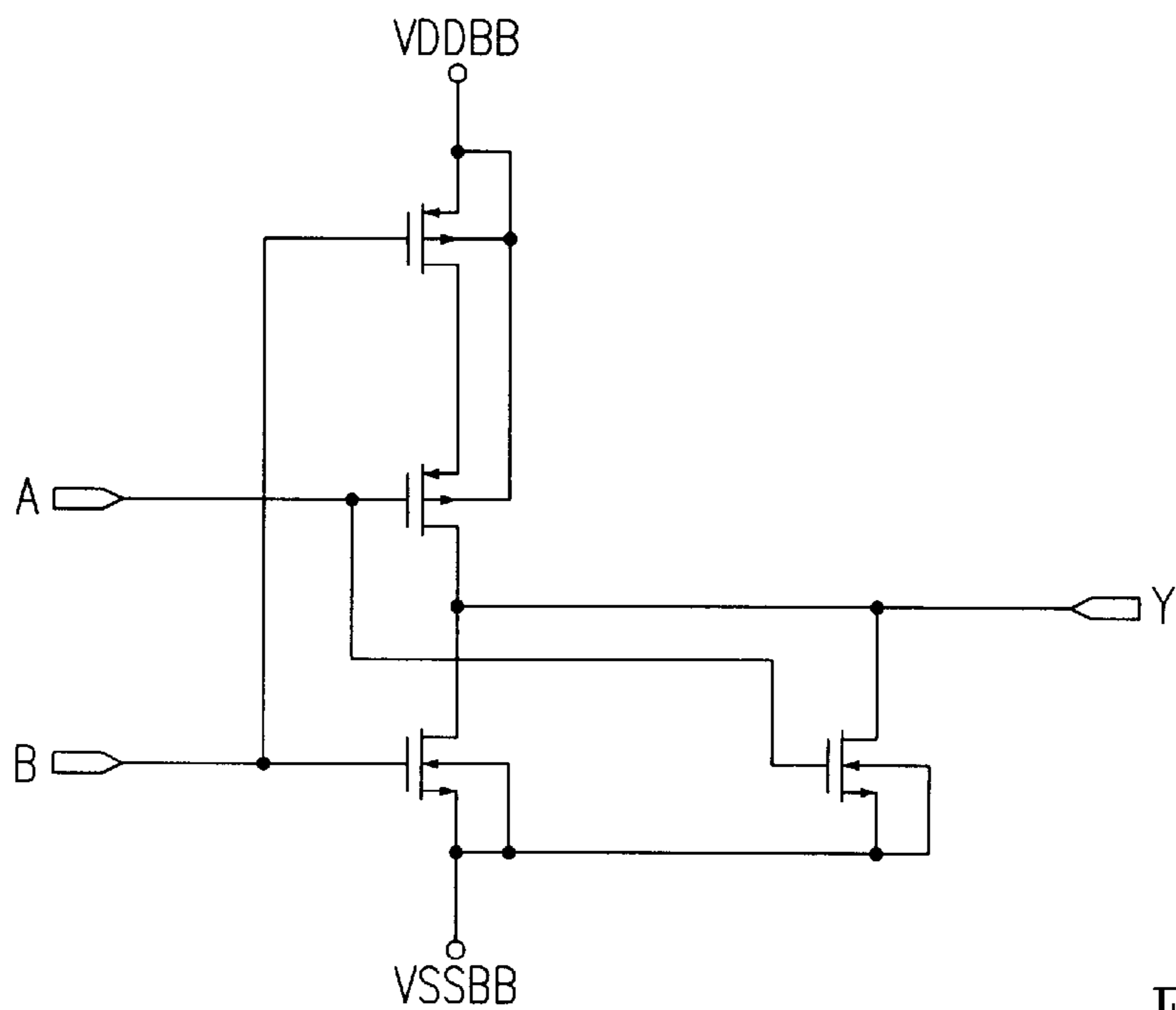
NOR2
