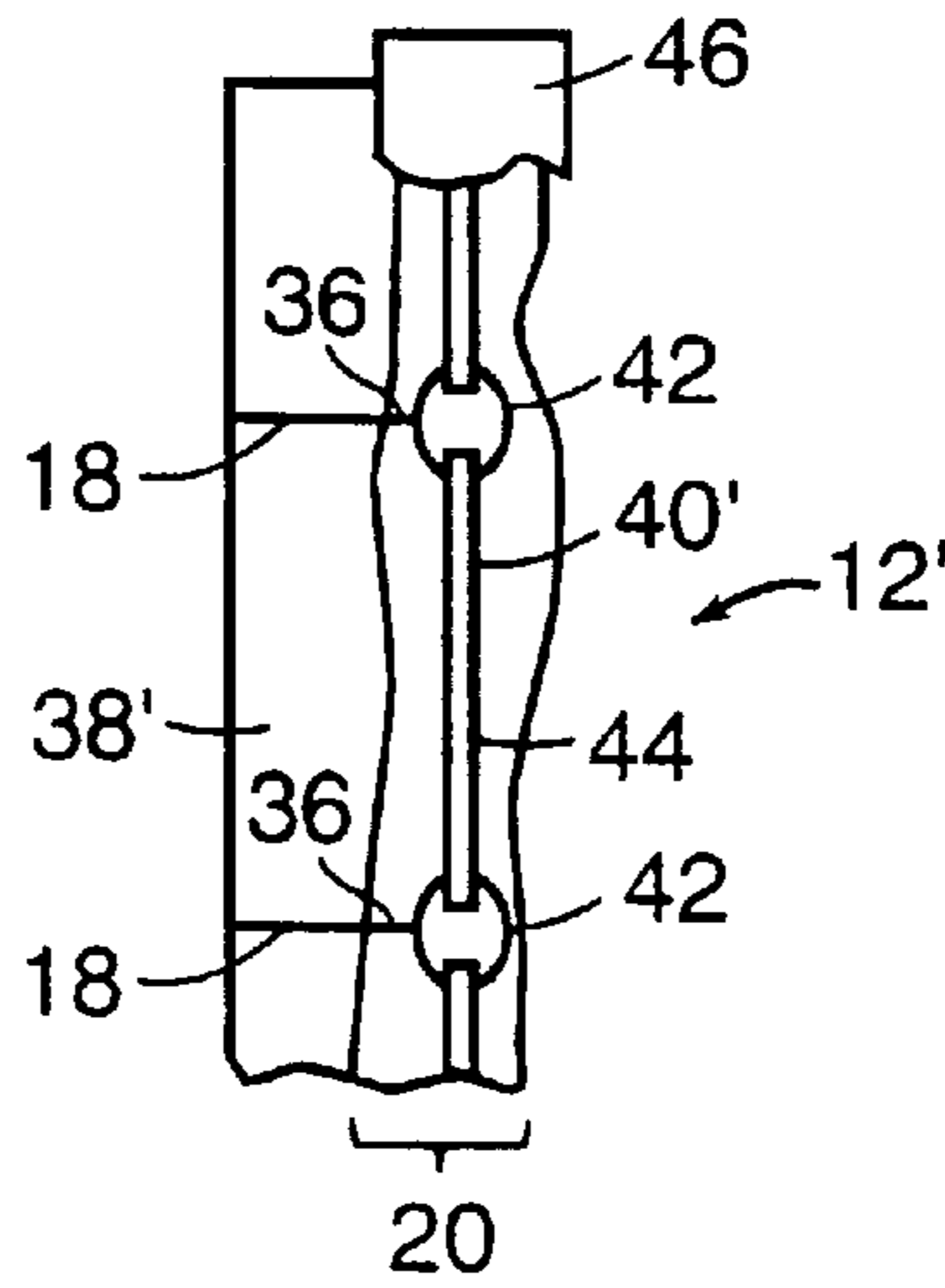
FIG. 20
