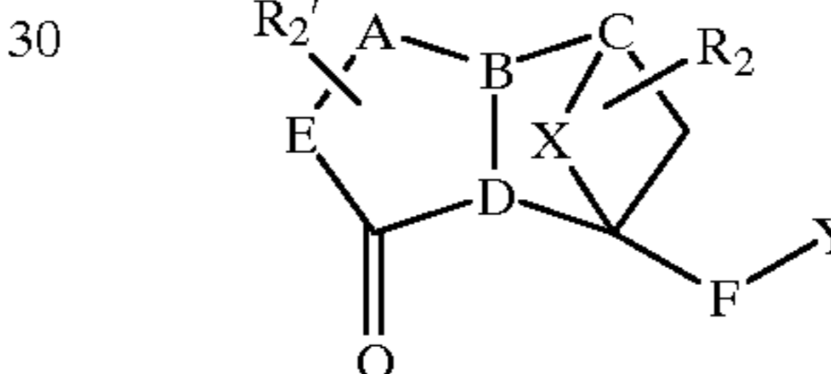
(VIII)
