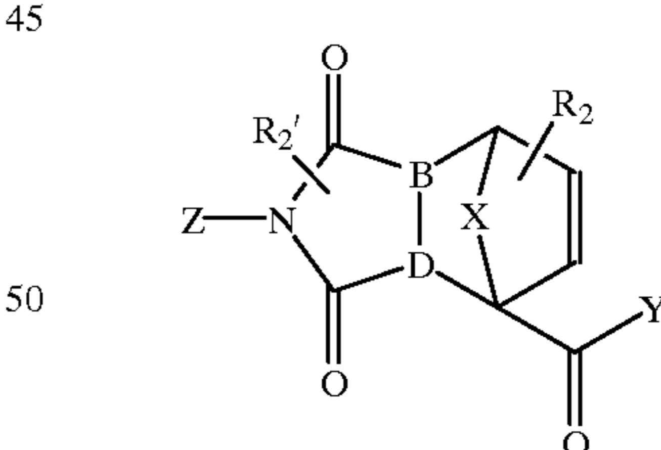
(VIIIa)
