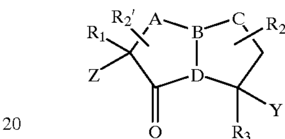
(VII)
