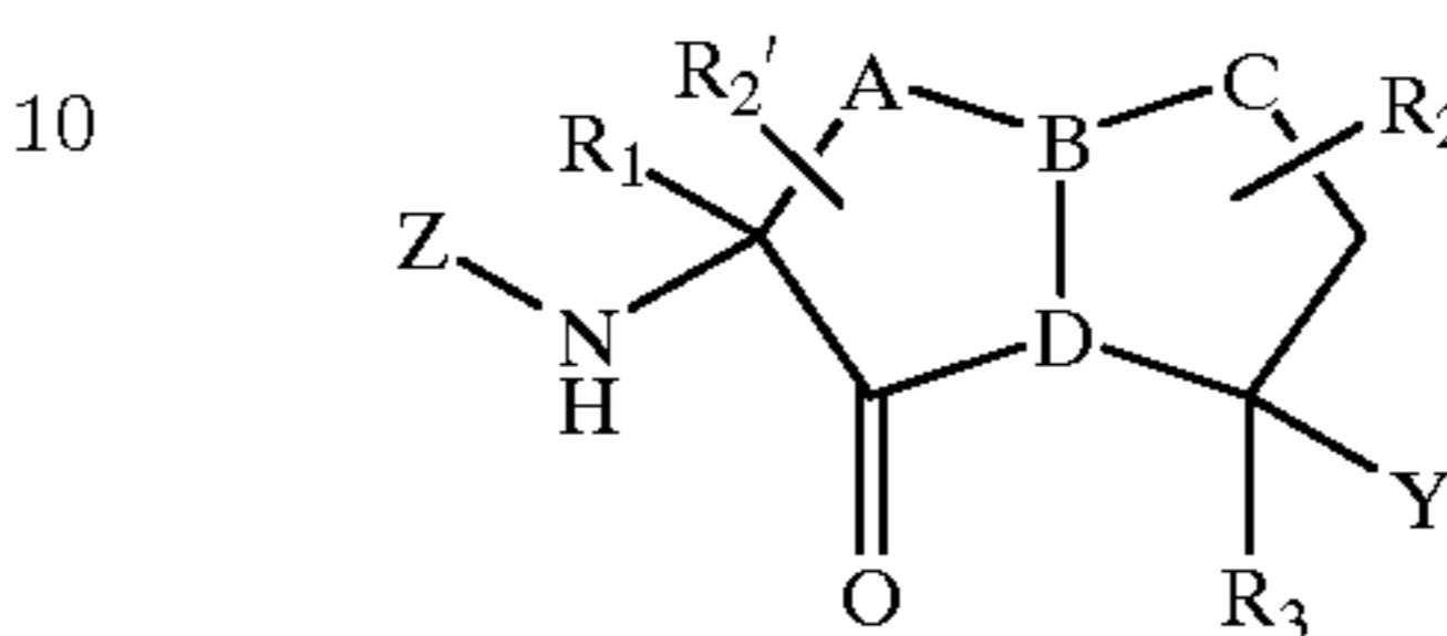
(VI)
