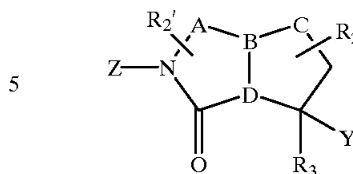
(V)
