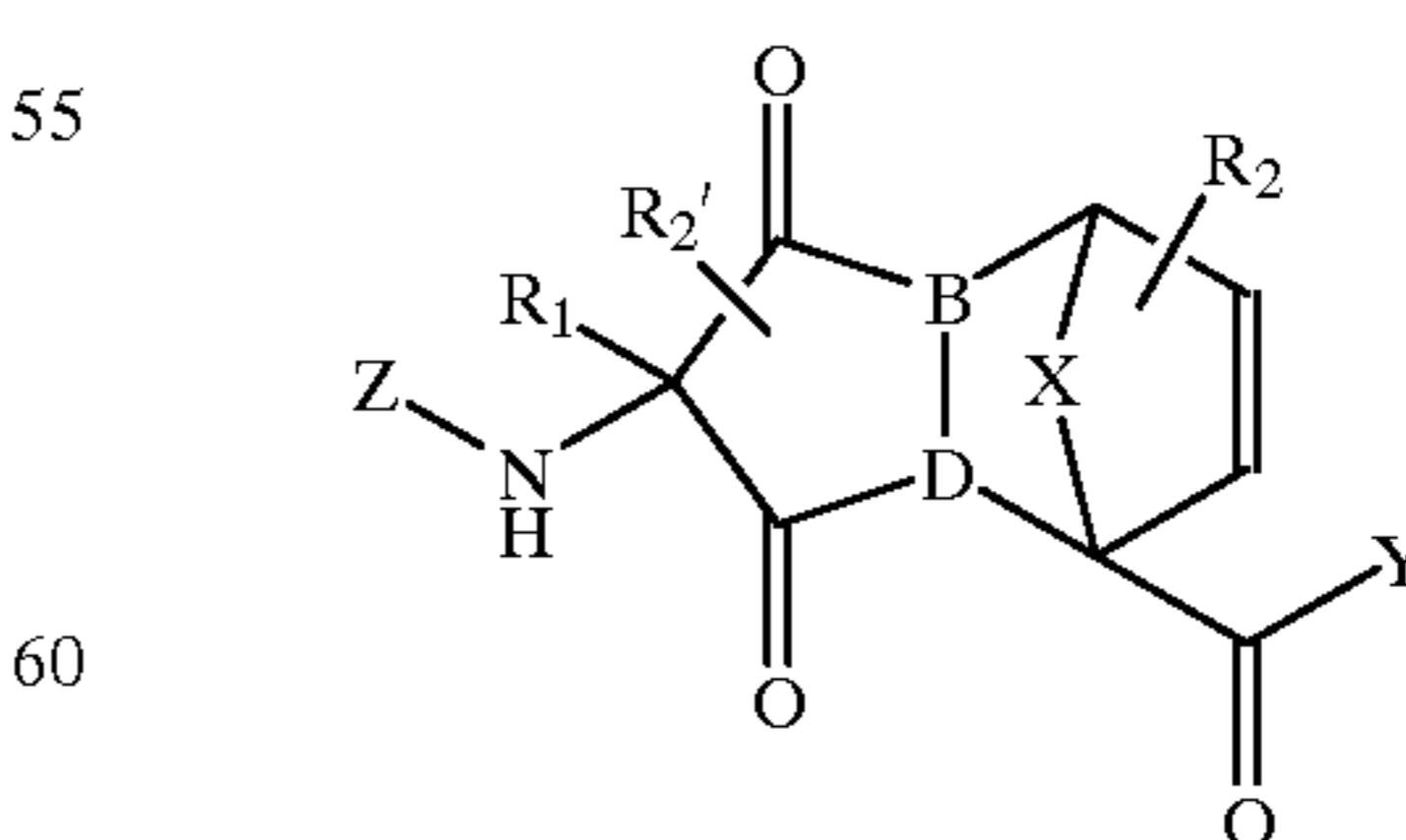
(VIIIb)
