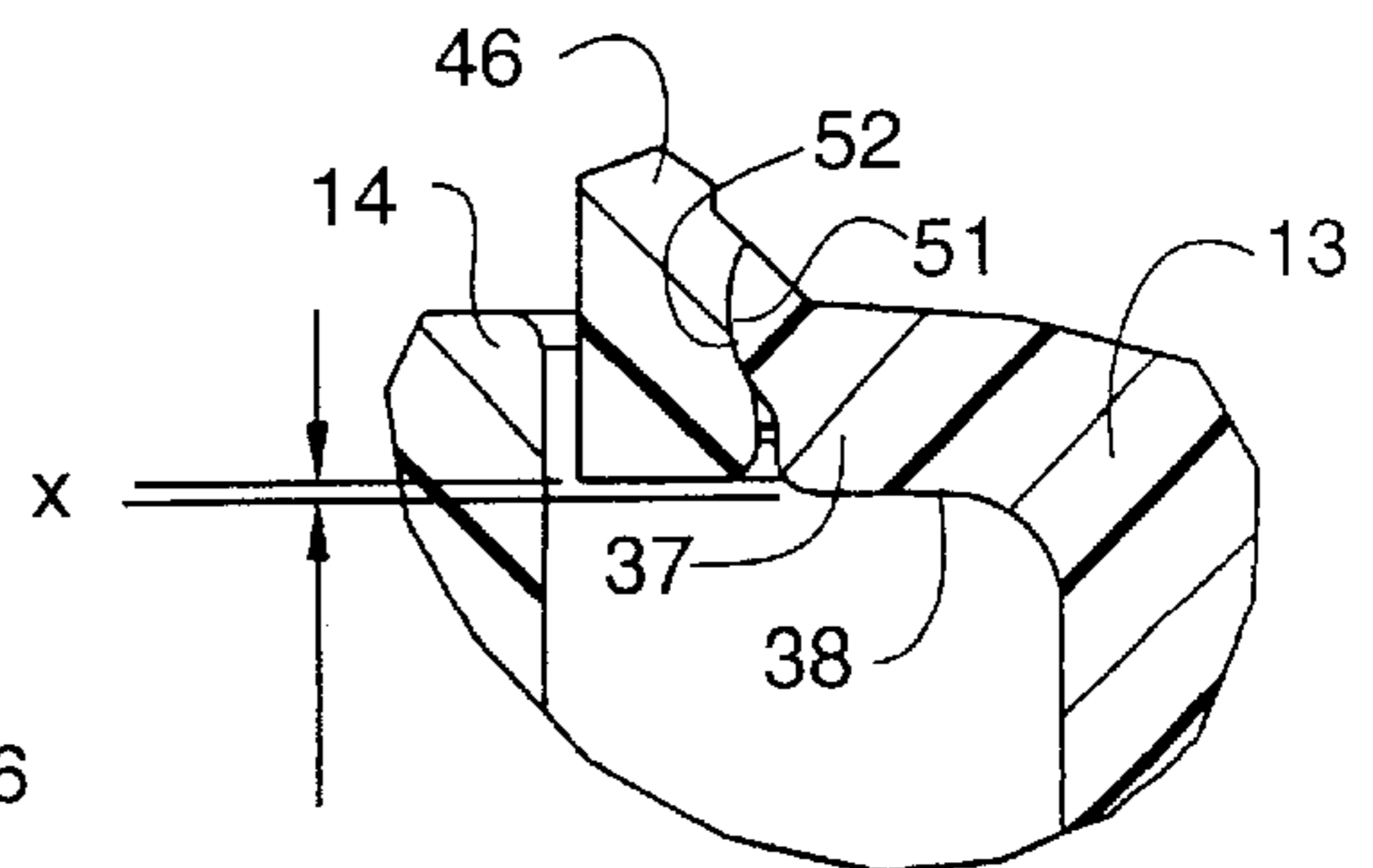
FIG. 3A.
