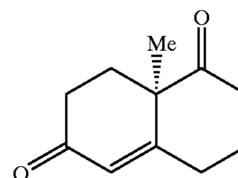
Wieland-Miescher Ketone (3)
