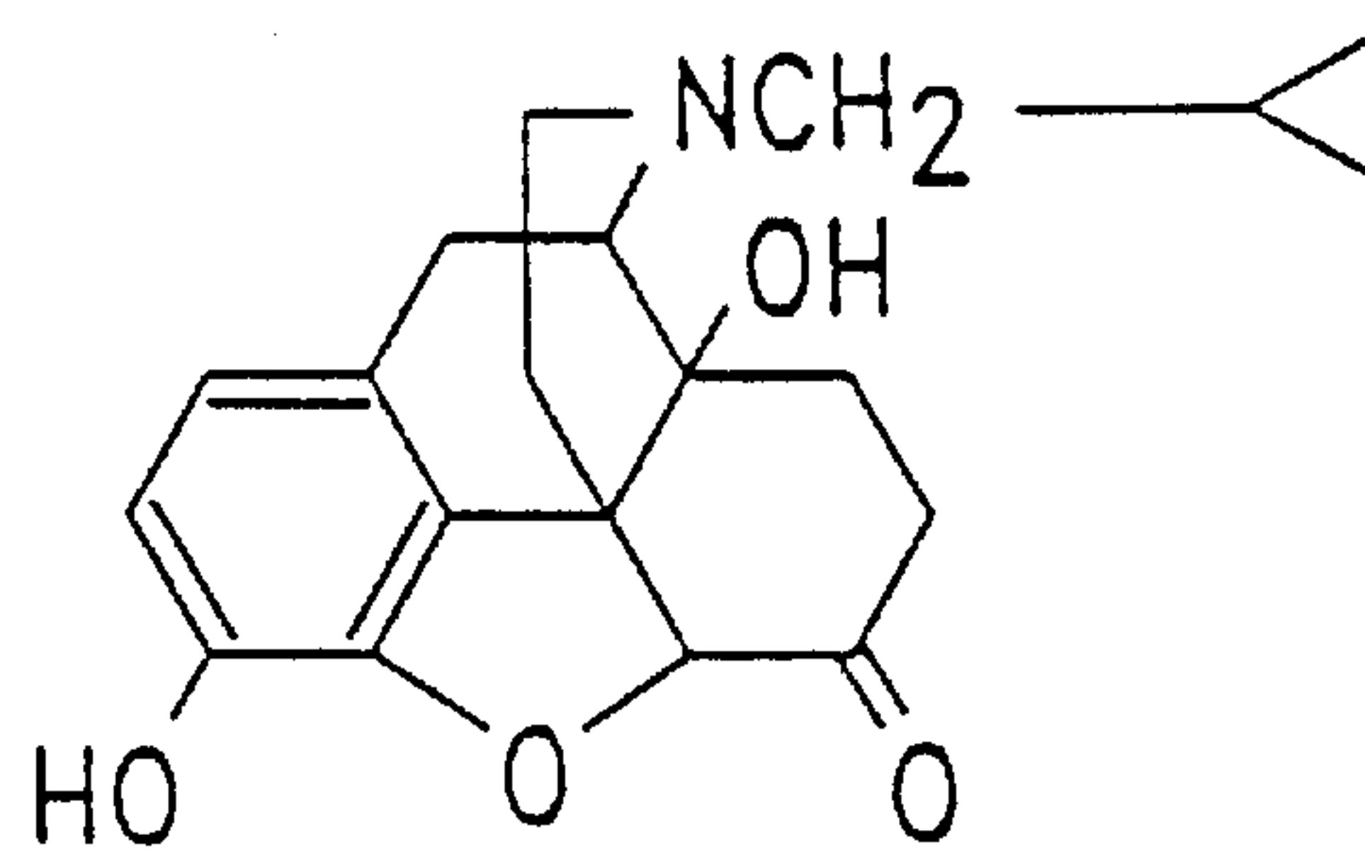
Naltrexone (R=O)
