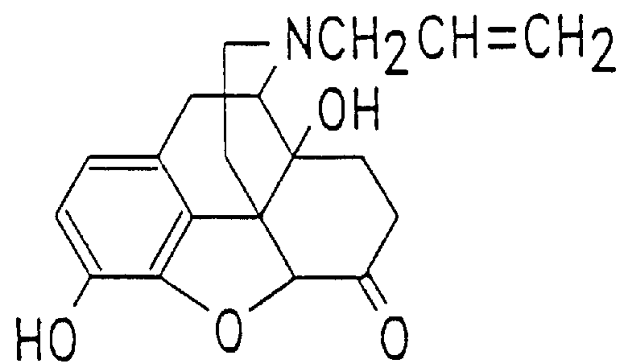
Naloxone
