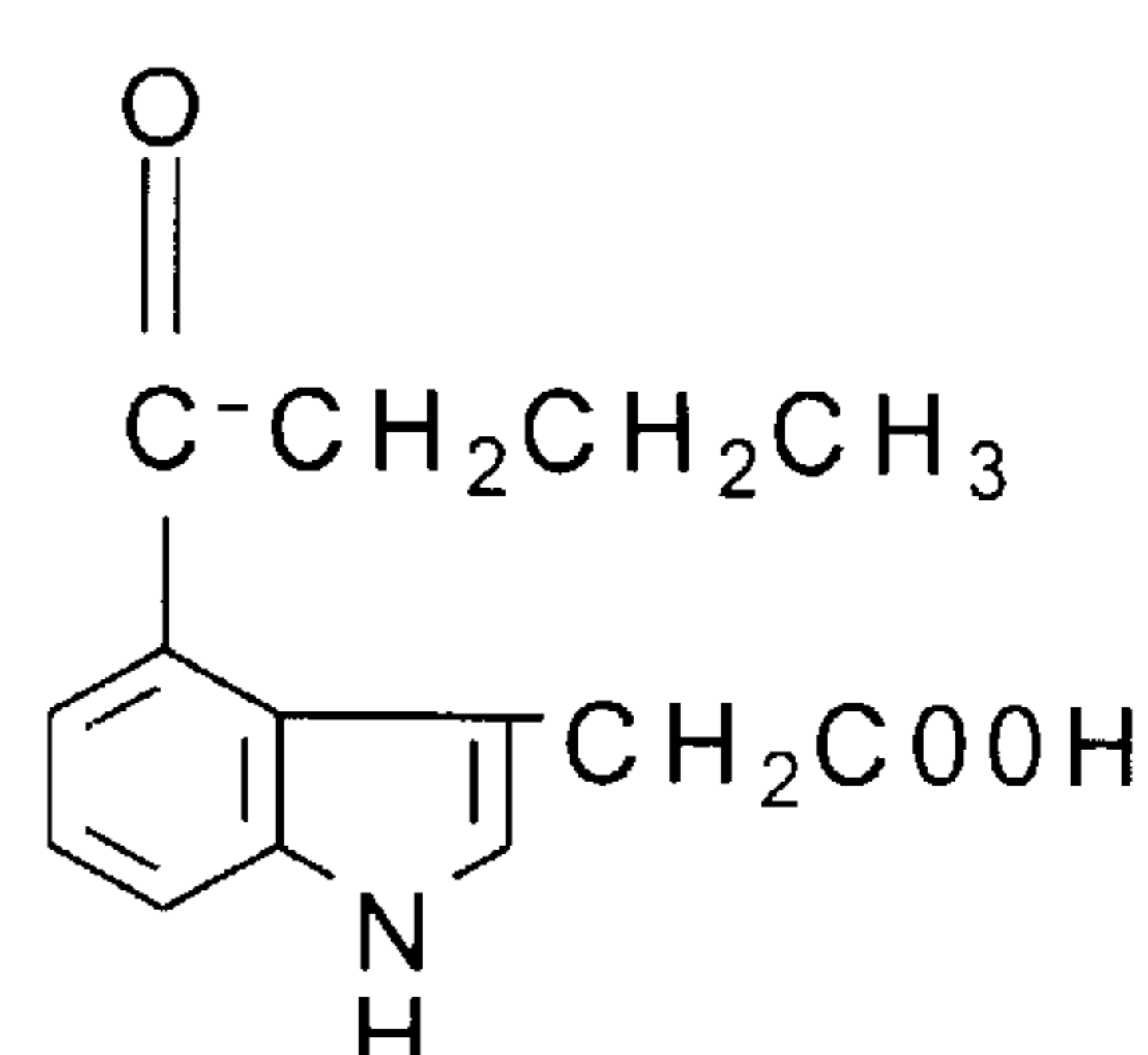
4-butyryl-IAA
