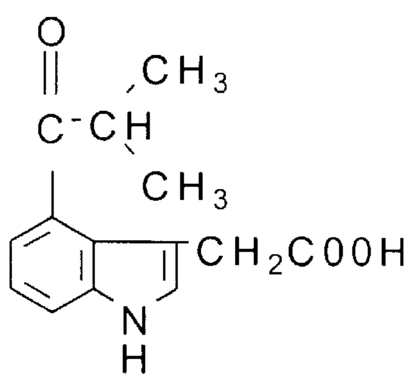
4-isobutyryl-IAA
