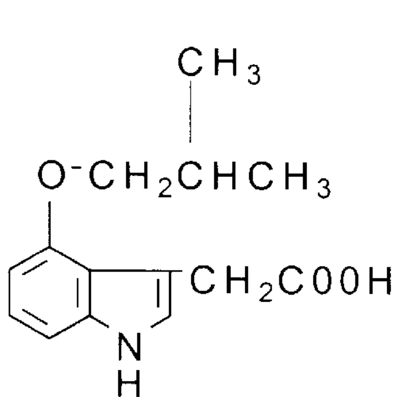
4-isobutoxy-IAA
