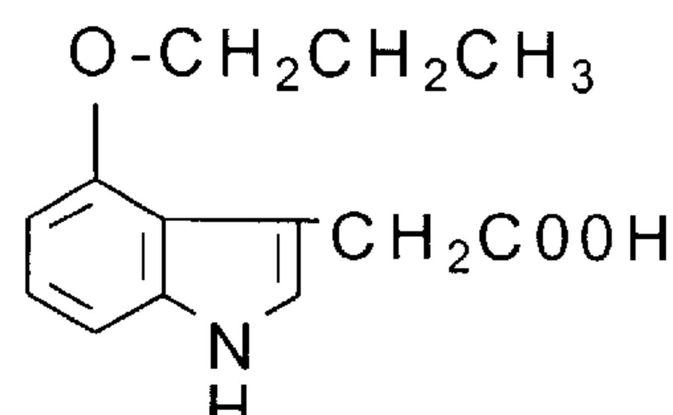
4-propoxy-IAA
