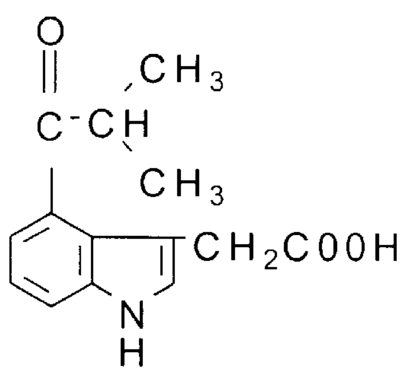
4-isobutyryl-IAA
