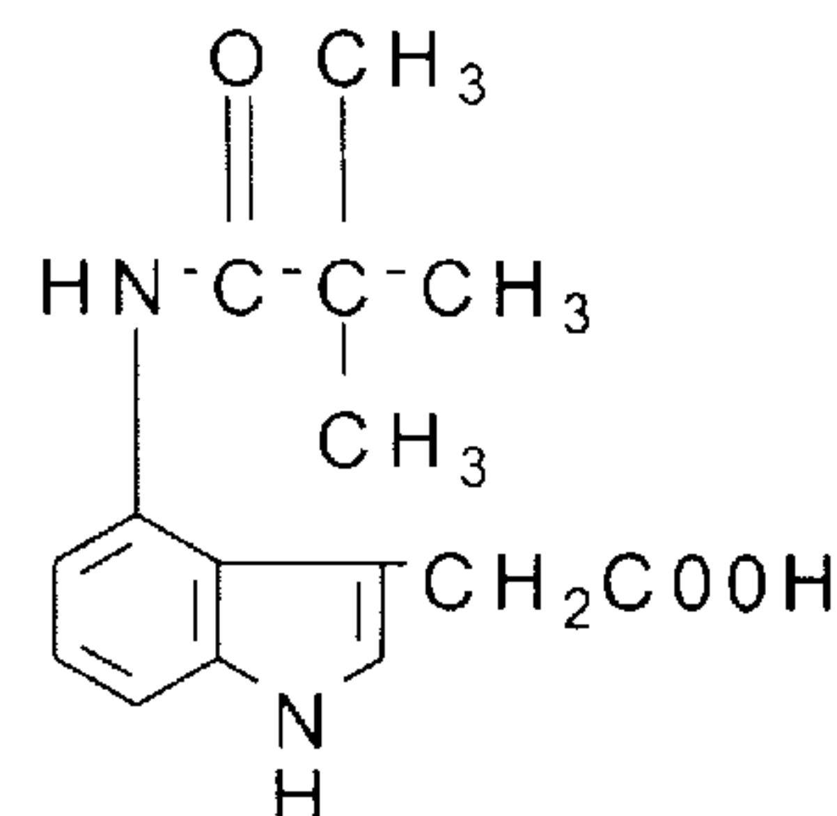
4-tert-valerylamido-IAA
