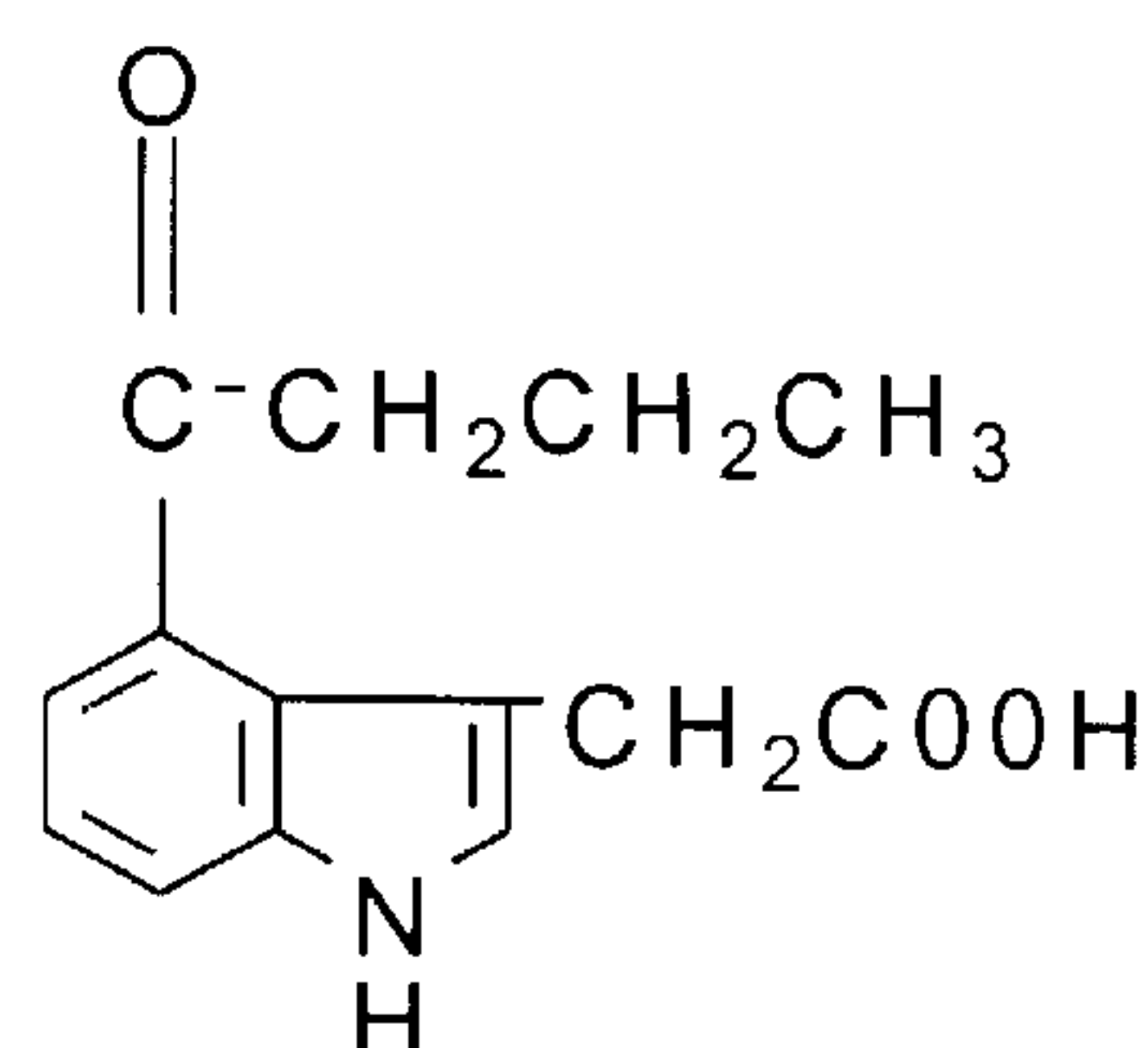
4-butyryl-IAA
