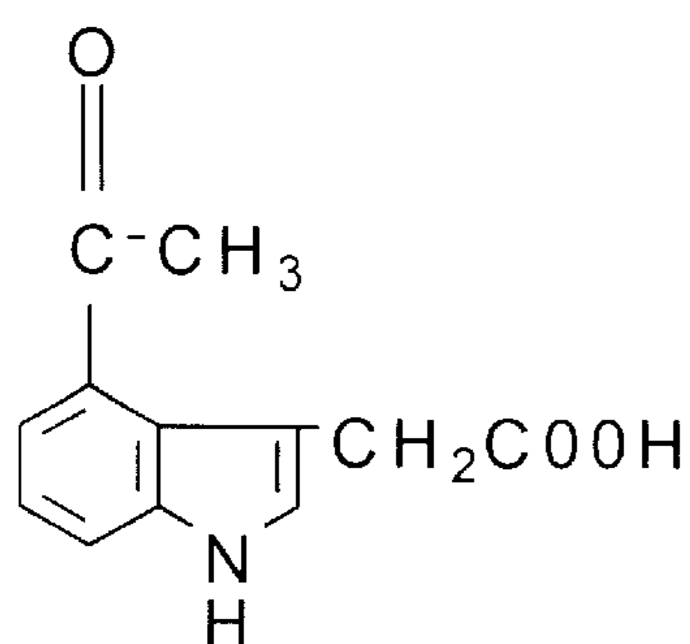
4-acetyl-IAA
