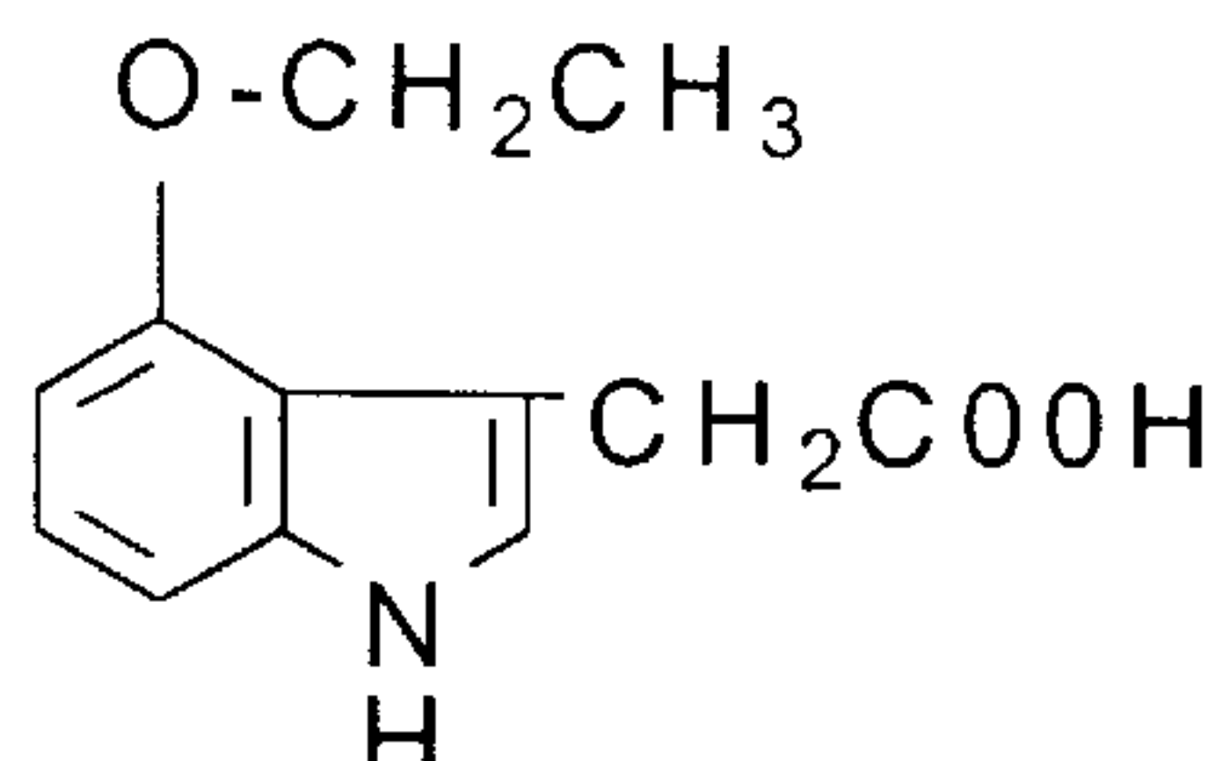
4-ethoxy-IAA
