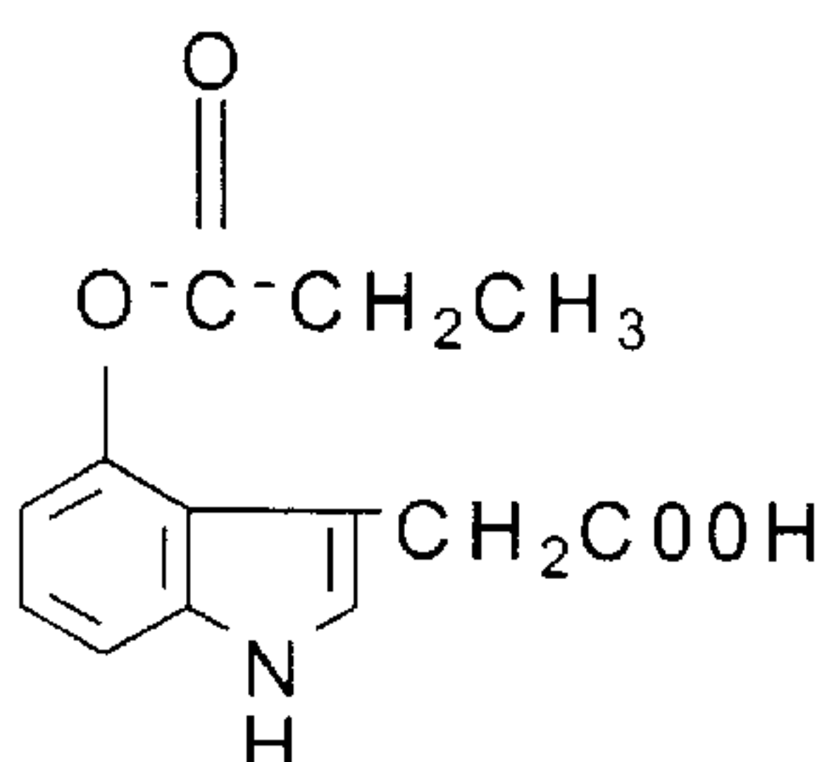
4-propionyloxy-IAA
