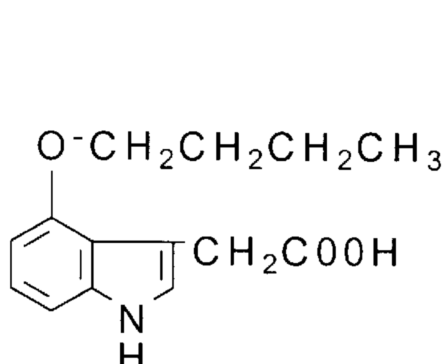
4-butoxy-IAA
