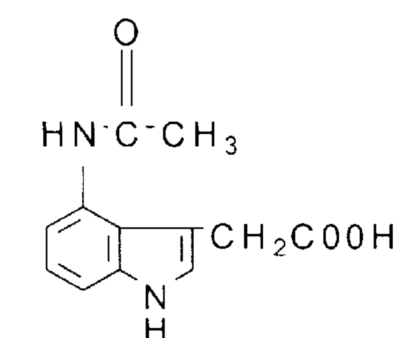
4-acetylamido-IAA
