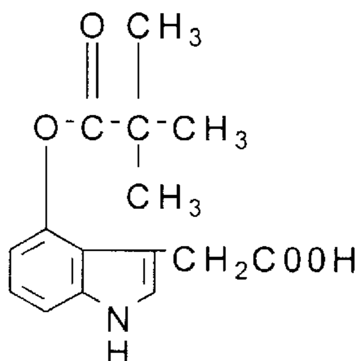
4-tert-valeryloxy-IAA
