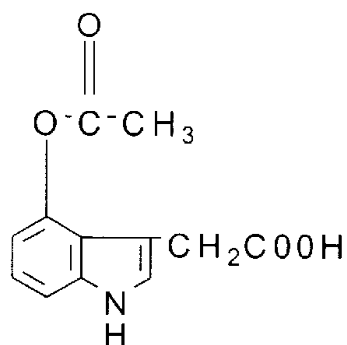
4-acetyloxy-IAA
