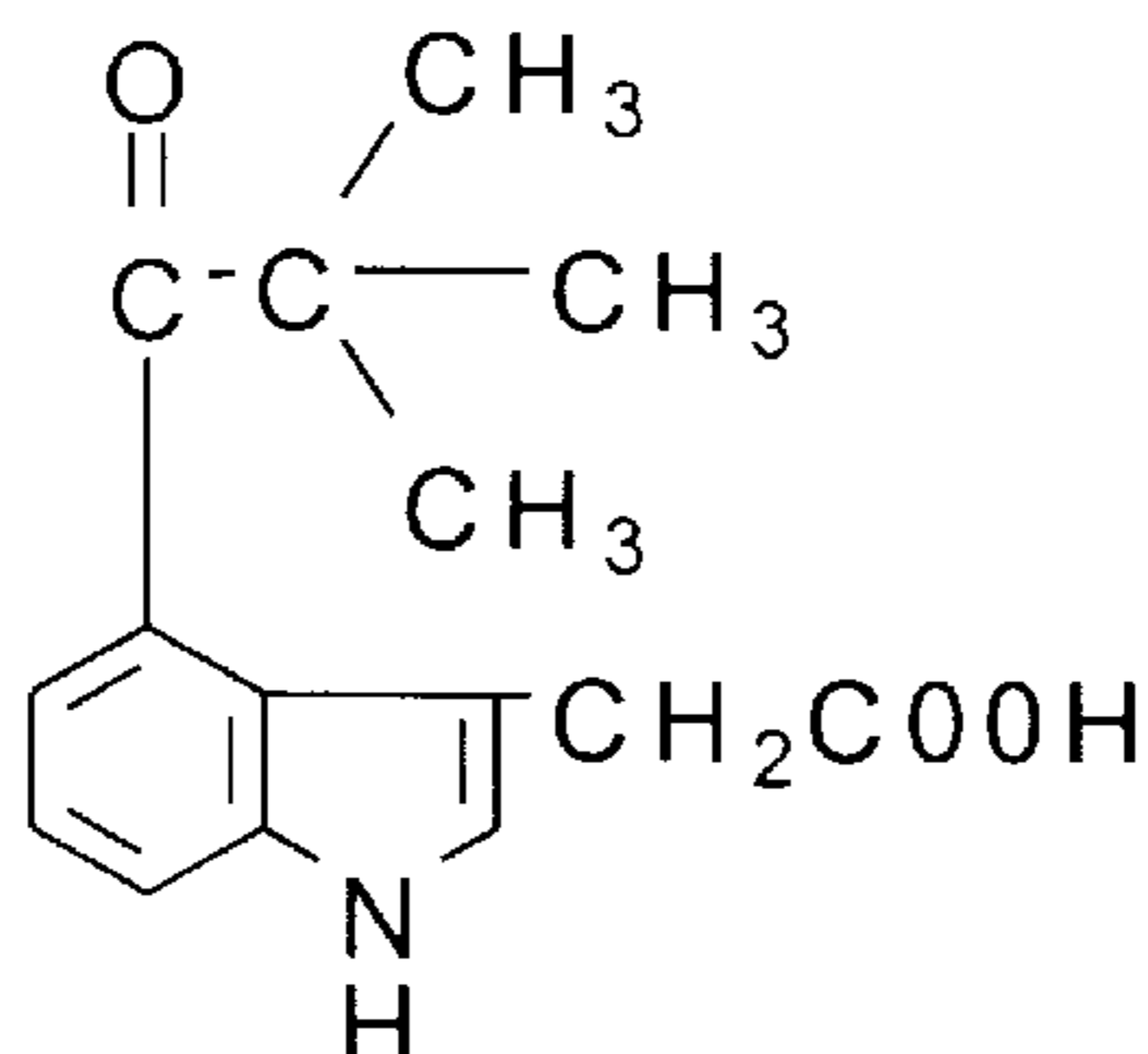
4-tert-valeryl-IAA
