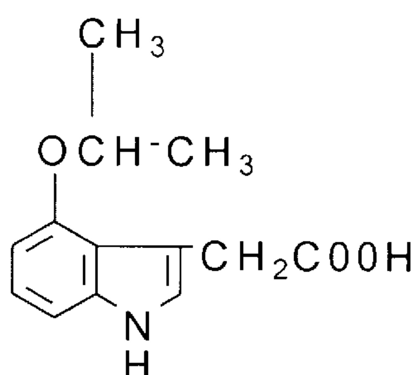
4-isopropoxy-IAA
