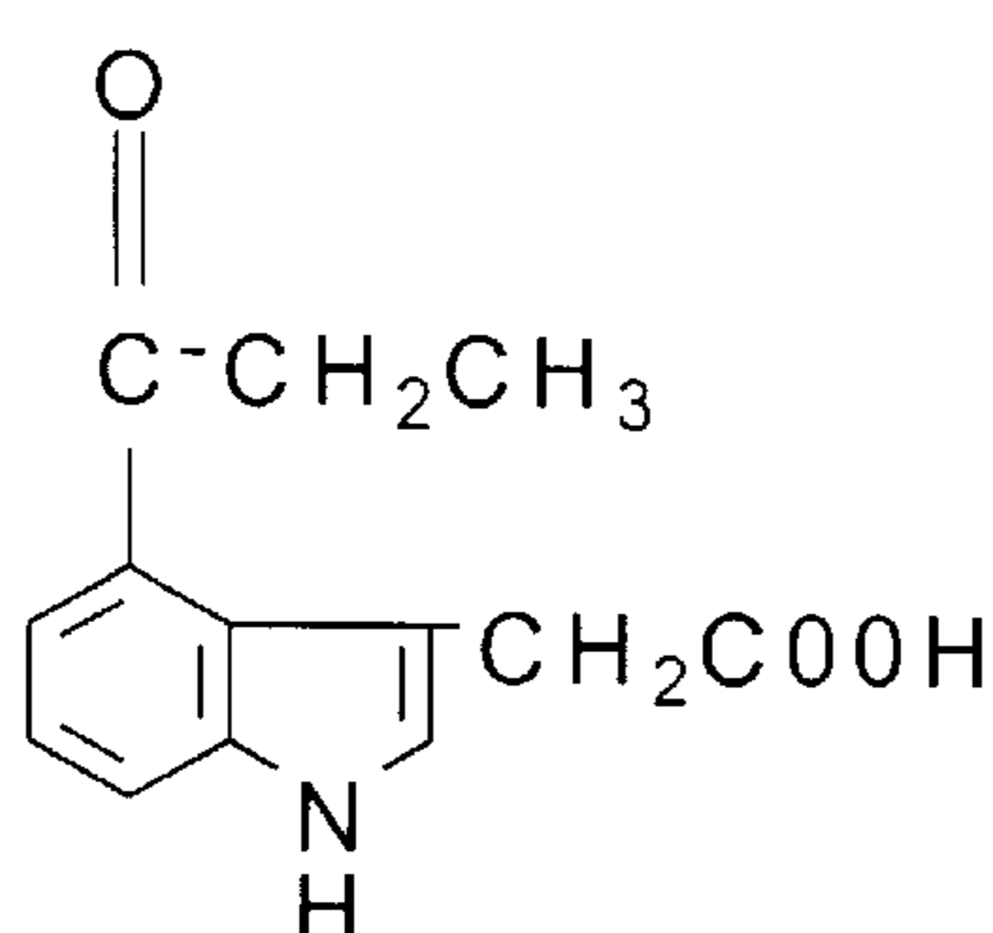
4-propionyl-IAA
