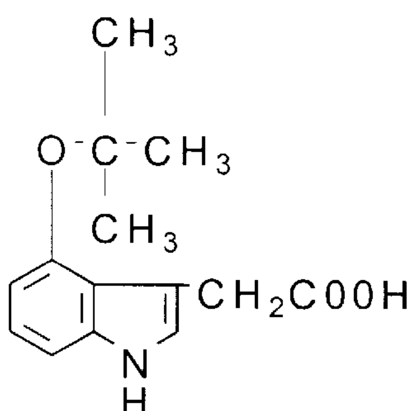
4-tert-butoxy-IAA
