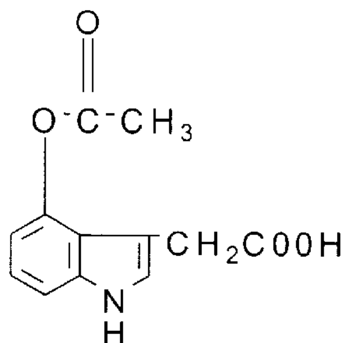
4-acetyloxy-IAA
