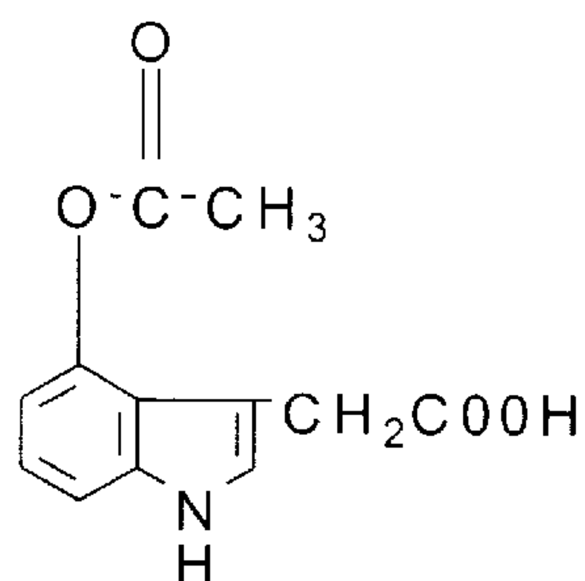
4-acetyloxy-IAA
