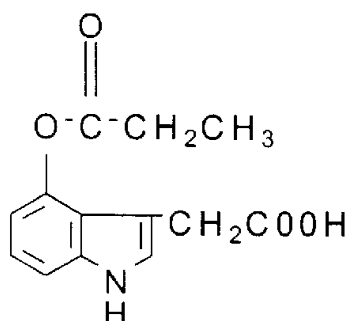
4-propionyloxy-IAA
