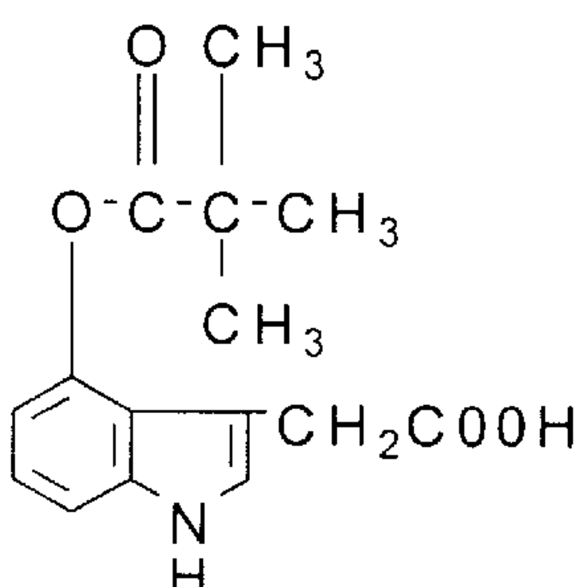
4-tert-valeryloxy-IAA
