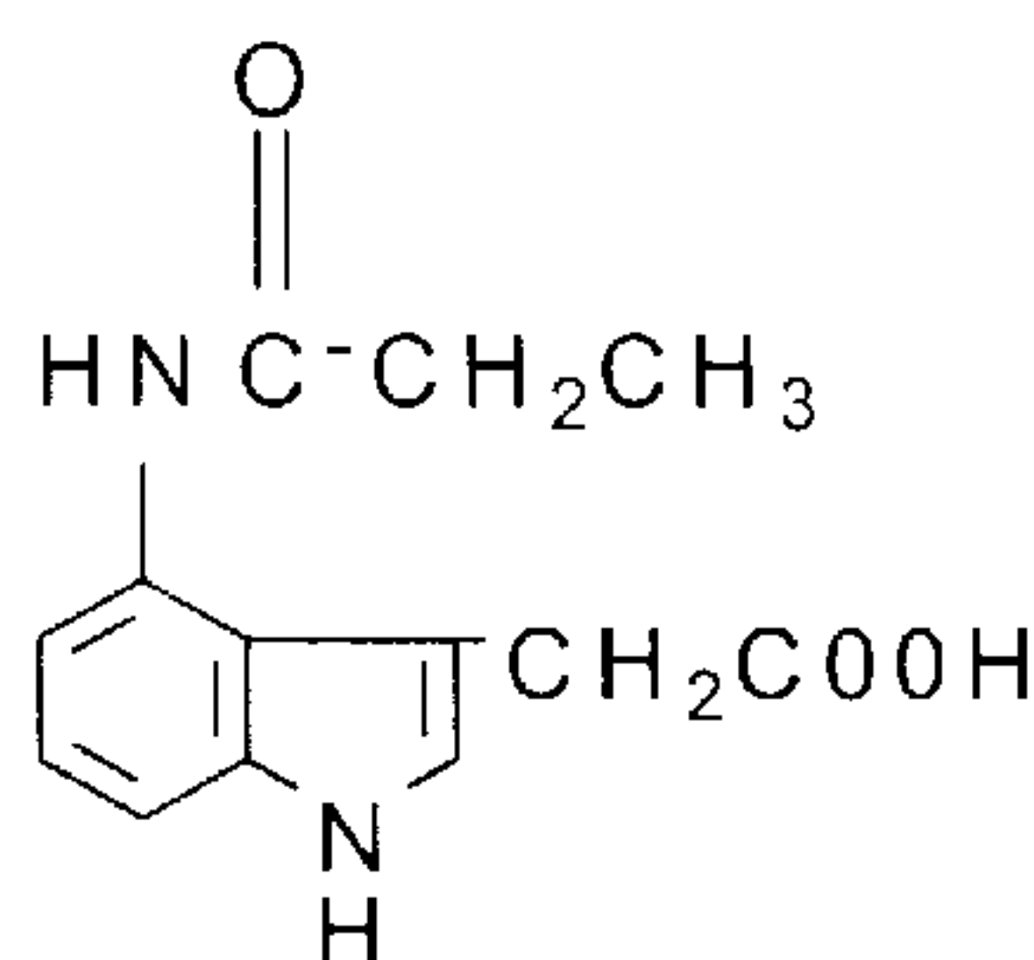
4-propionylamido-IAA
