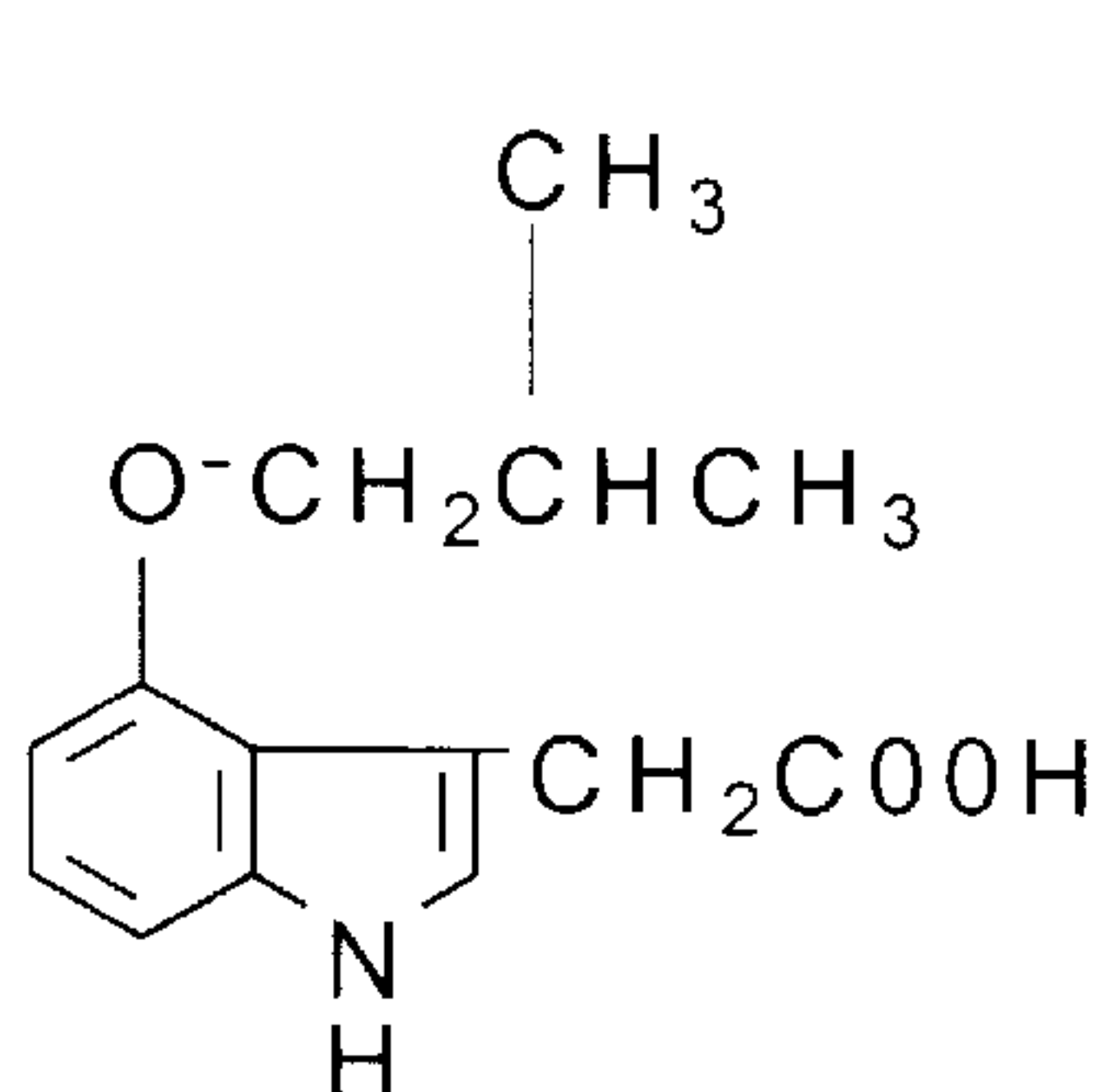
4-isobutoxy-IAA
