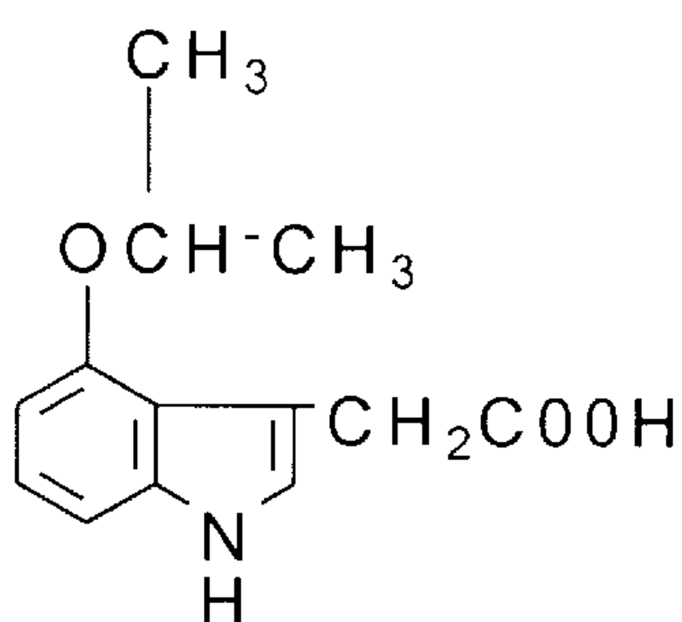
4-isopropoxy-IAA
