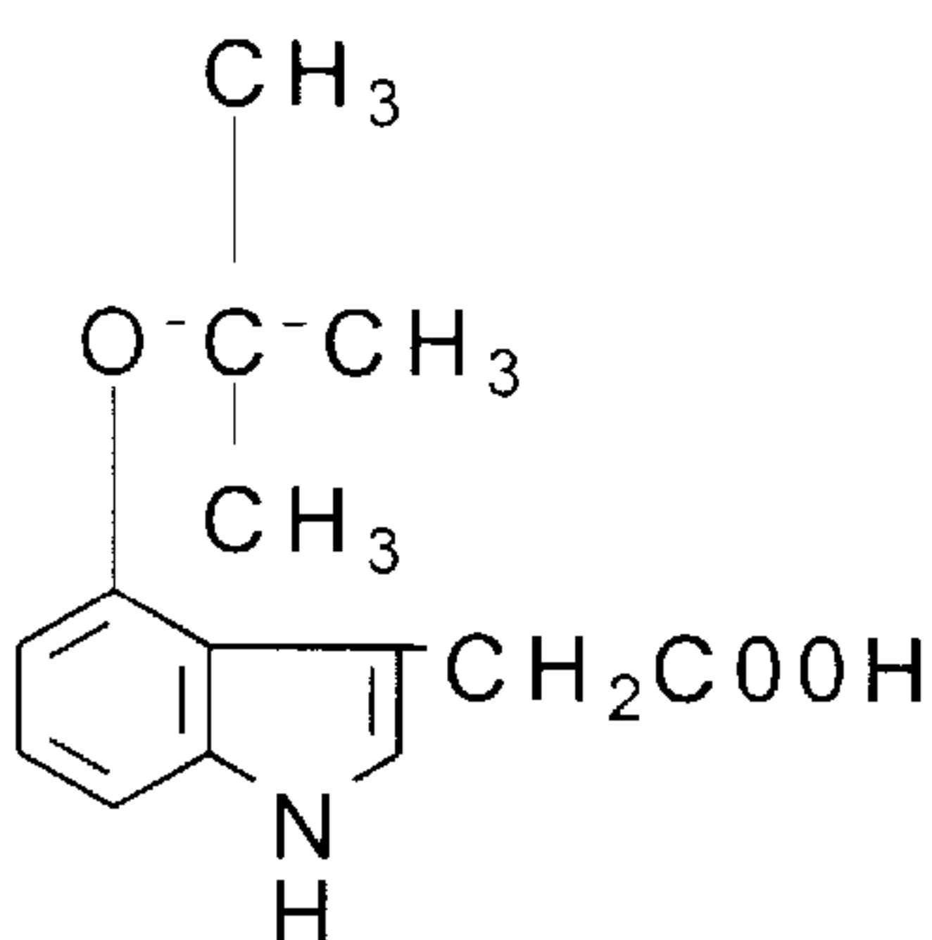
4-tert-butoxy-IAA
