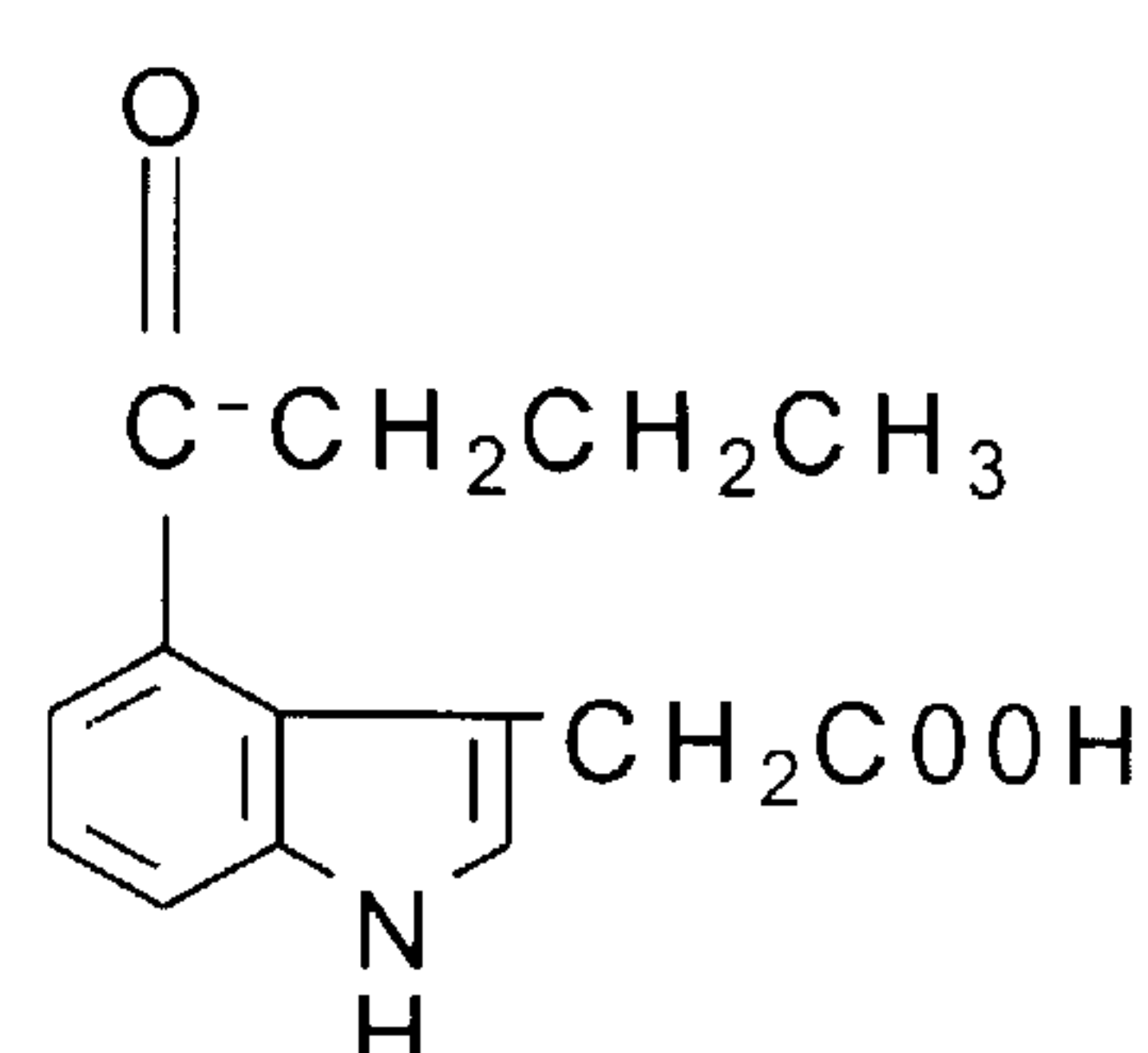
4-butyryl-IAA
