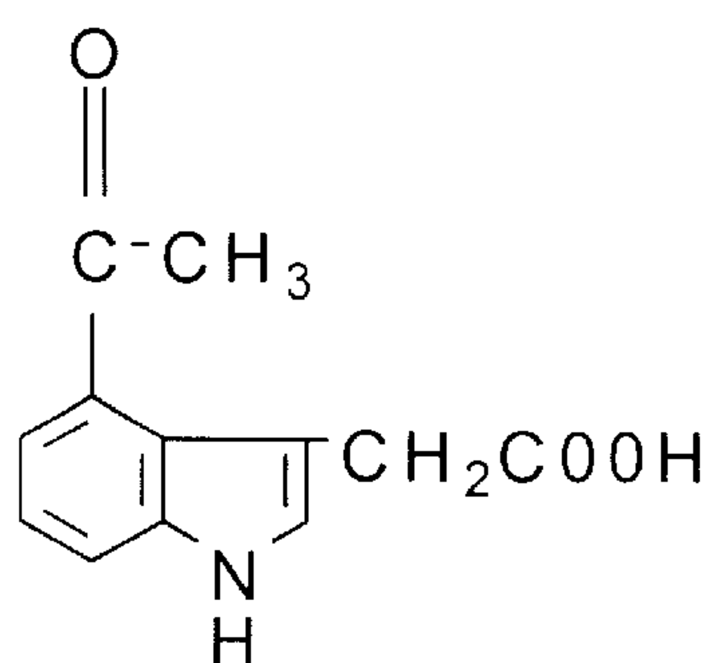
4-acetyl-IAA
