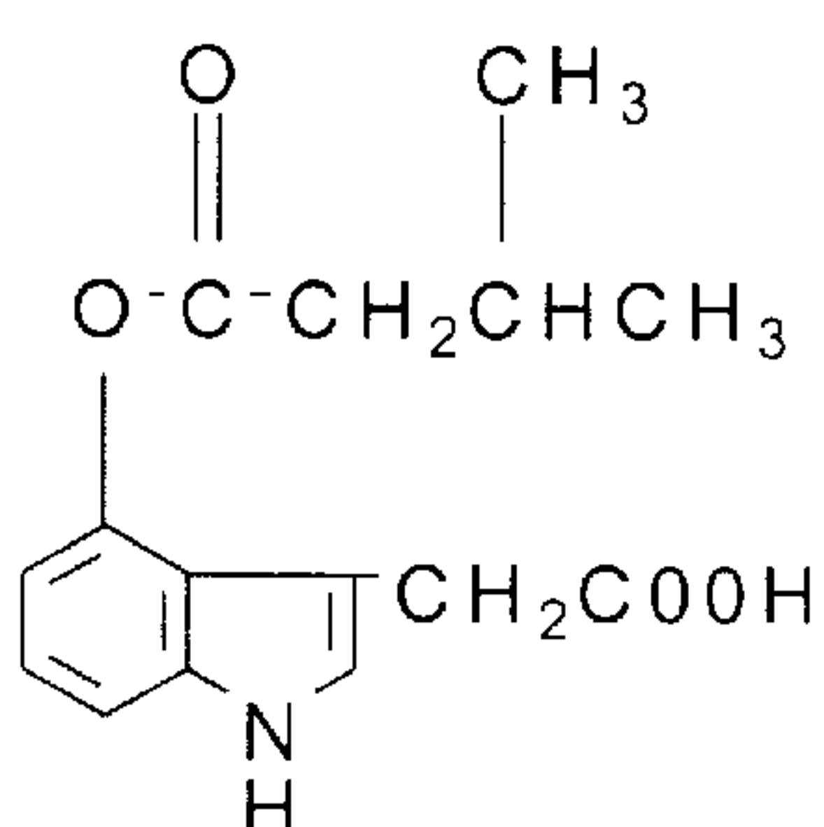
4-isovaleryloxy-IAA
