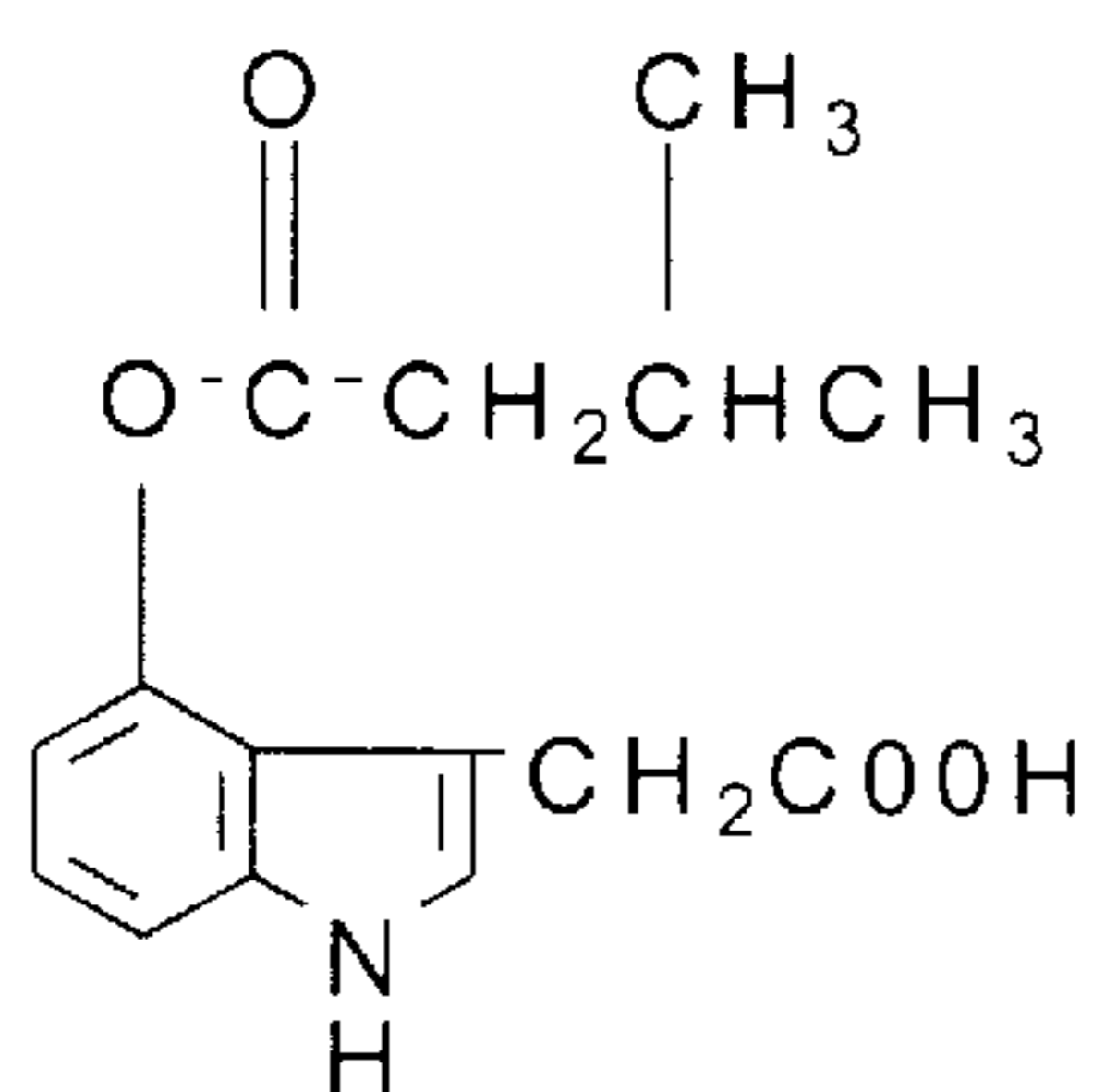
4-isovaleryloxy-IAA
