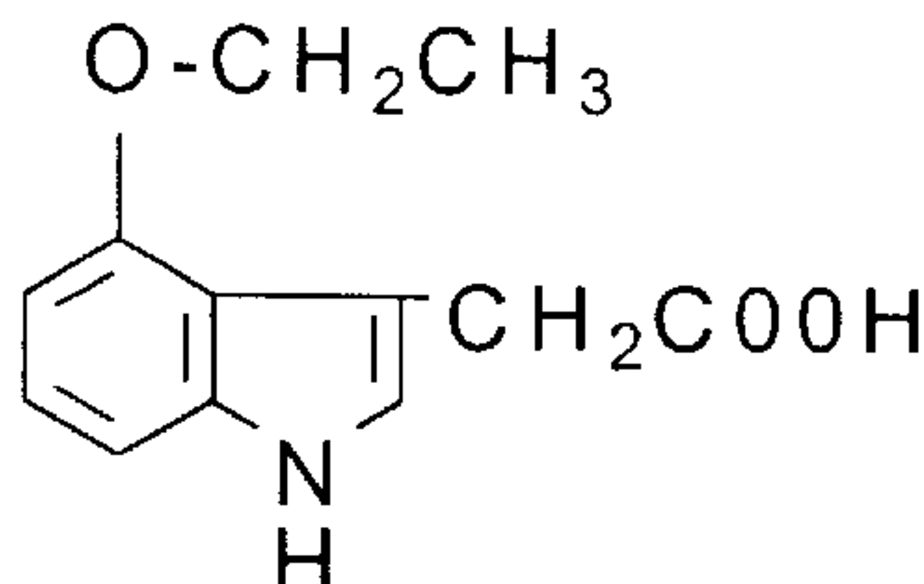
4-ethoxy-IAA
