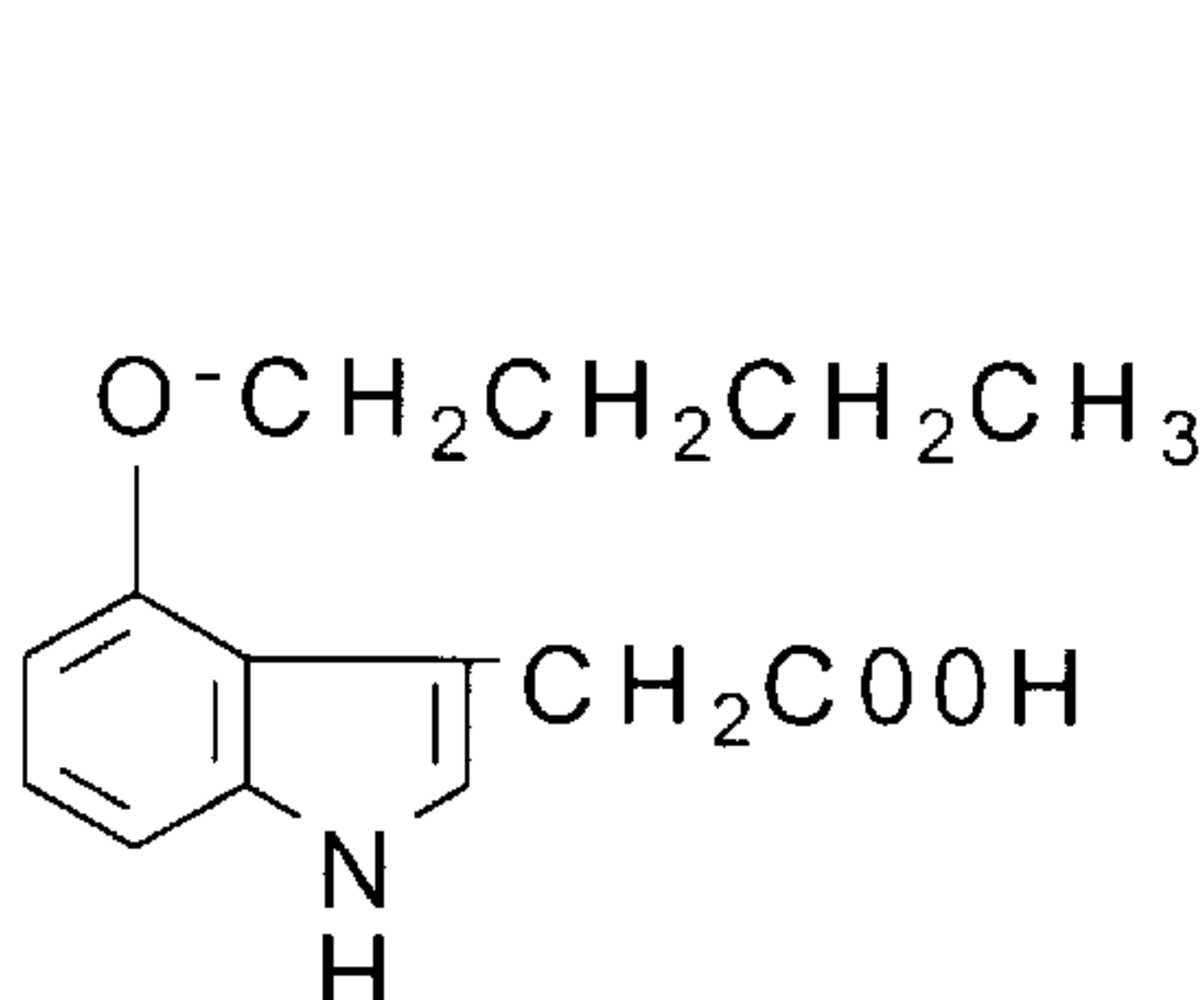
4-butoxy-IAA
