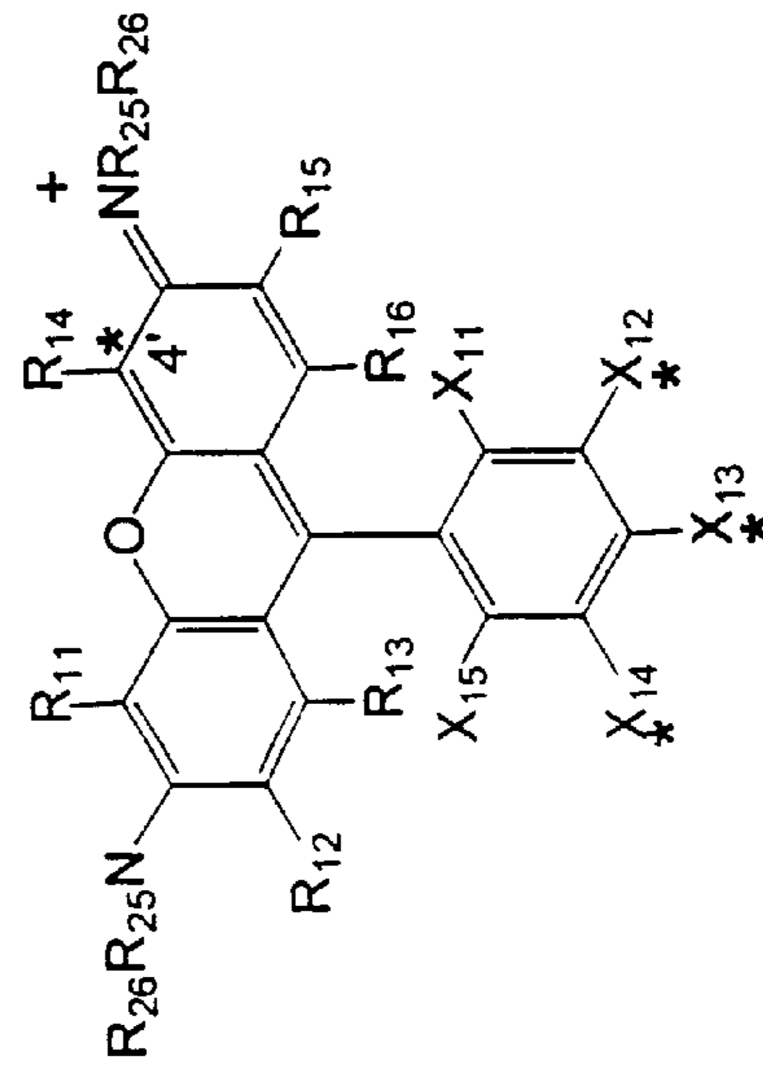
RHODAMINE
