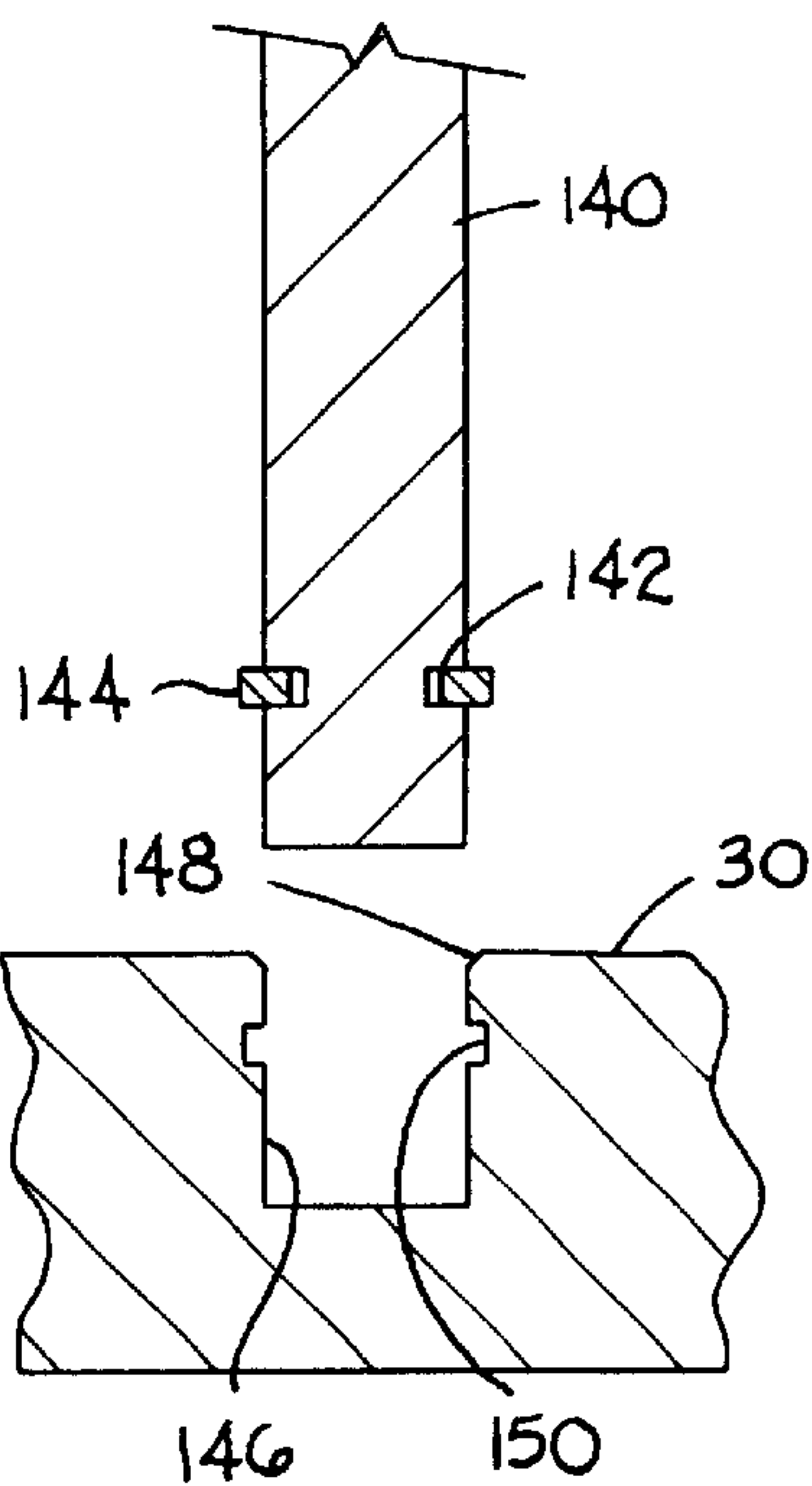
FIG. 6
