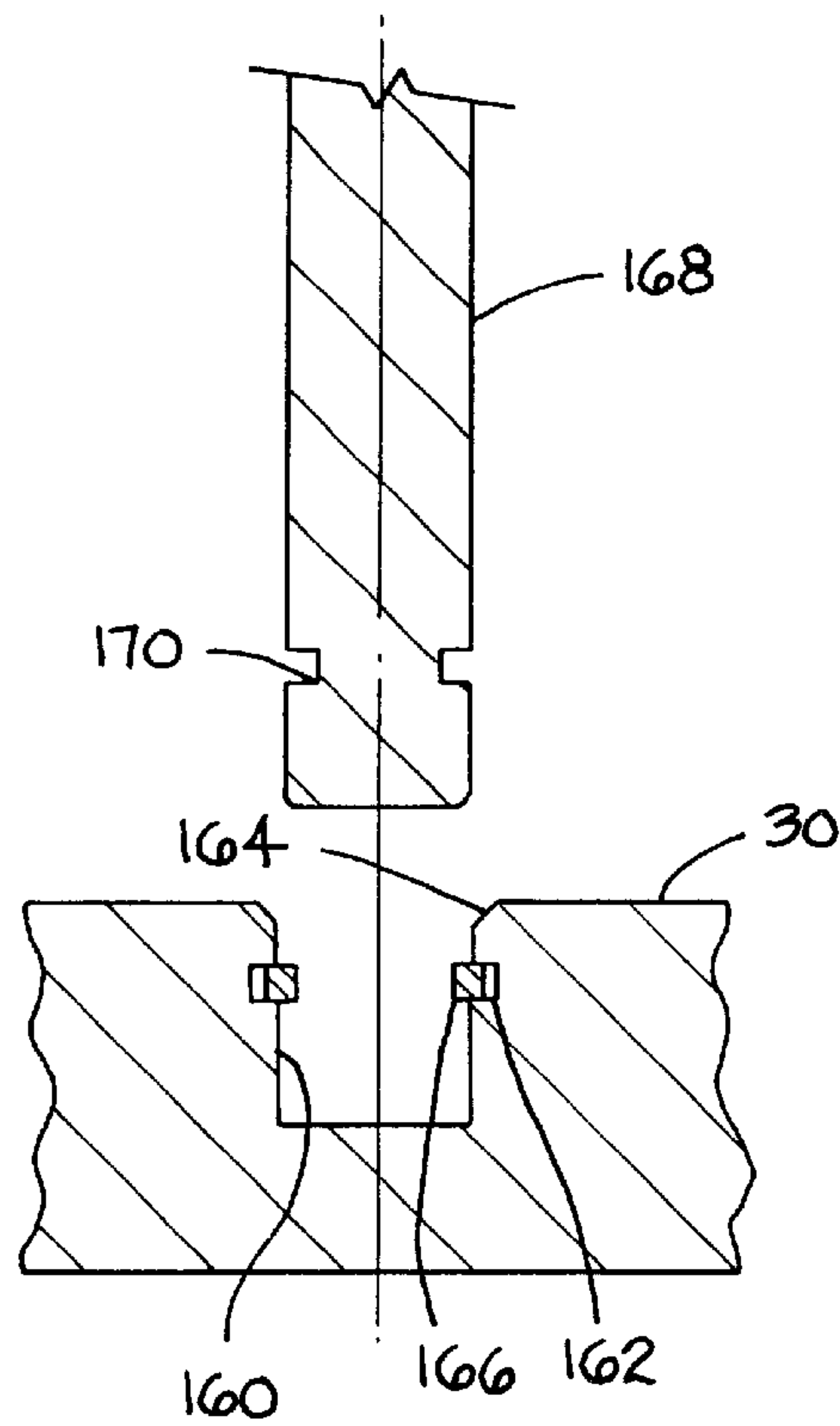
FIG. 8
