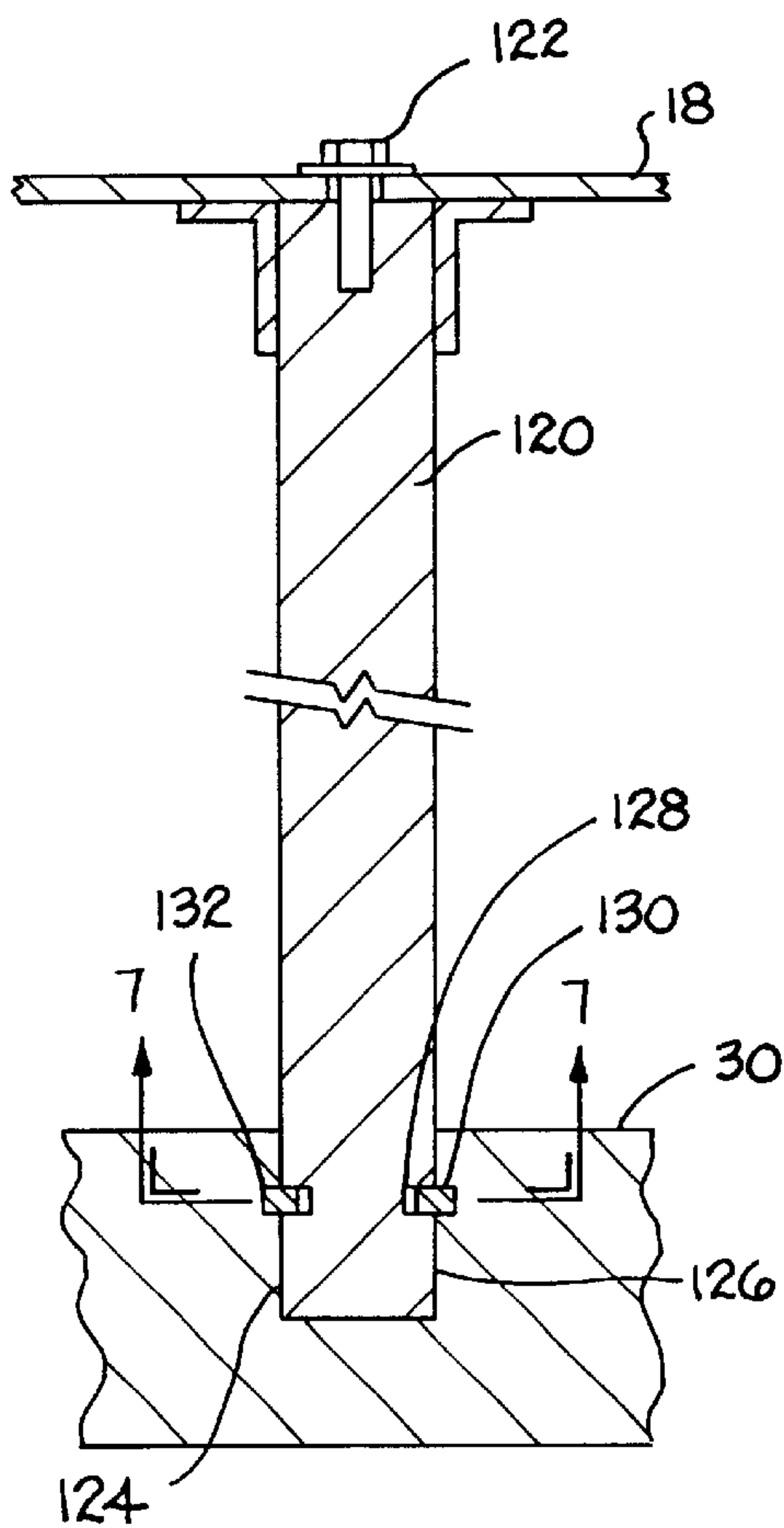
FIG. 5
