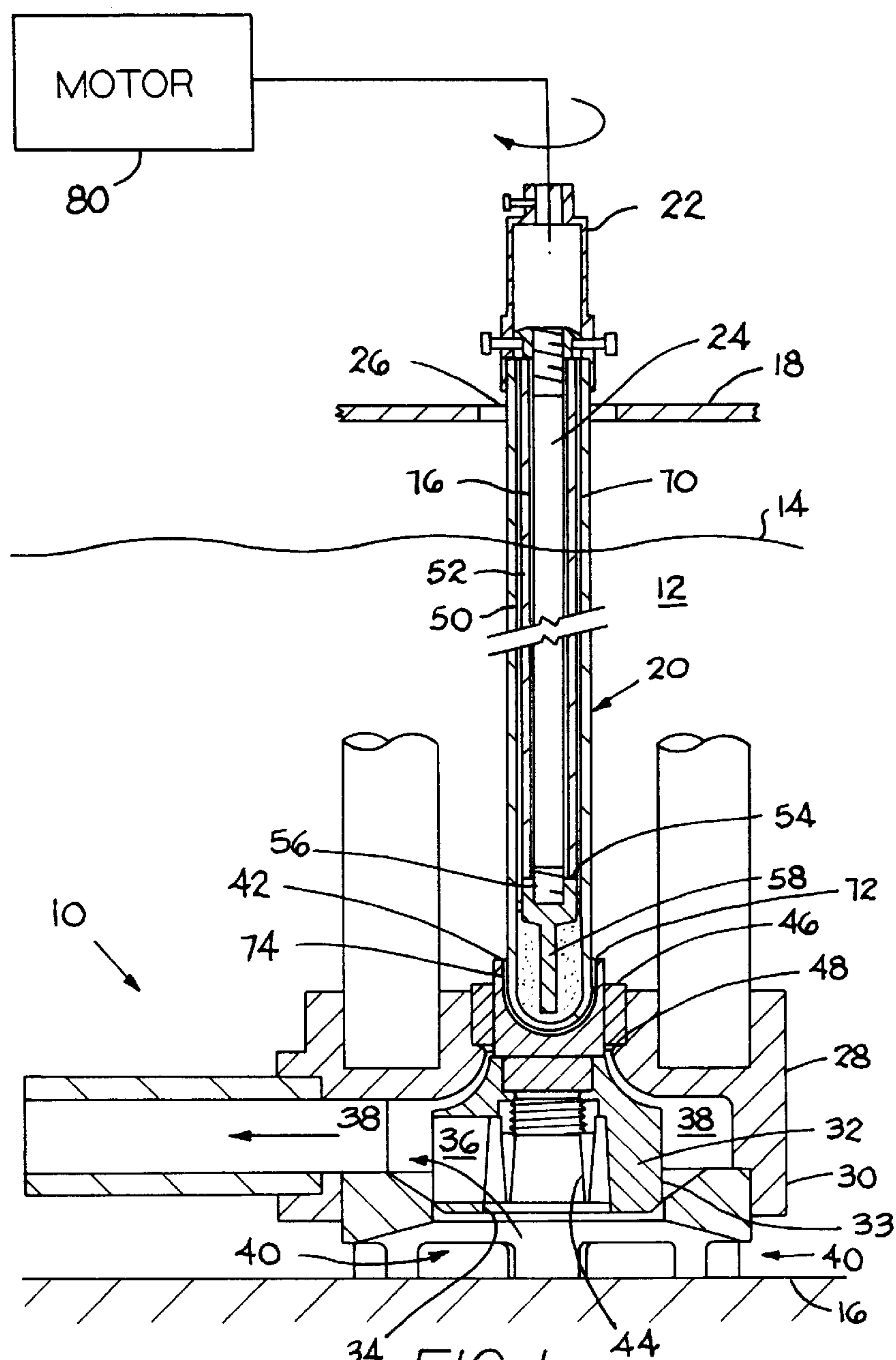
FIG. 1
