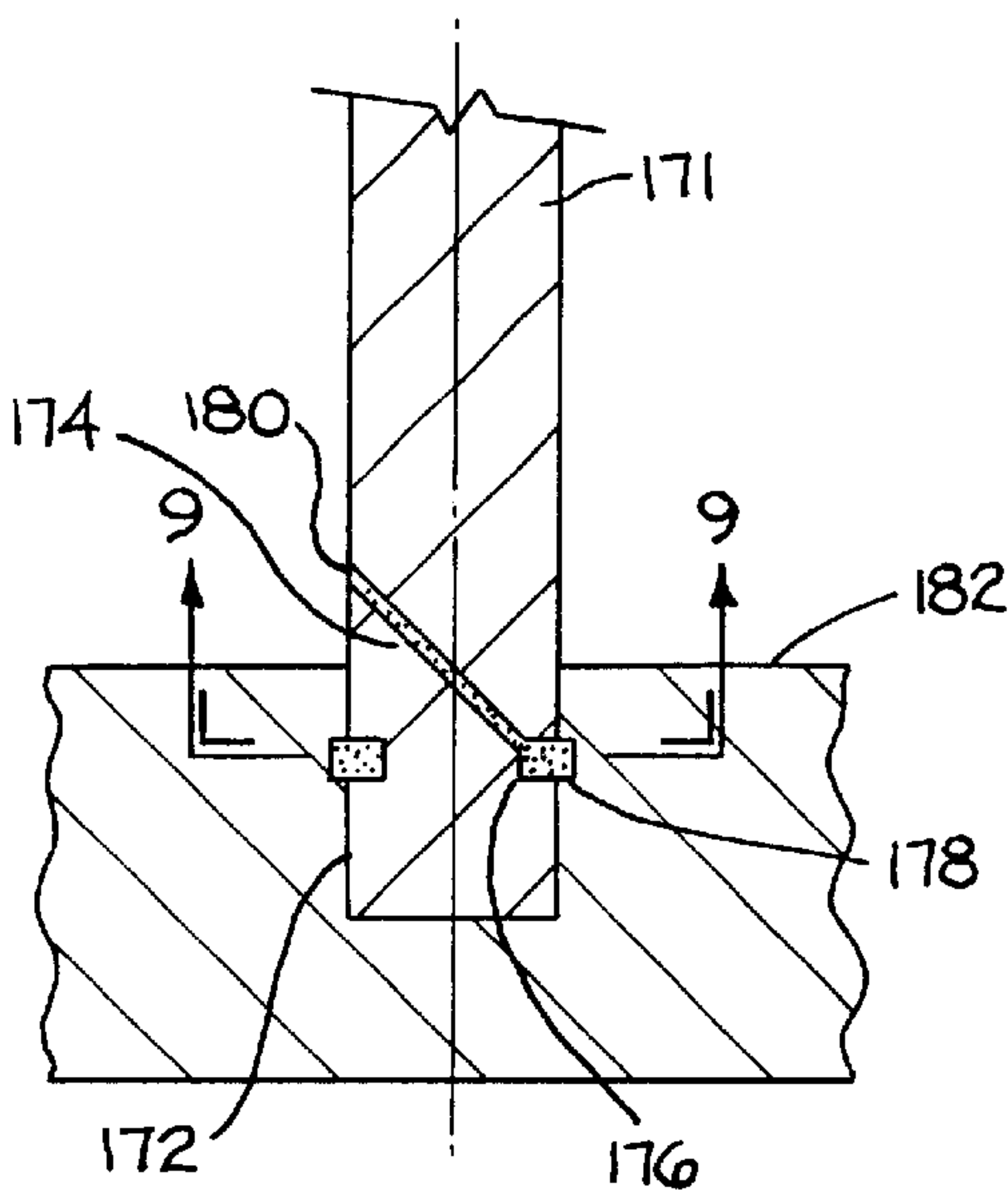
FIG. 8A
