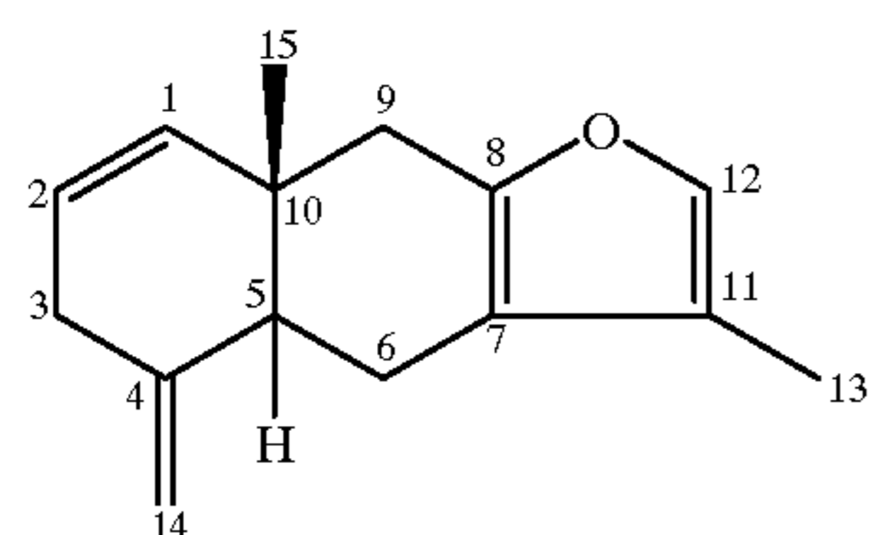
Lindestrone (Furanogermaorans type)
