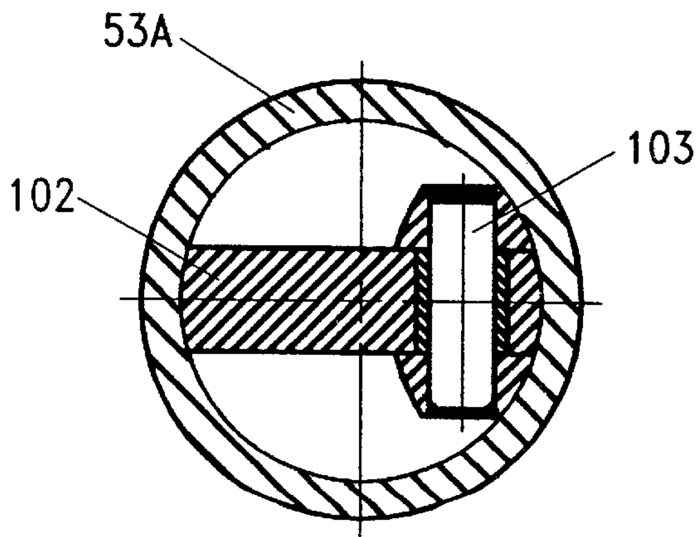
SECTION D-D
