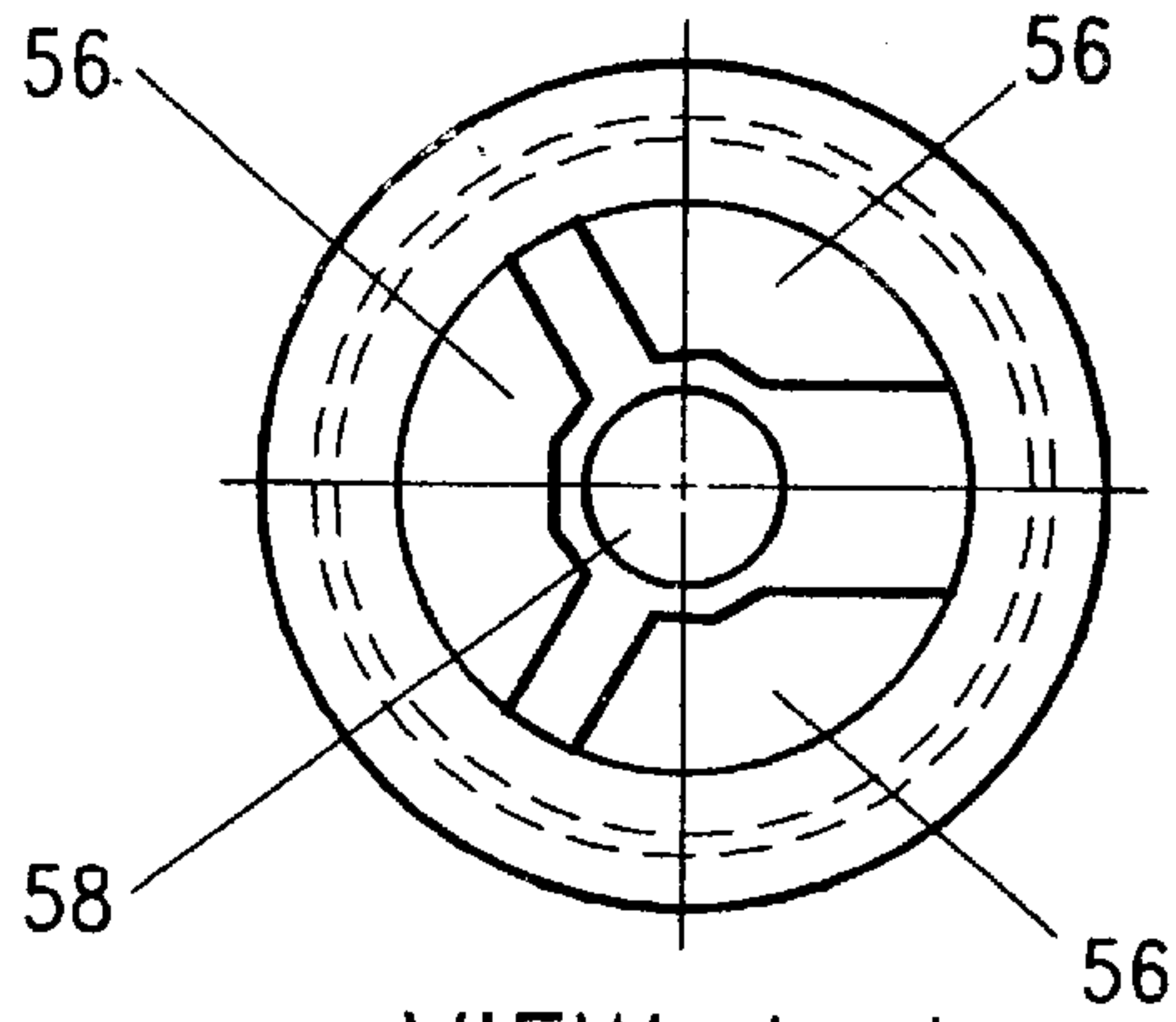
VIEW A-A
