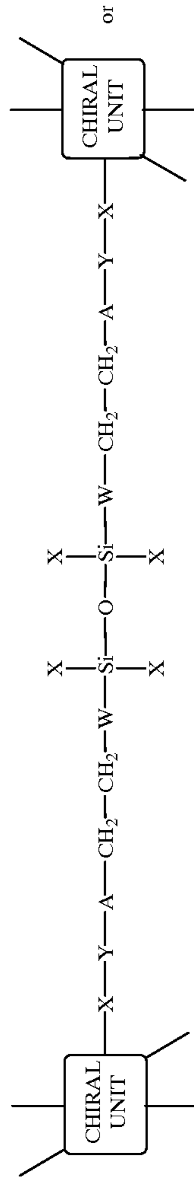
(IXc)
