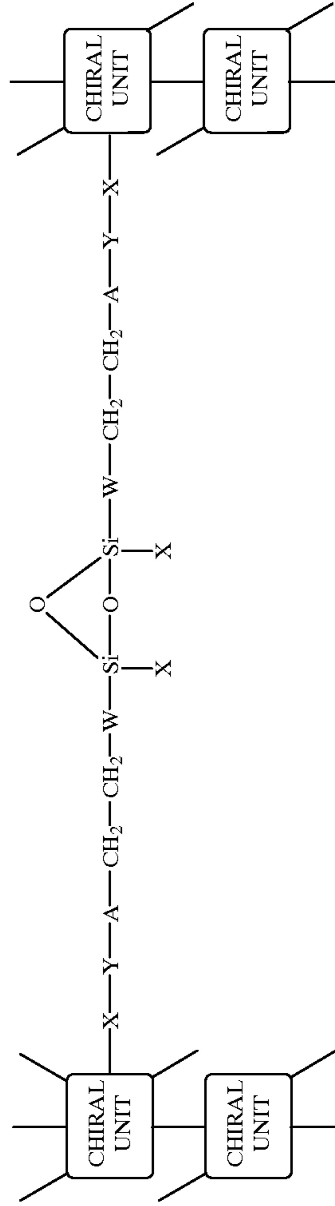
(IXd)
