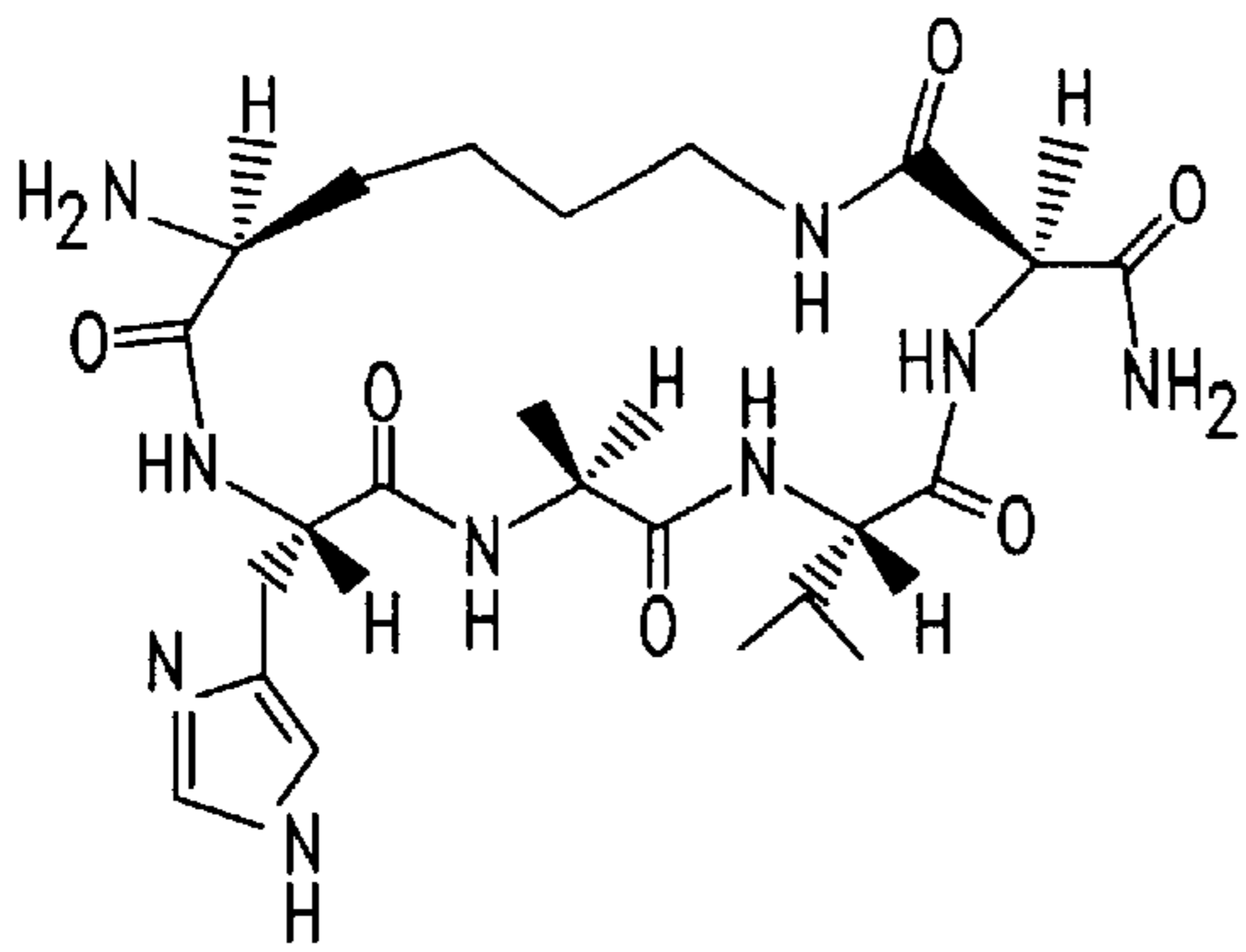
H-KHAVD-NH 2
