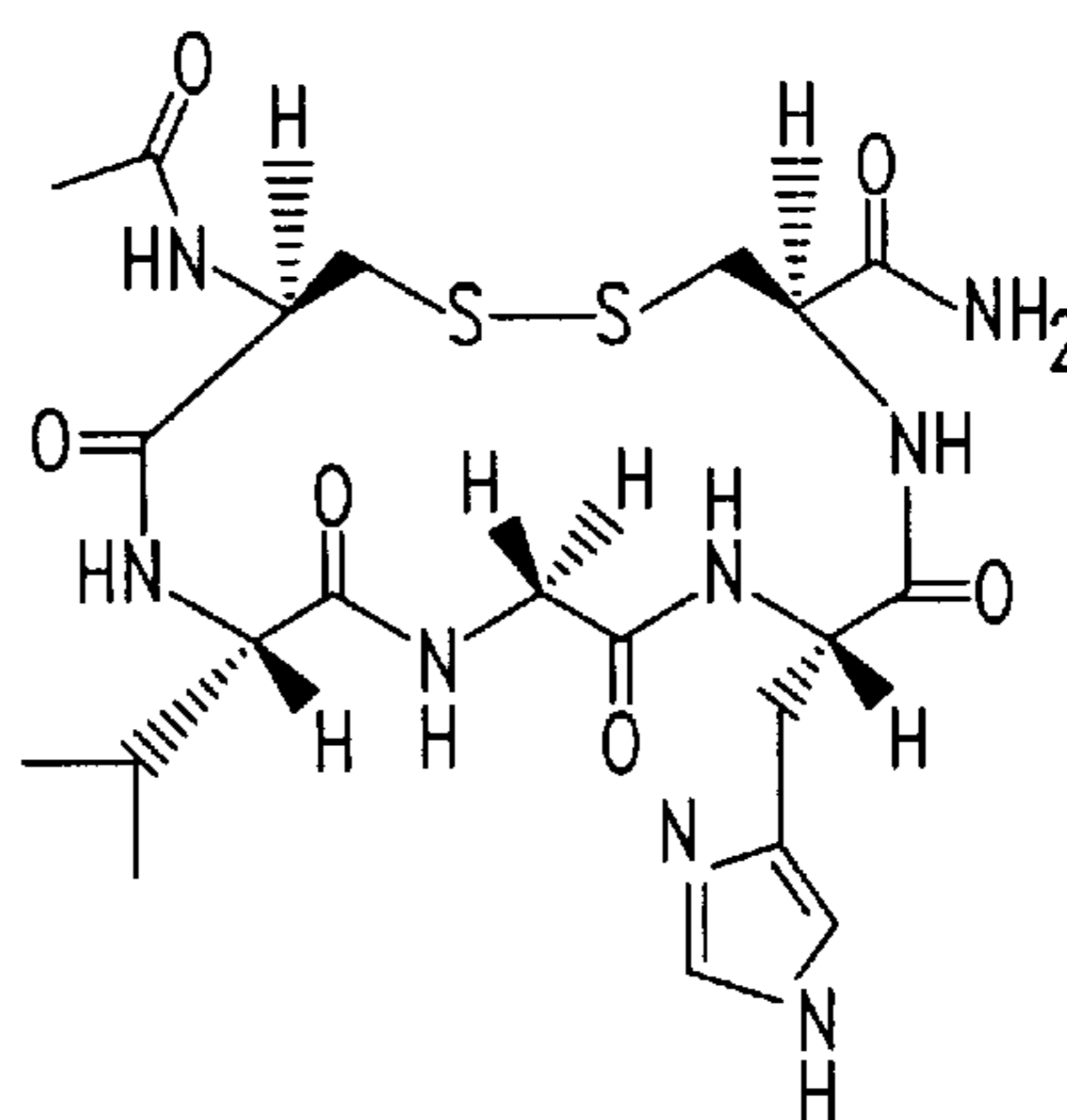
N-Ac-CVGHC-NH 2
