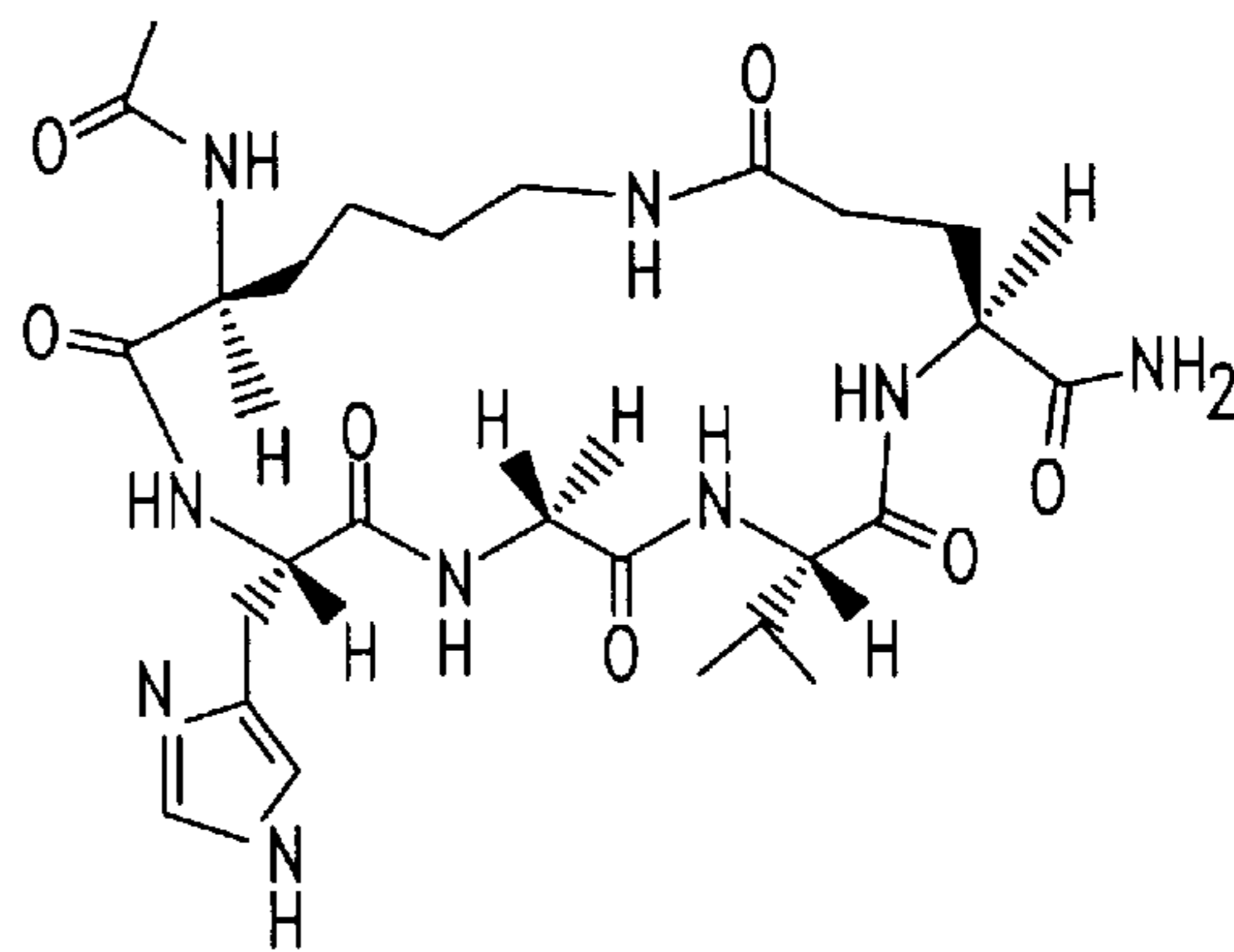
N-Ac-KHGVK-NH 2
