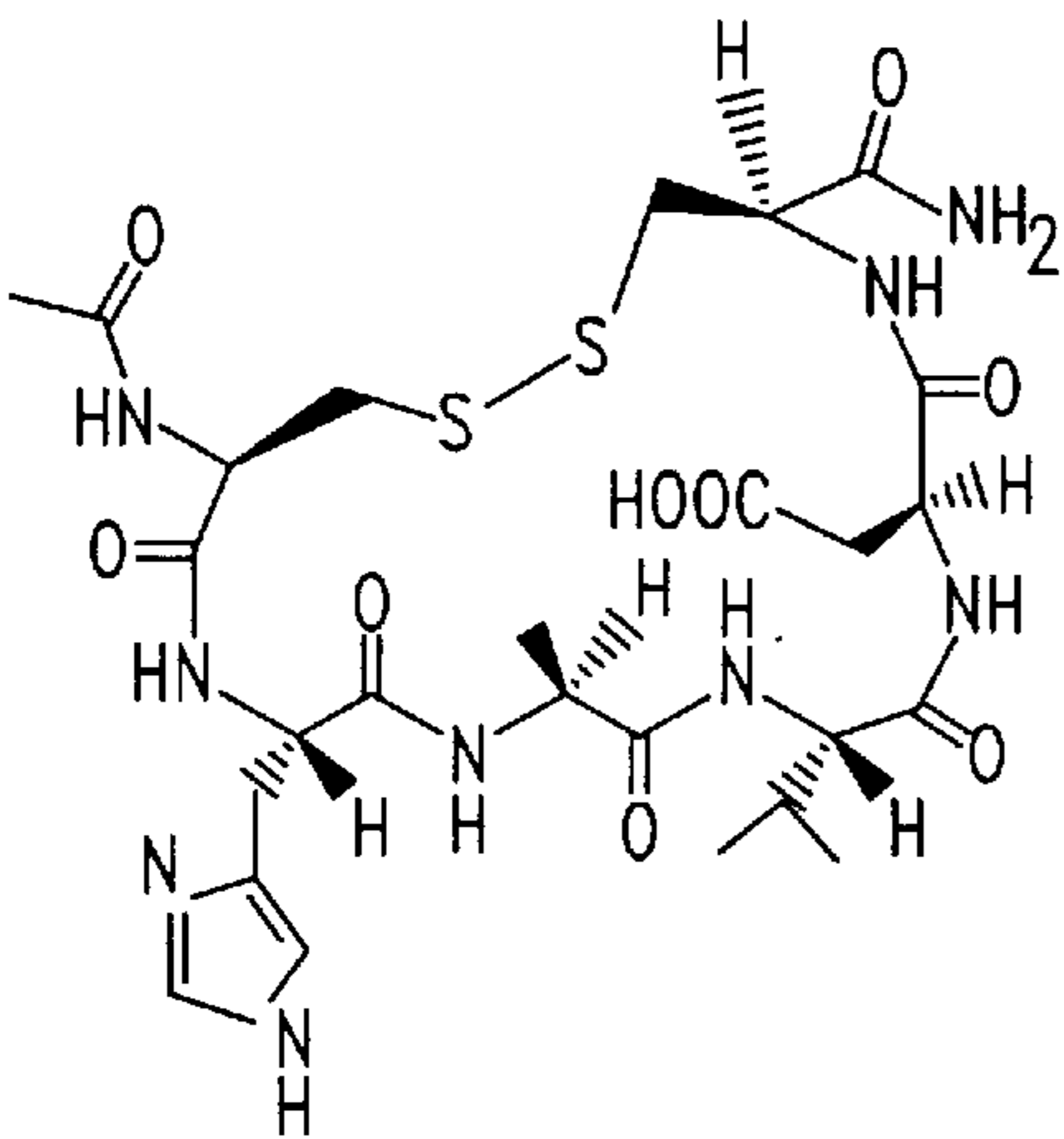
N-Ac-CHAVDC-NH 2
