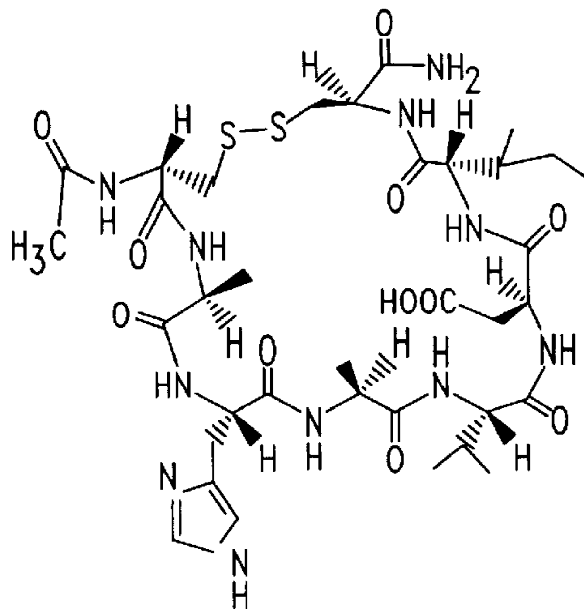
N-Ac-CAHAVDIC-NH 2
