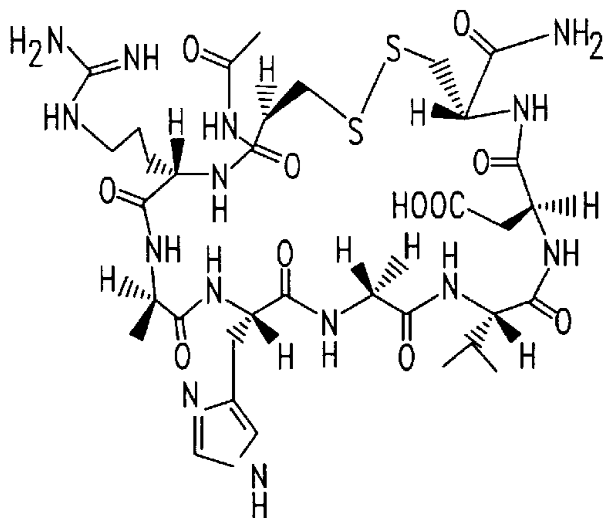
N-Ac-CRAHAVDC-NH 2
