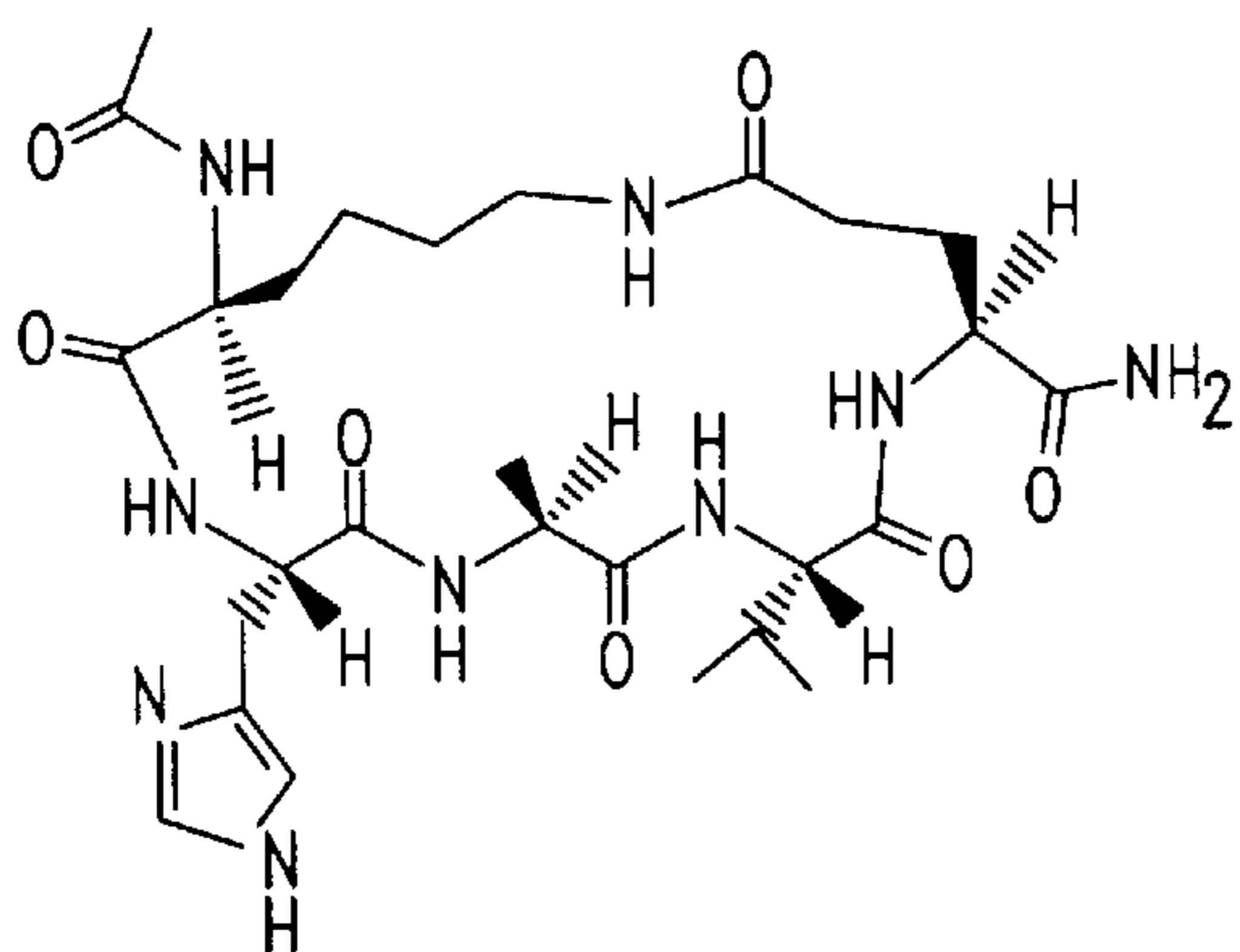
N-Ac-KHAVE-NH 2
