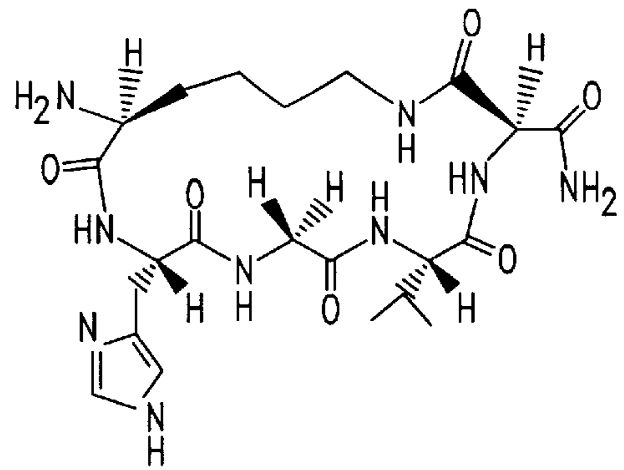
H-KHGVND-NH 2
