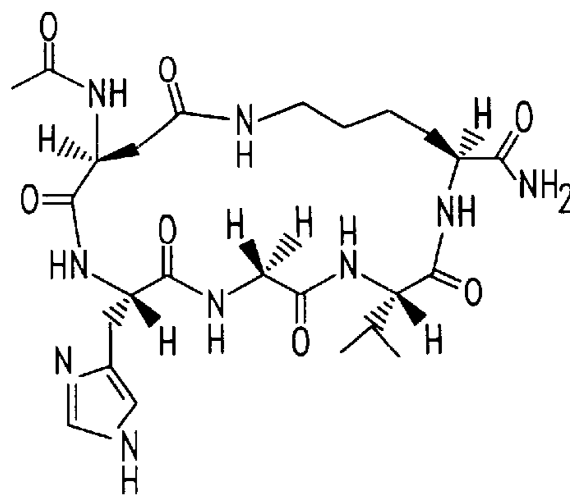
N-Ac-DHGVK-NH 2
