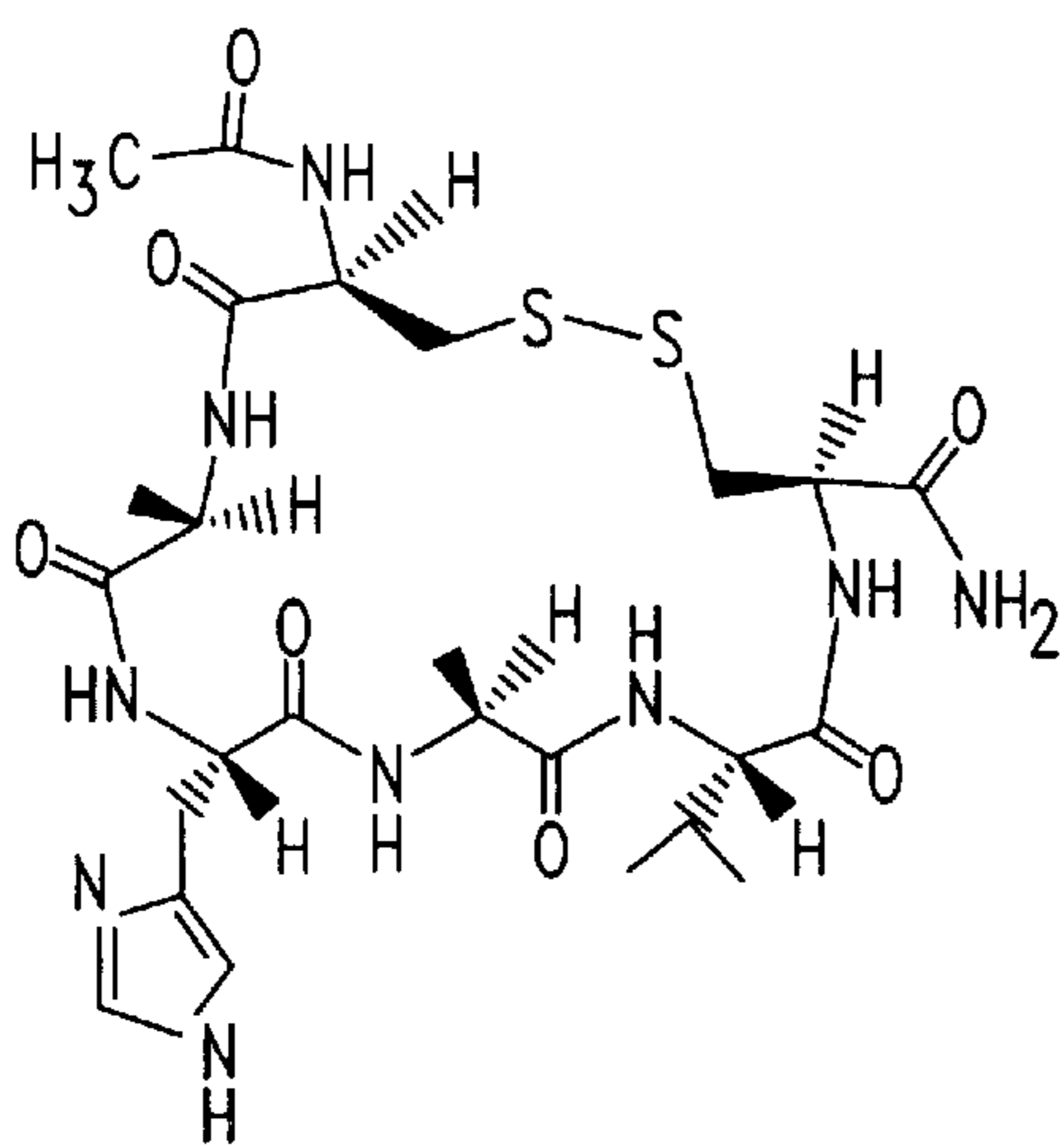
N-Ac-CAHAVC-NH 2
