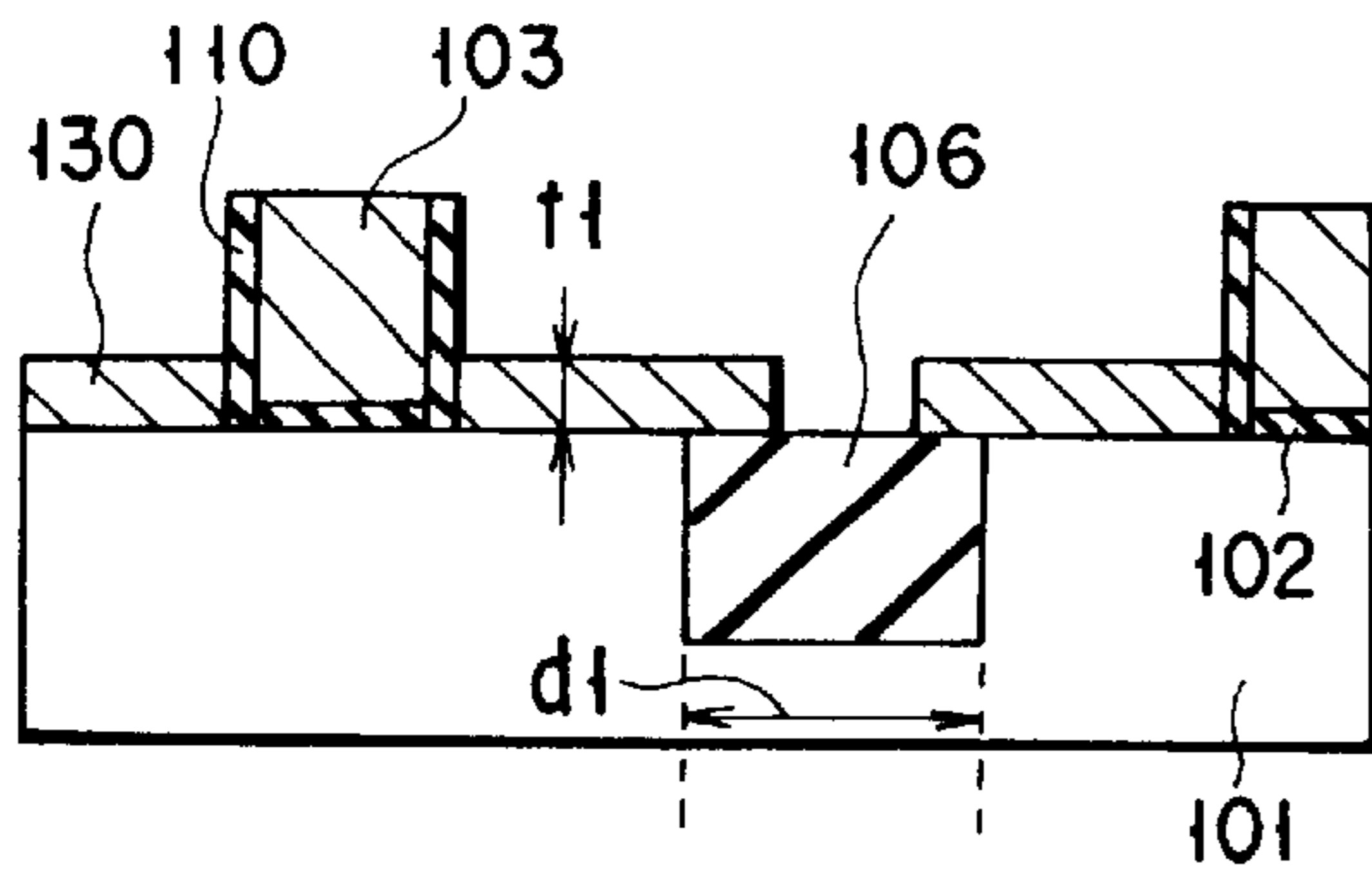
FIG. 20A PRIOR ART
