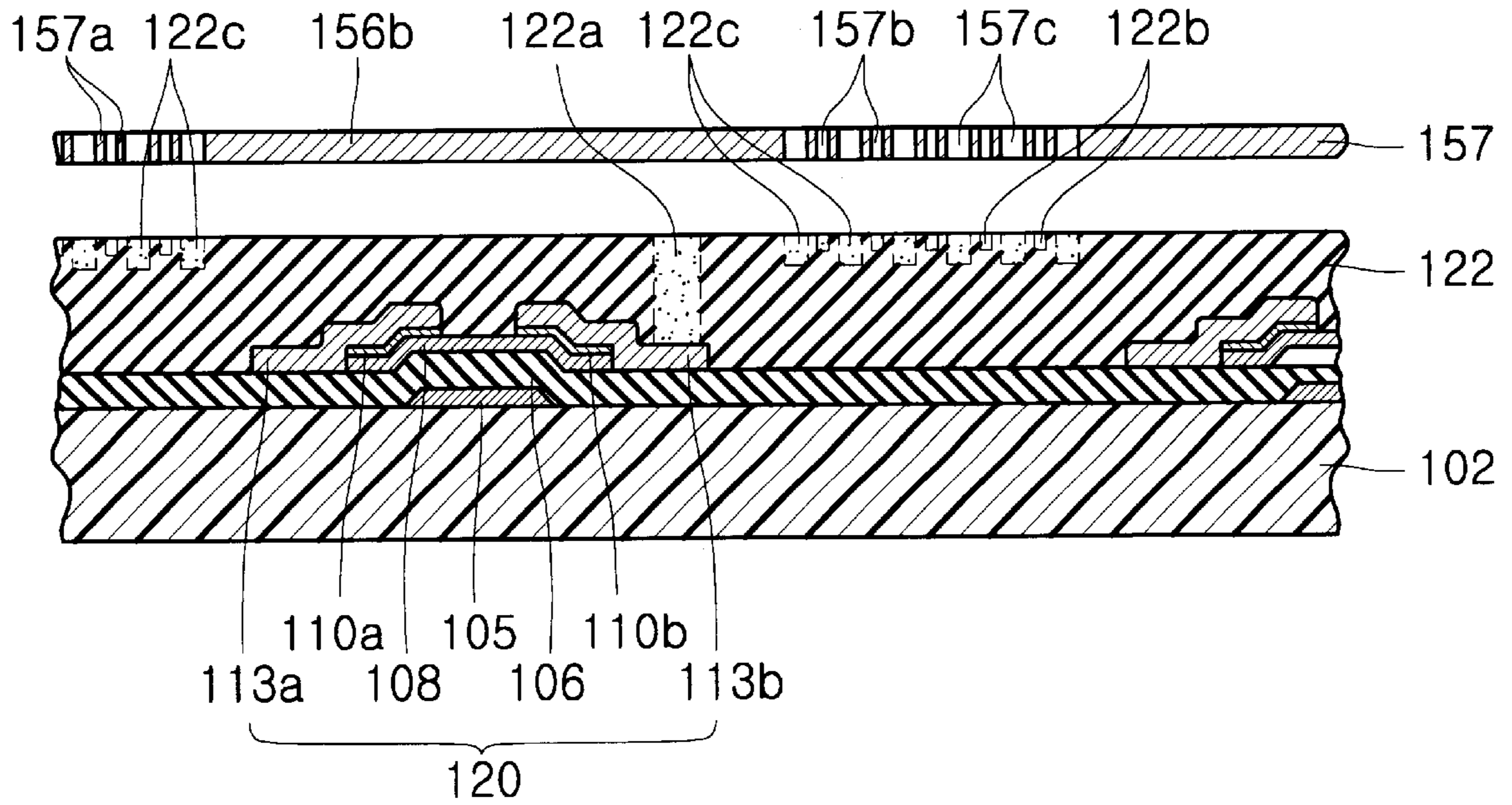
FIG. 6C
