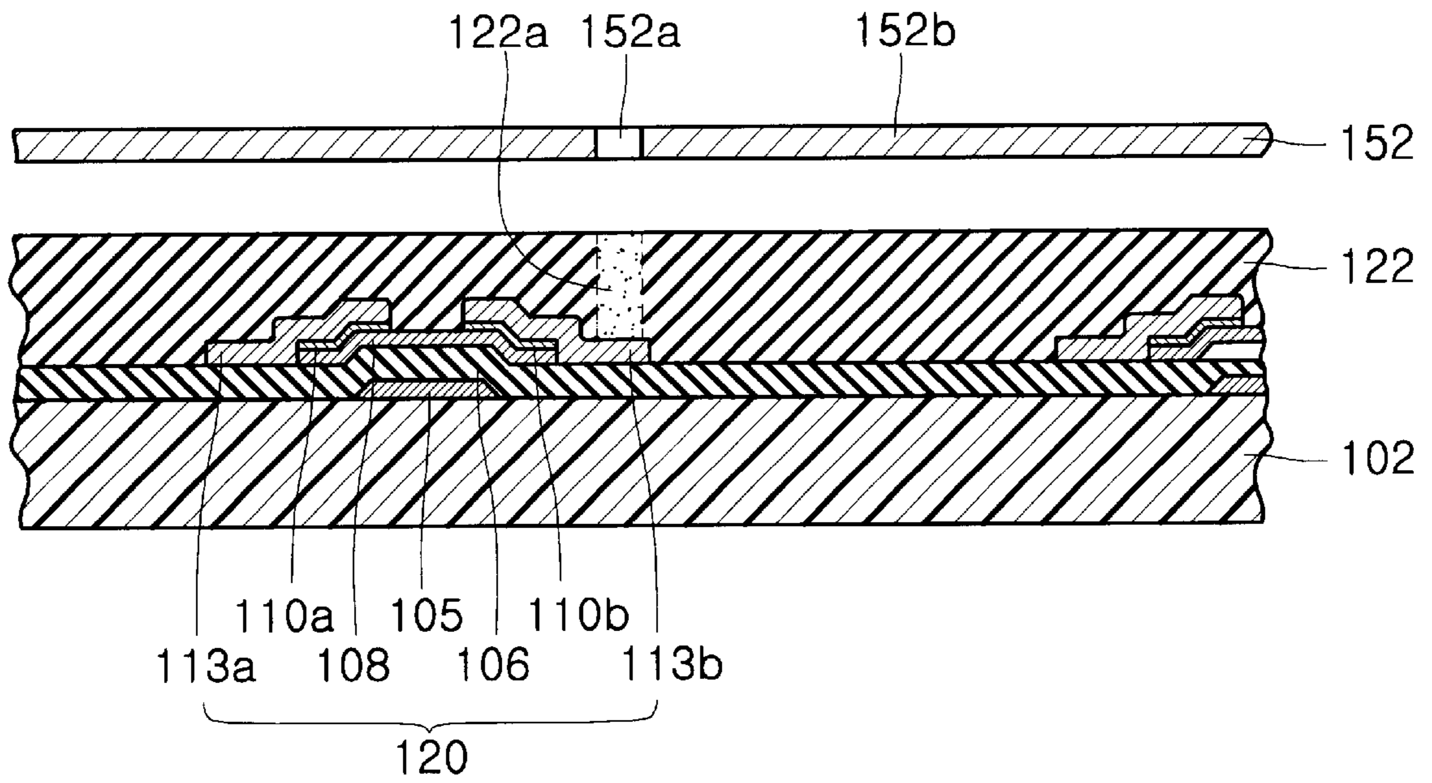
FIG. 6B
