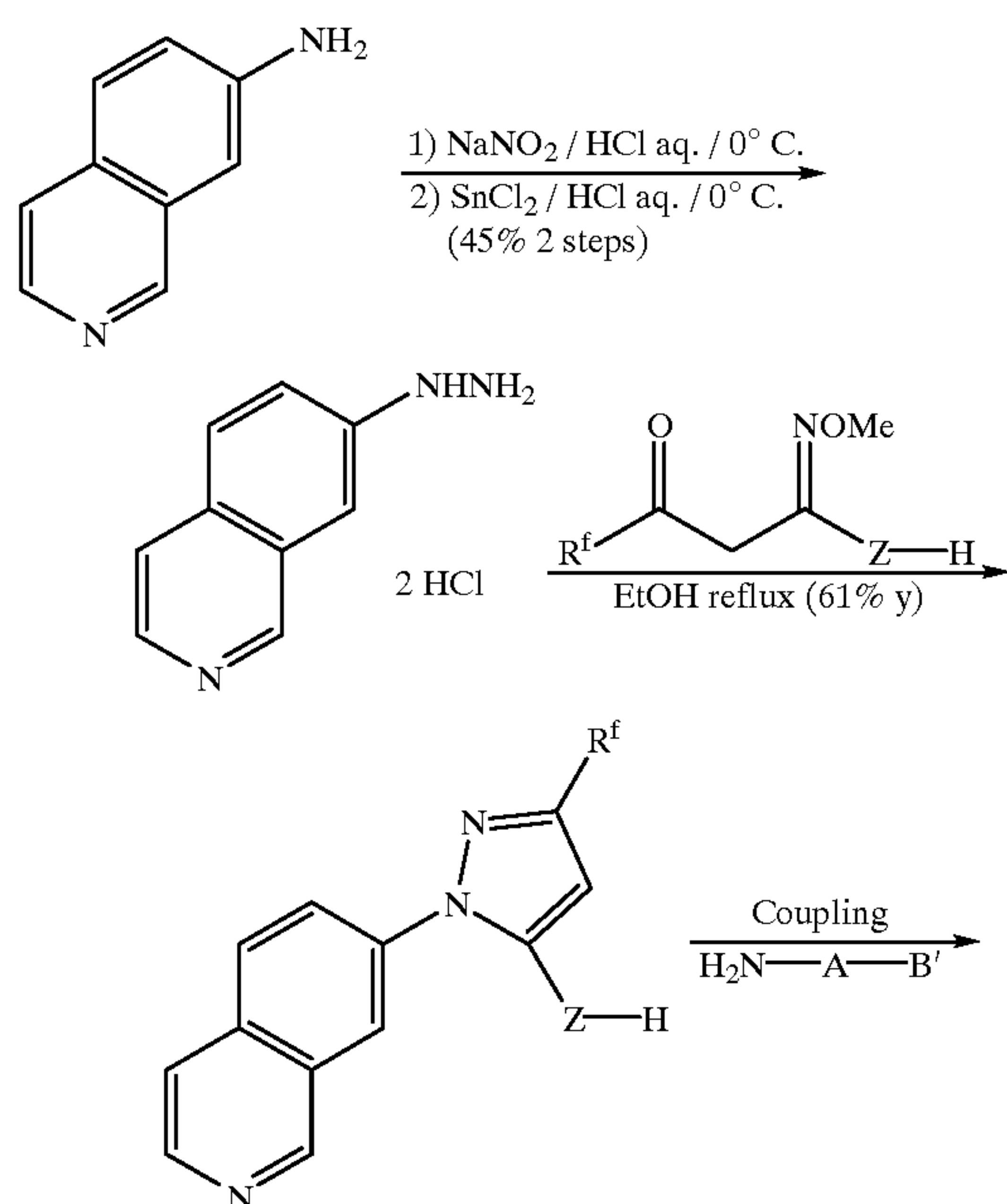
SCHEME 2a
