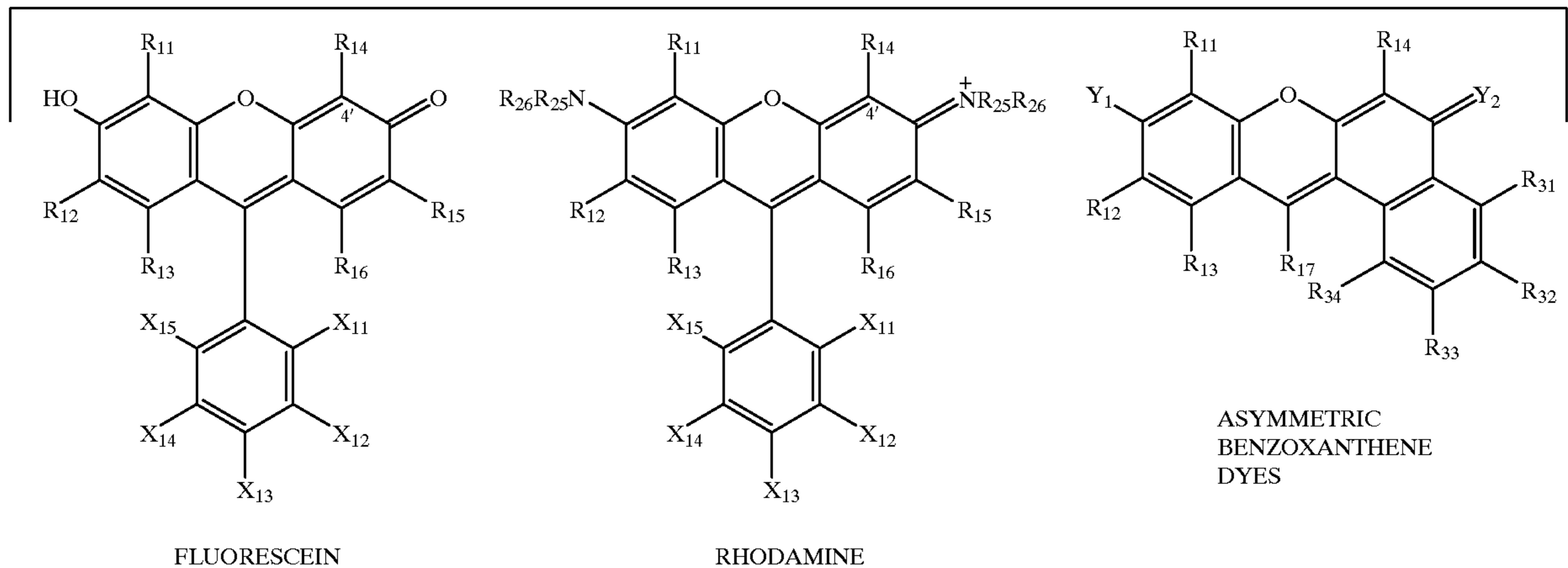
XANTHENE
