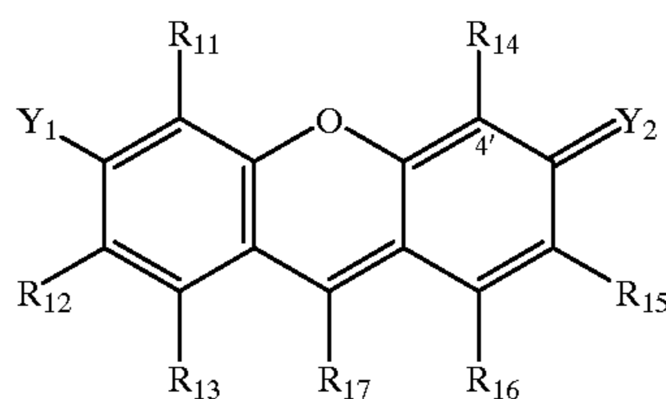
XANTHENE
