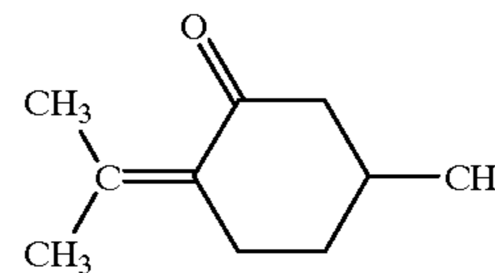
pulegone
