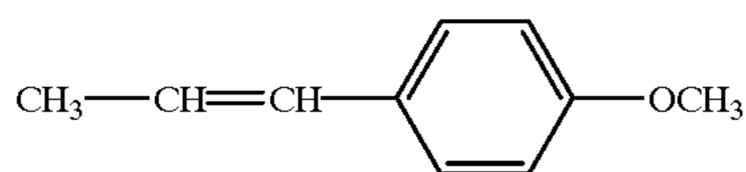
trans-anethole
