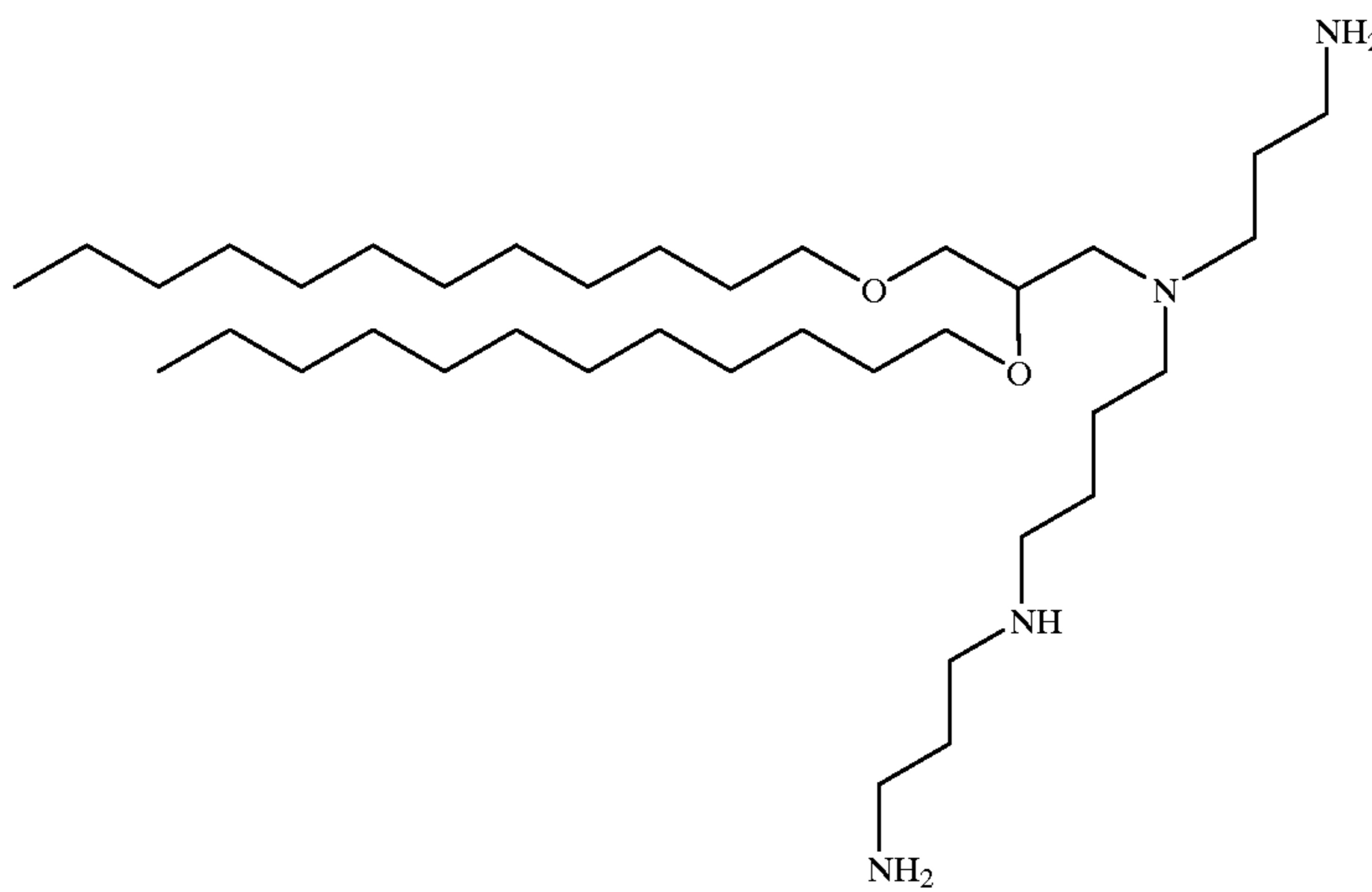
N 4 -spermine)-2,3-dilauryl-oxypropylamine
