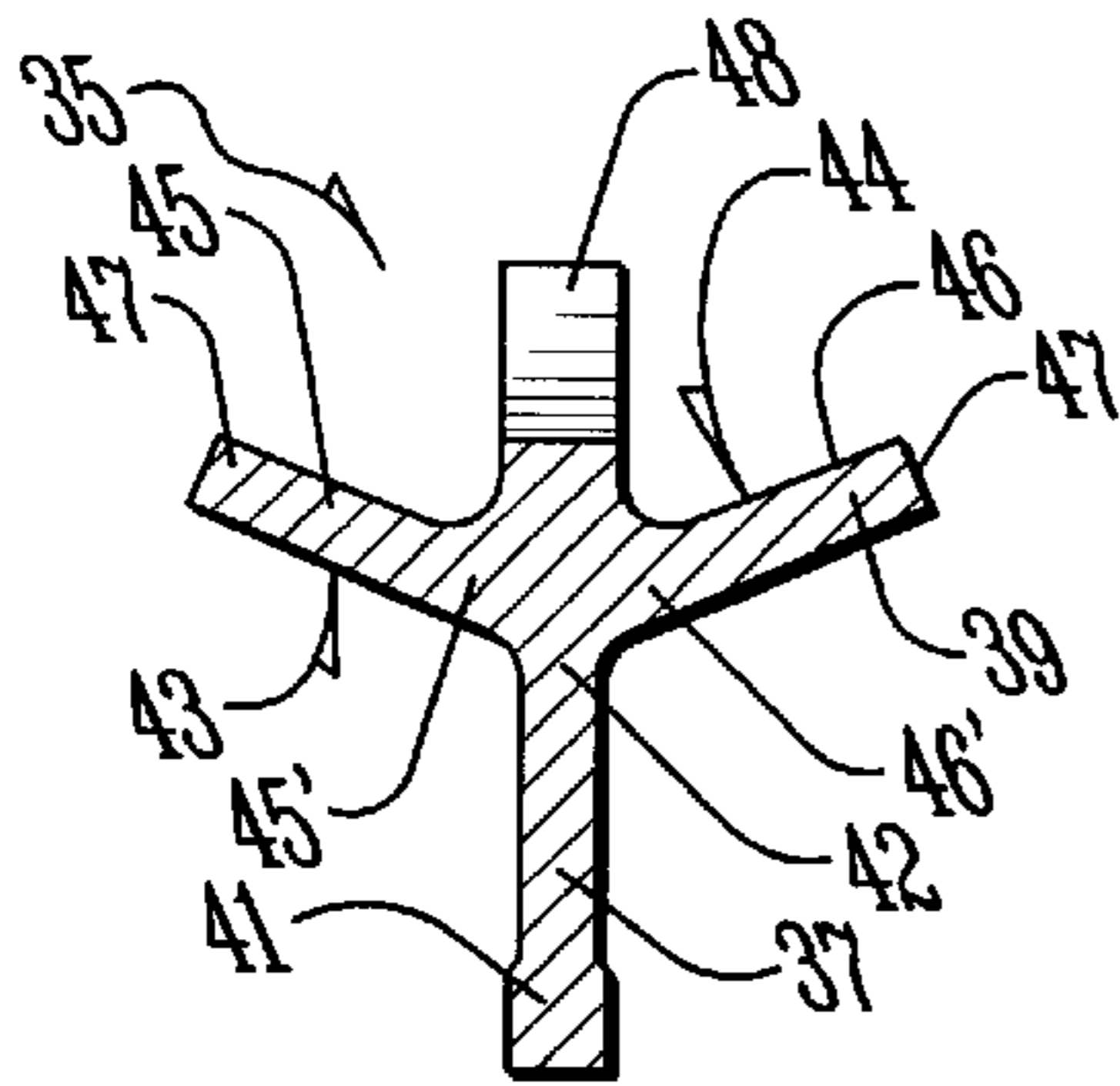
Fig. 15 ( PRIOR ART )
