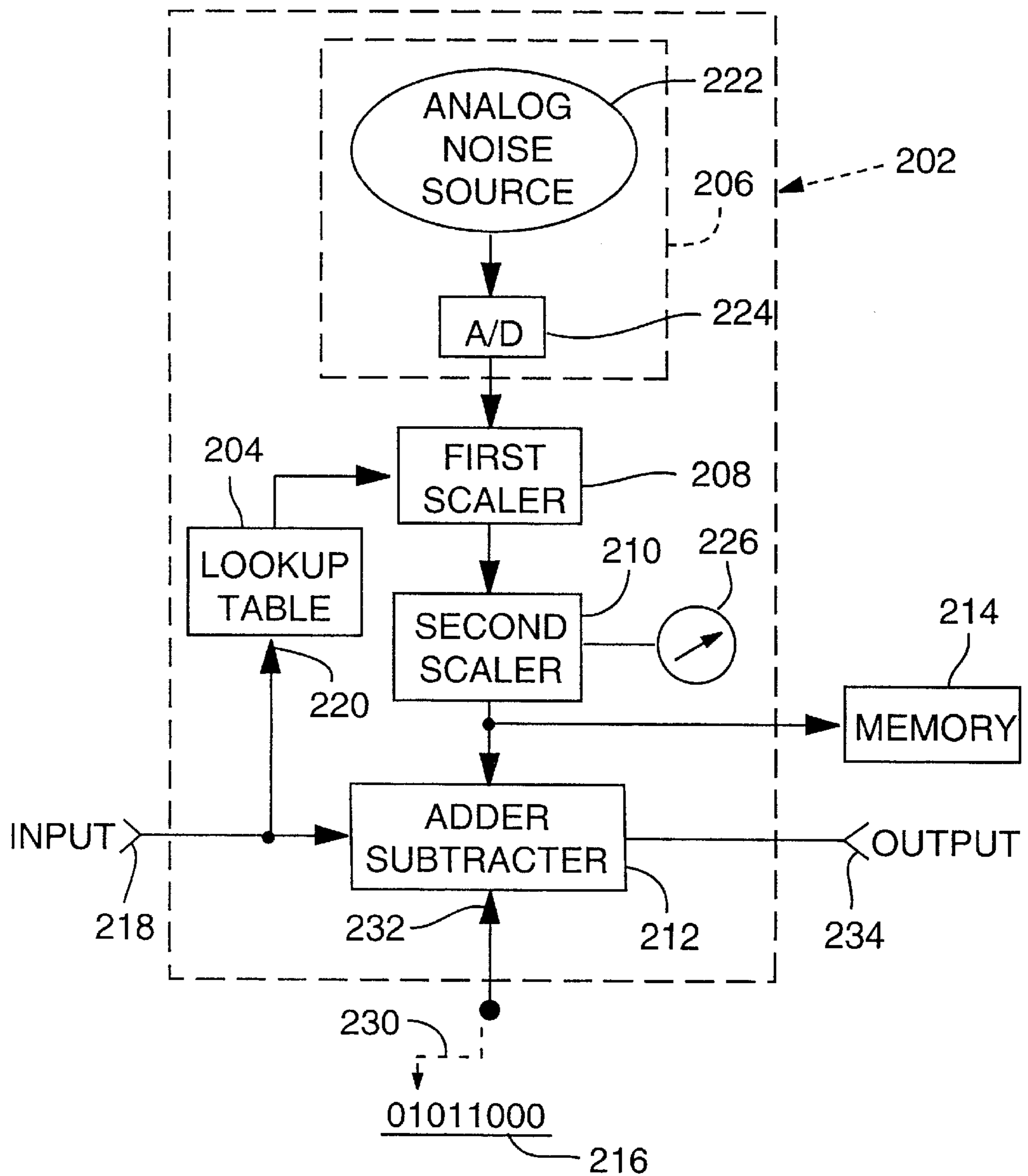
FIG. 6
