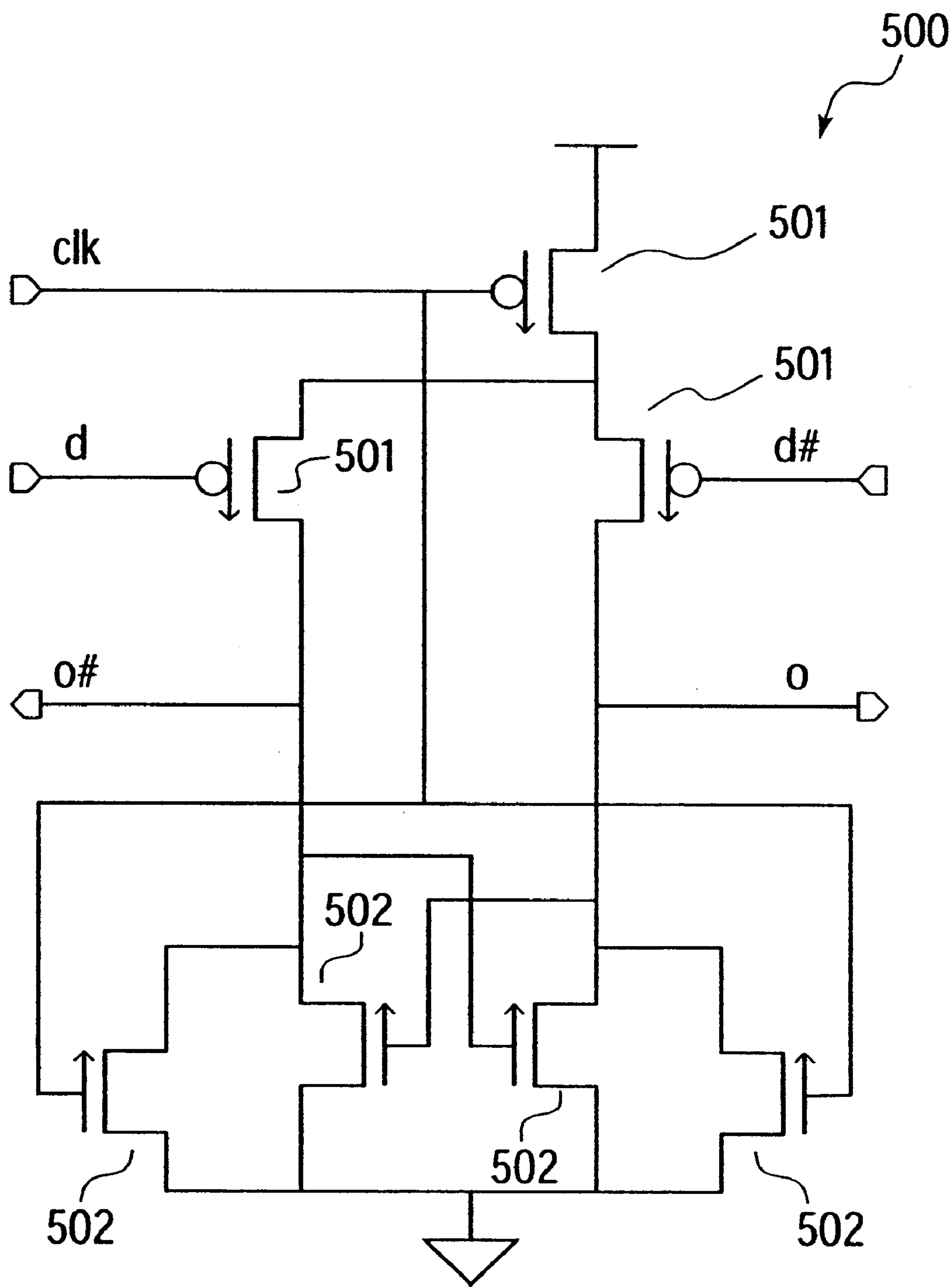
Ratioed PFET sense amp
