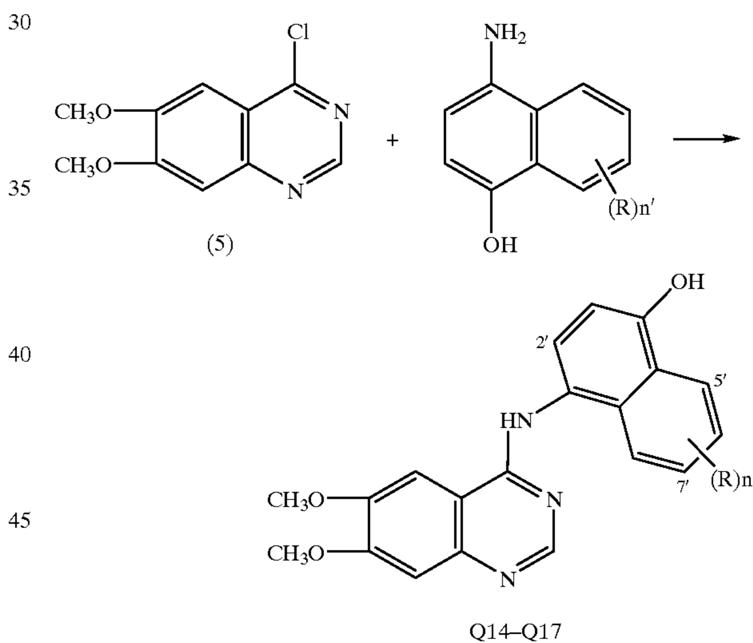
Scheme 3D Synthesis of quinazoline derivatives Q14-Q17
