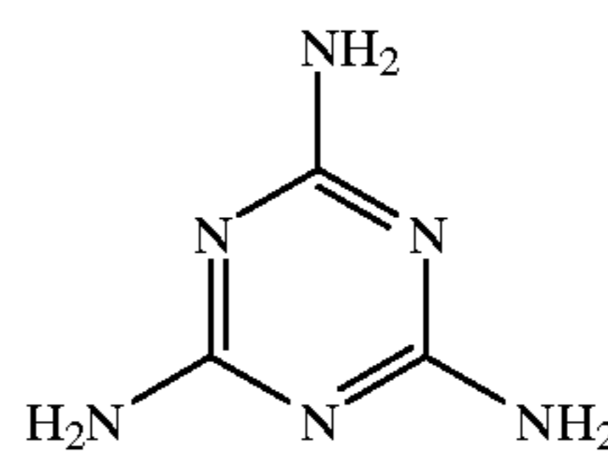
melamine
