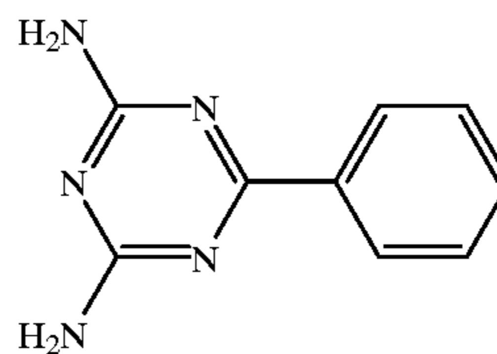
benzoguanamine
