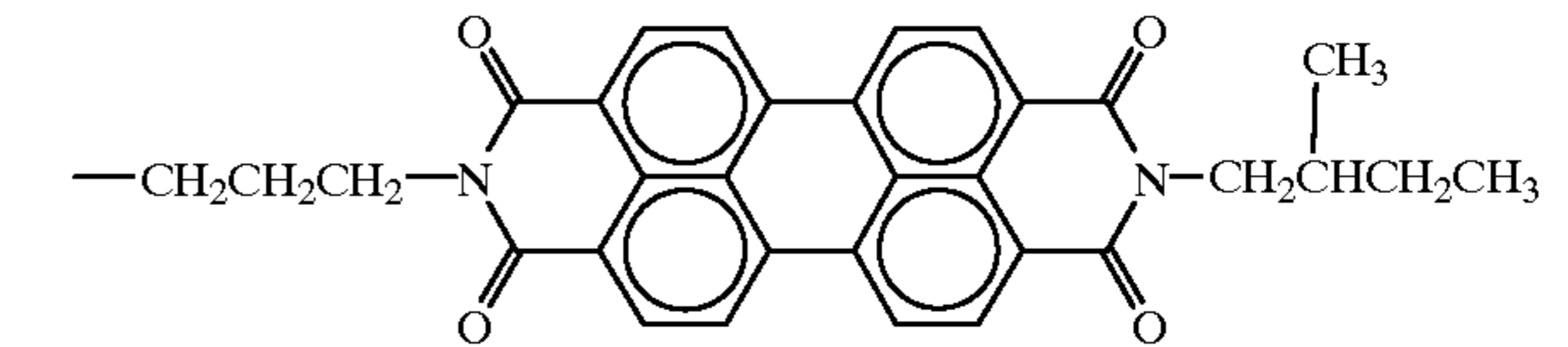
1,3-bis(2-methylbutylimido peryleneimido)propane
