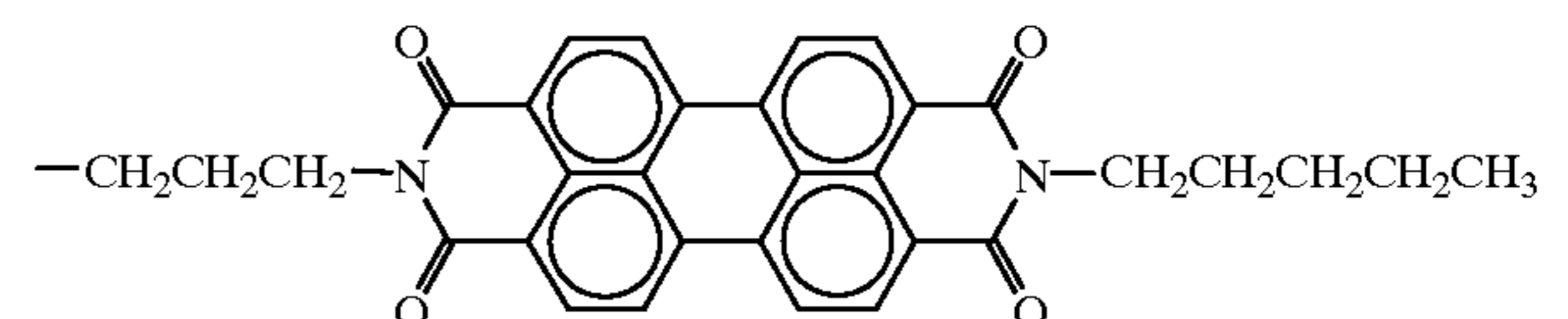
1,3-bis(2-methylbutylimido peryleneimido)propane
