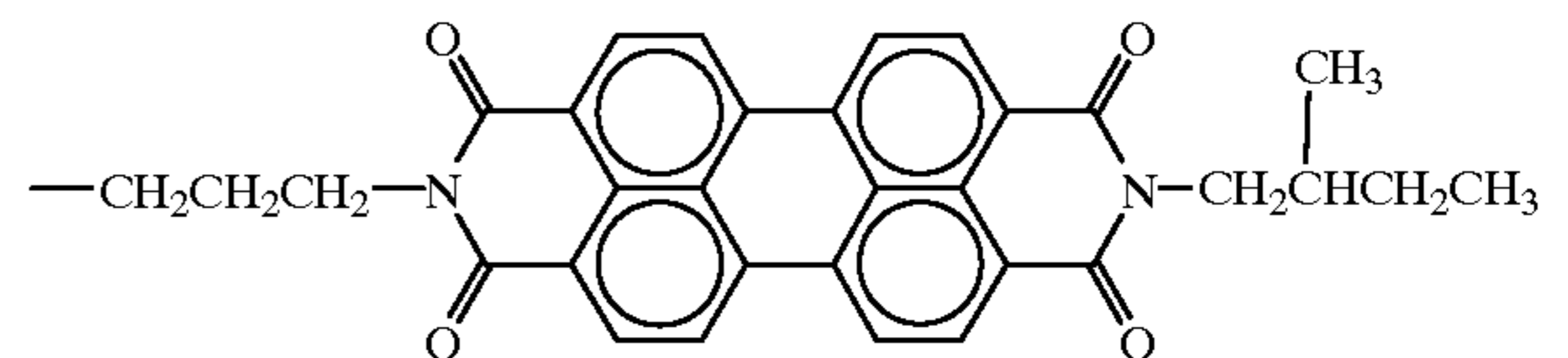
1,3-bis(2-methylbutylimido peryleneimido)propane
