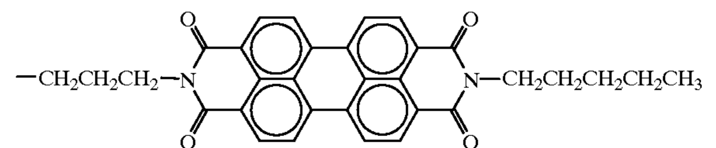
1,3-bis(2-methylbutylimido peryleneimido)propane
