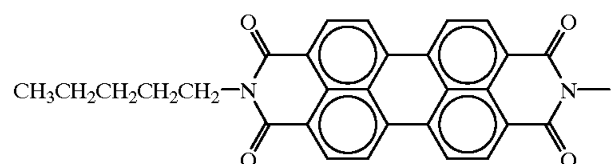
1,3-bis(2-methylbutylimido peryleneimido)propane
