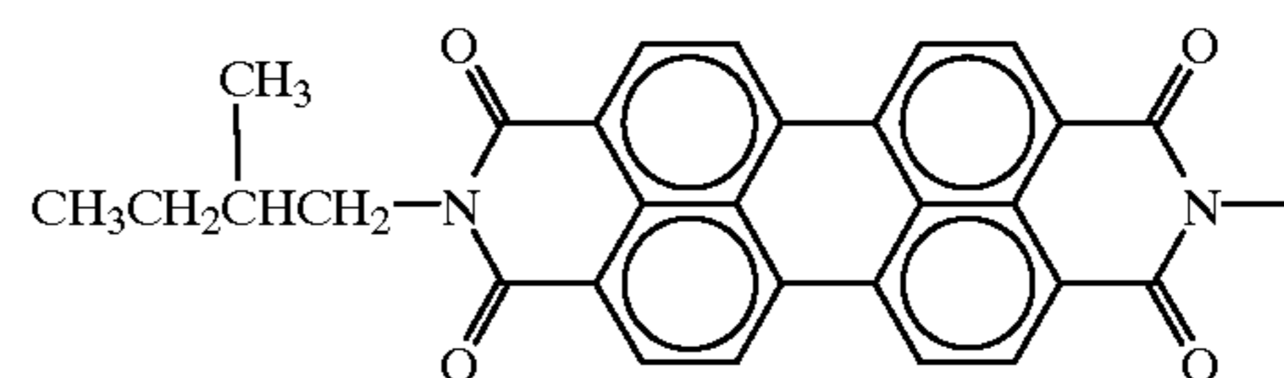
1,3-bis(2-methylbutylimido peryleneimido)propane
