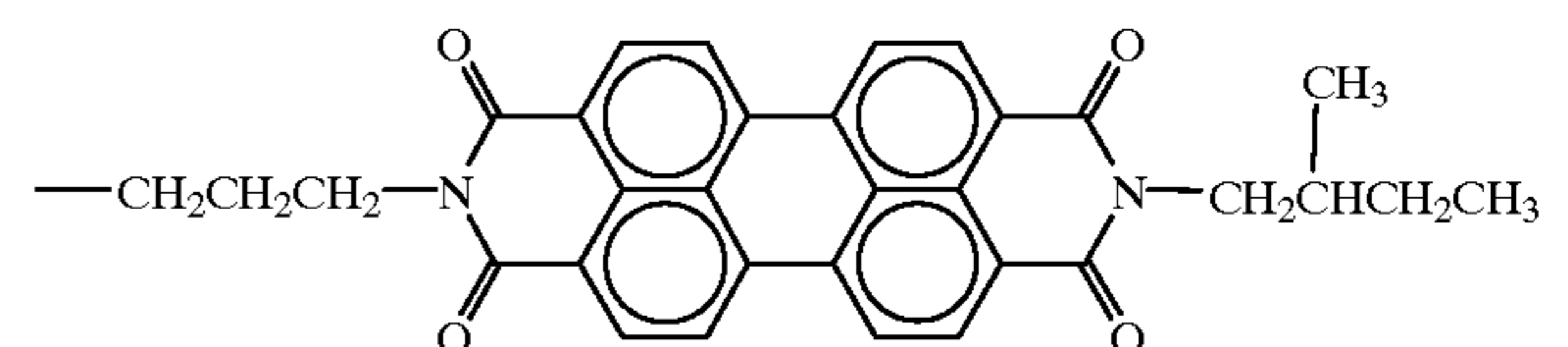
1-(n-pentylimidoperyleneimido)-3-(2-methylbutylimido peryleneimido)propane
