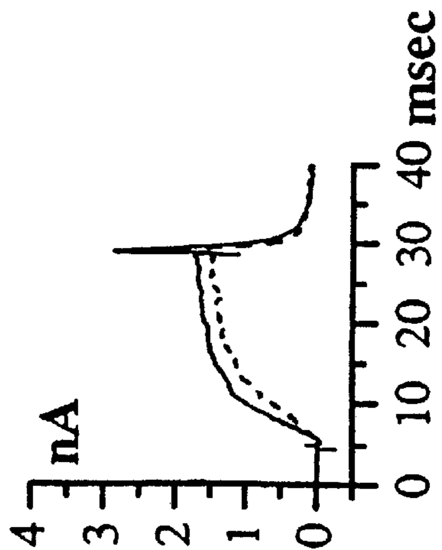
FIG. 4a acetate
