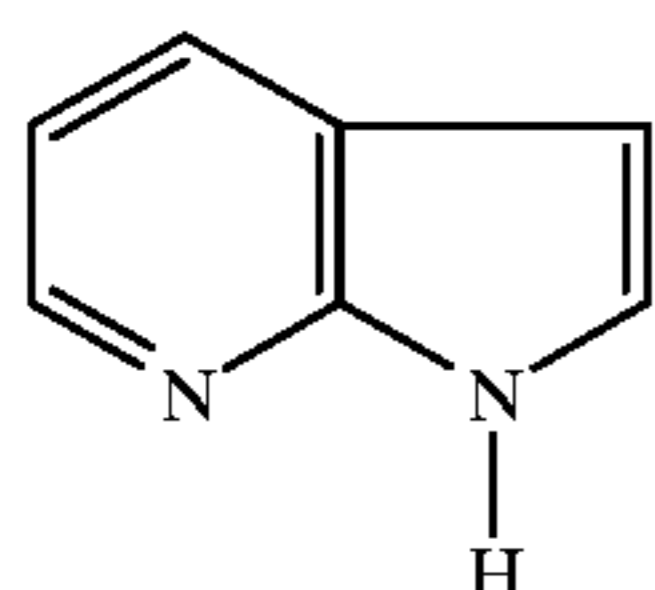
7-azaindole
