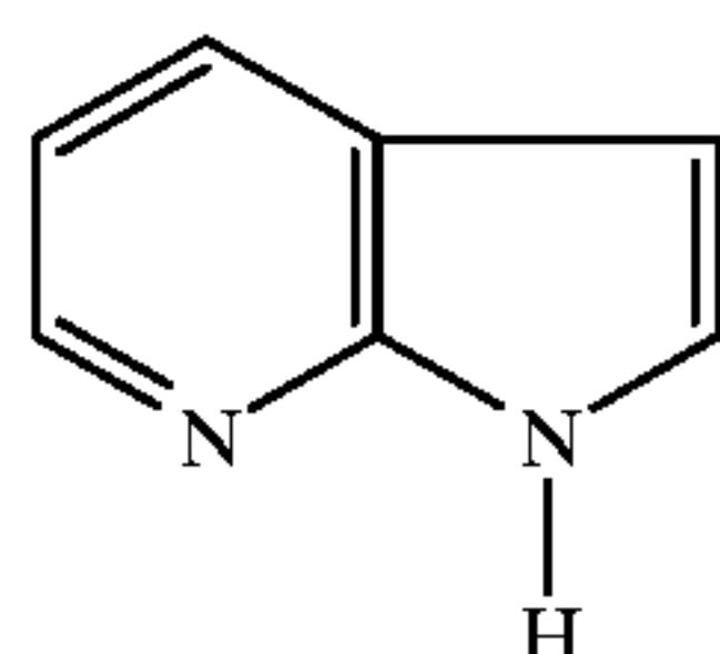
7-azaindole
