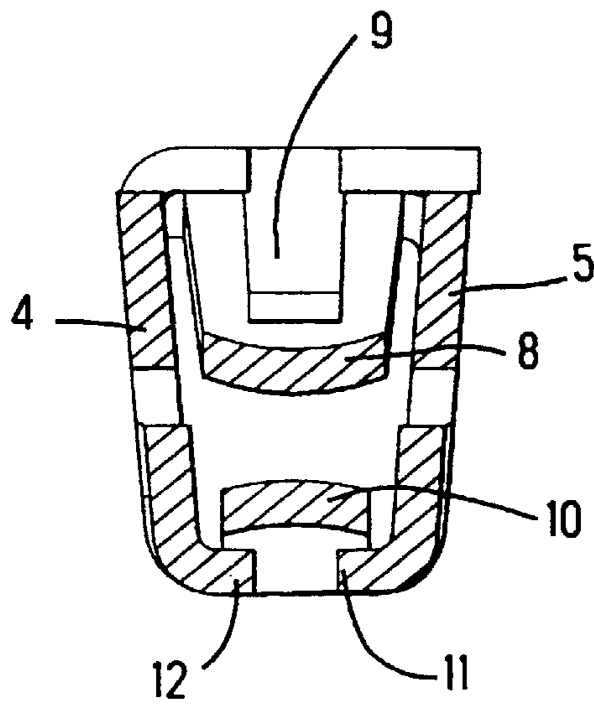
A-A Fig. 9
