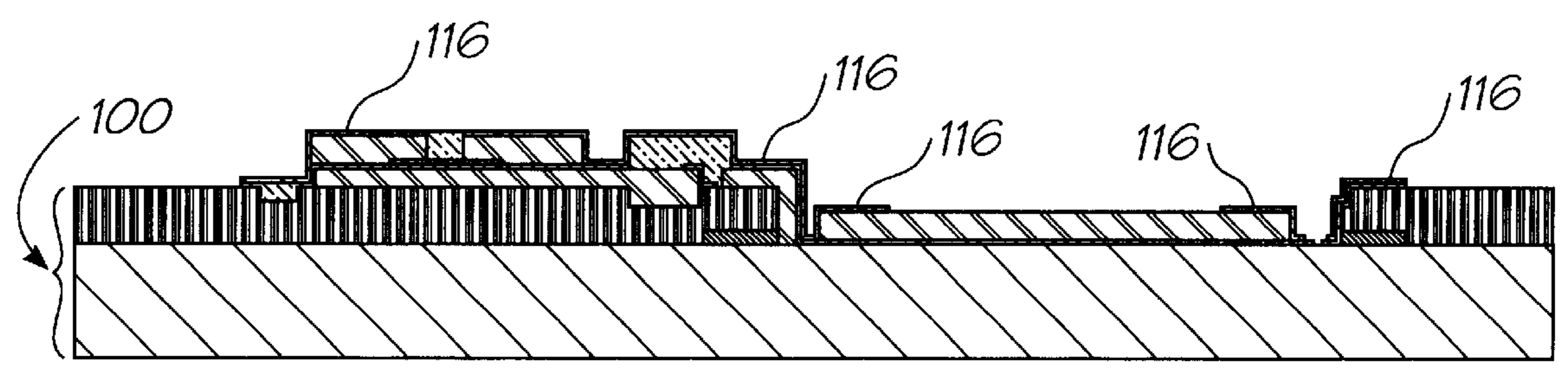
0.05 micron Si_xN_yH_z 0.2 micron TiN
