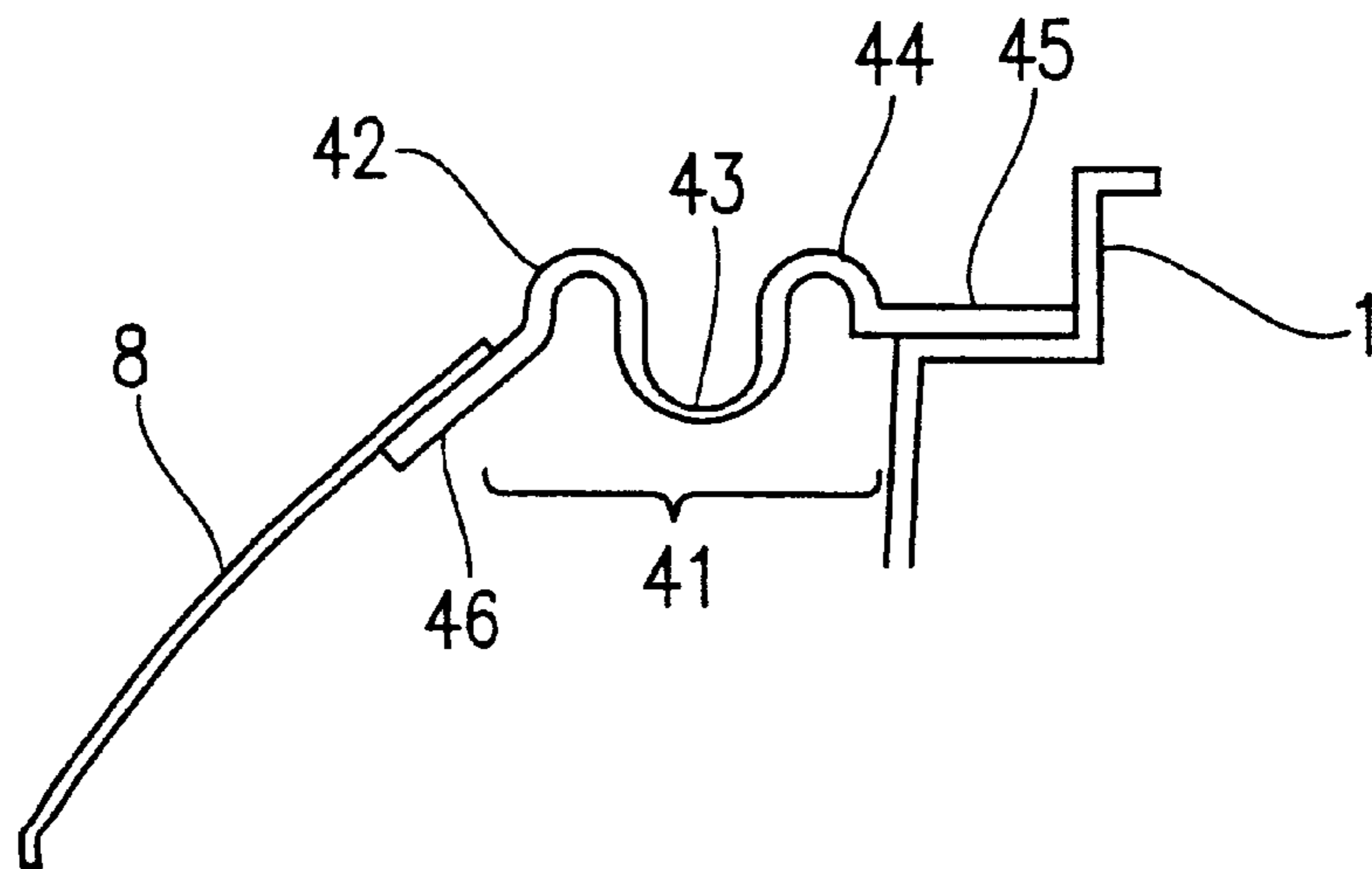
FIG. 6B
