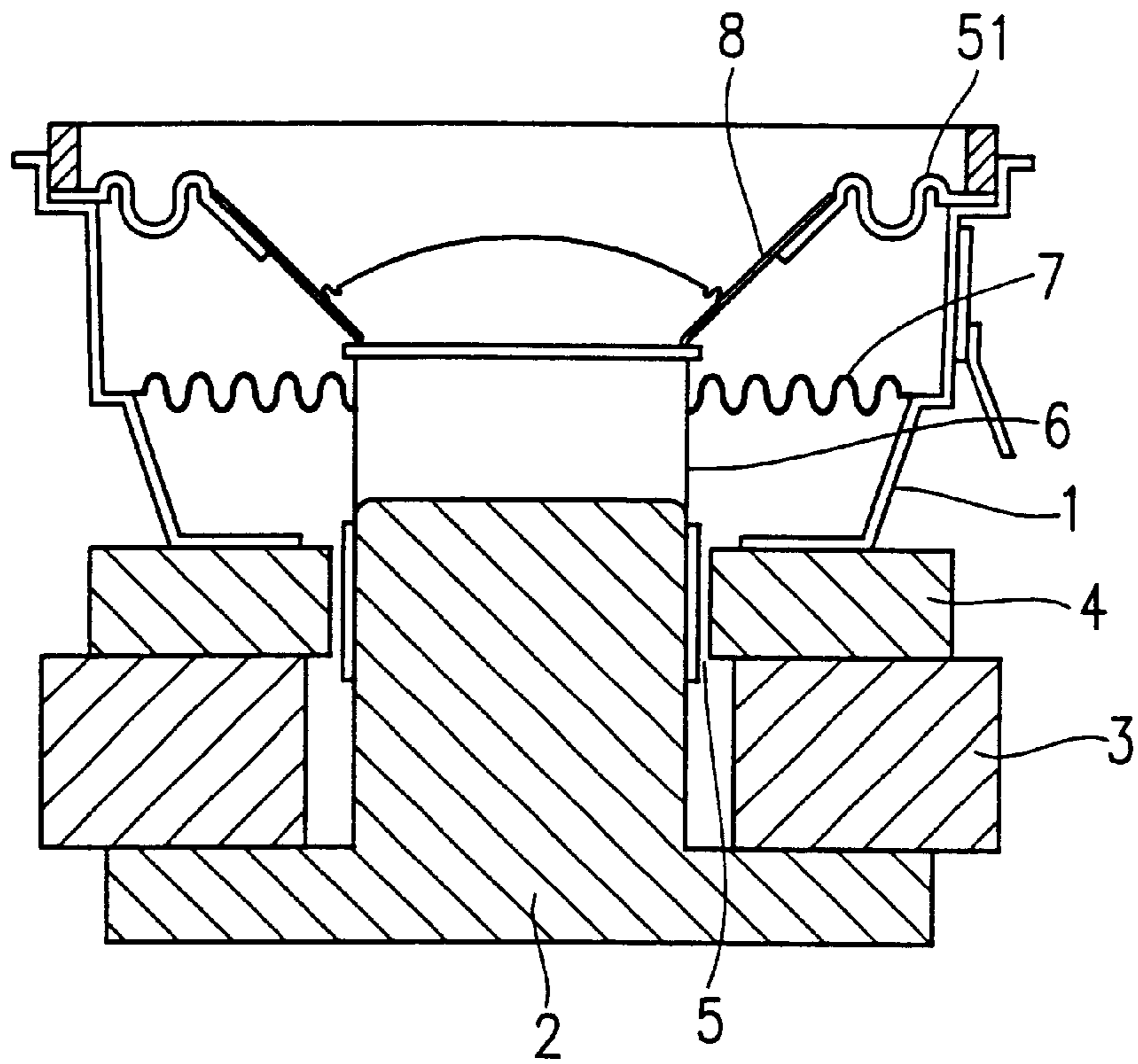
FIG. 7A
