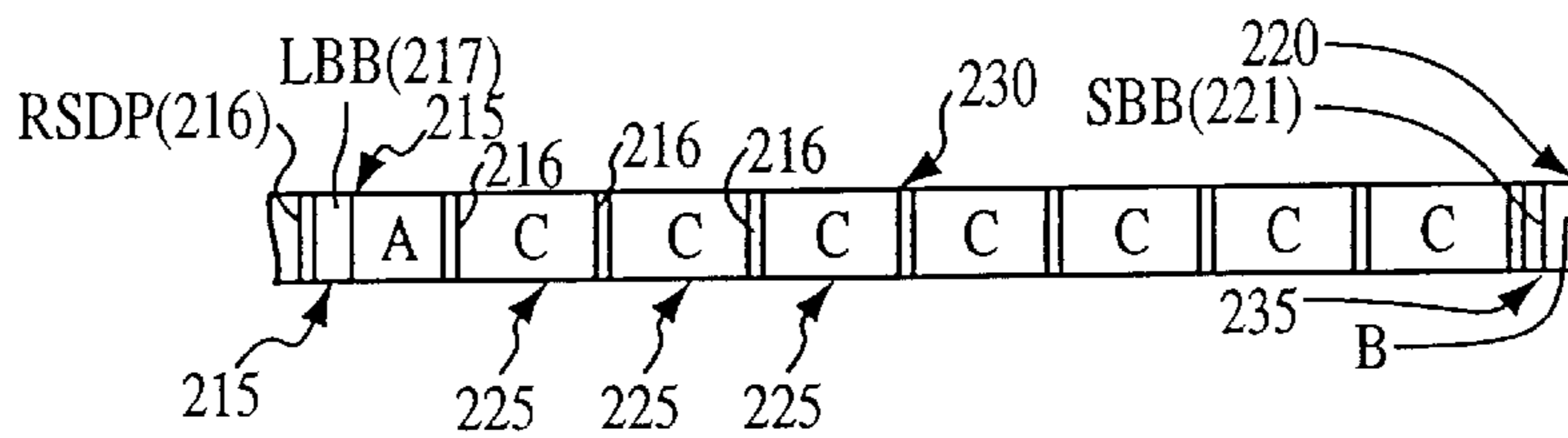
FIG. 6B FRAME TYPE A
