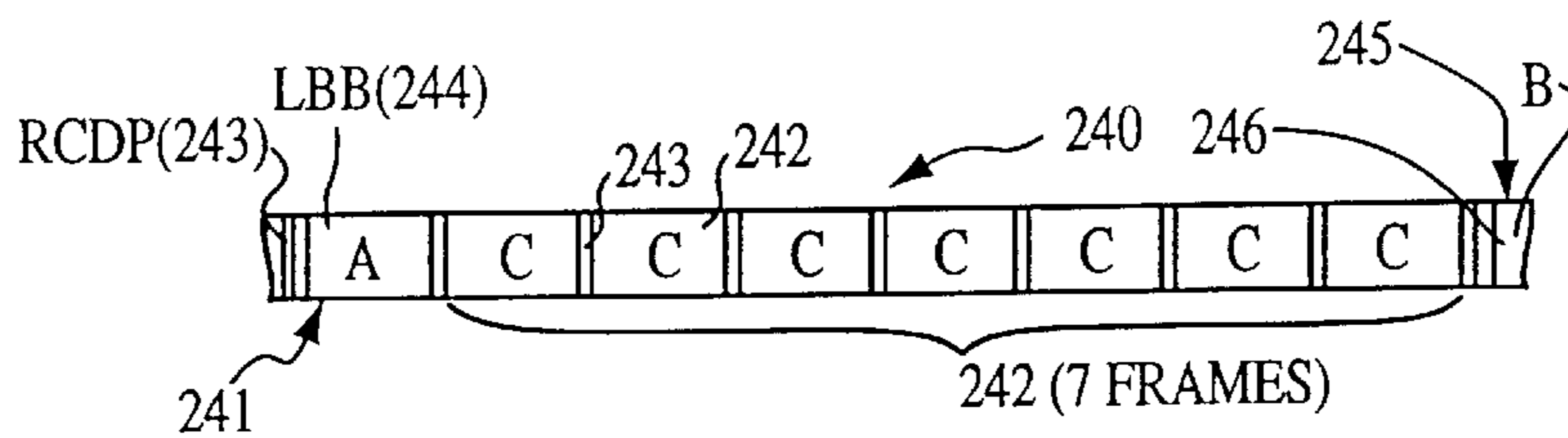
FIG. 6F 1200 BPS
