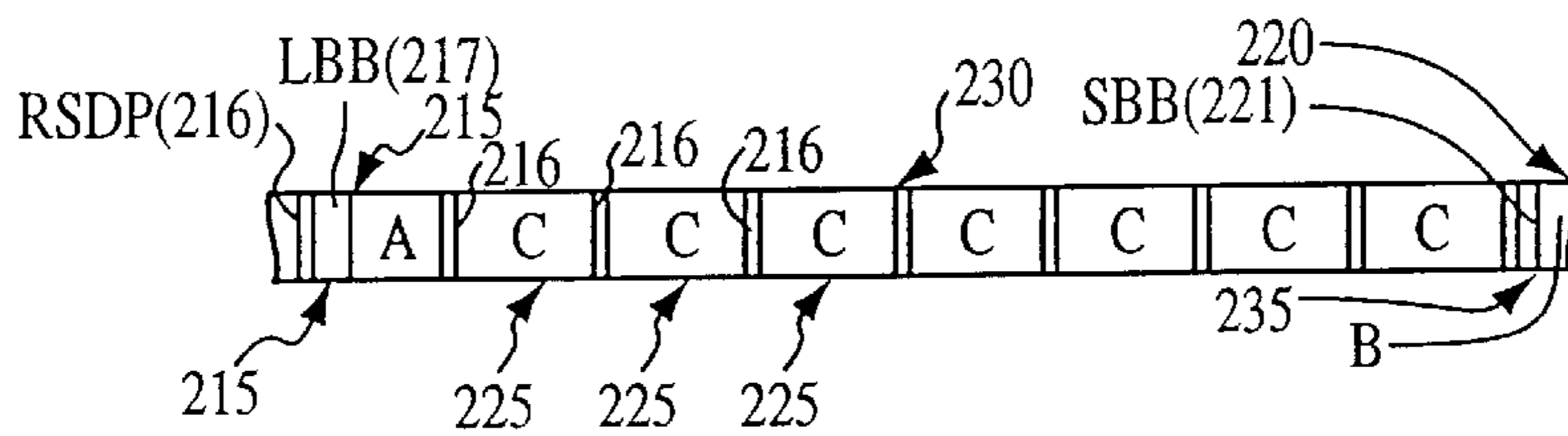
FIG. 6E 600 BPS
