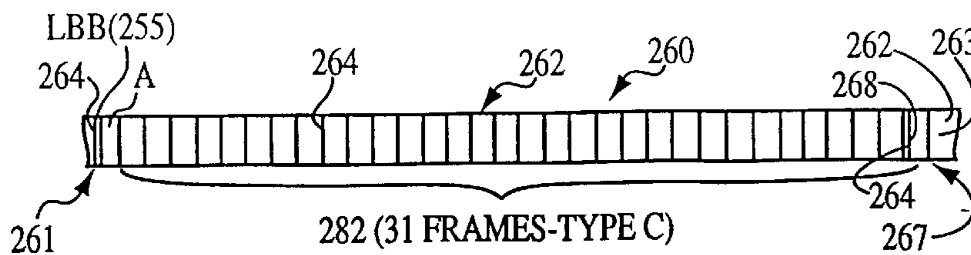
FIG. 6H 4800 BPS
