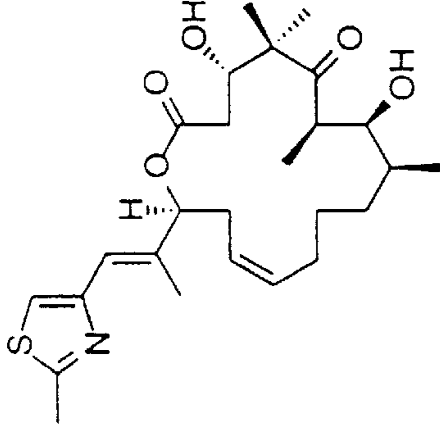
desoxyepothilone A
