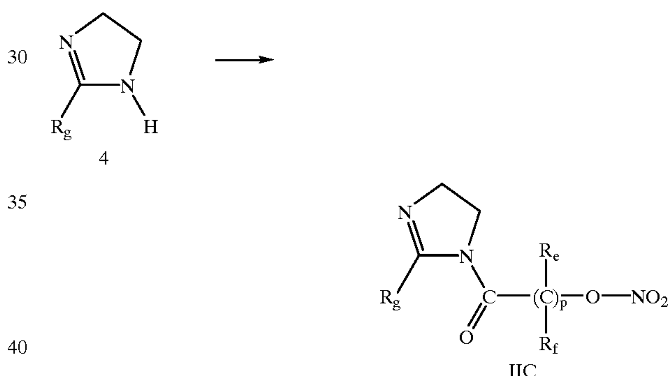
Scheme VI
