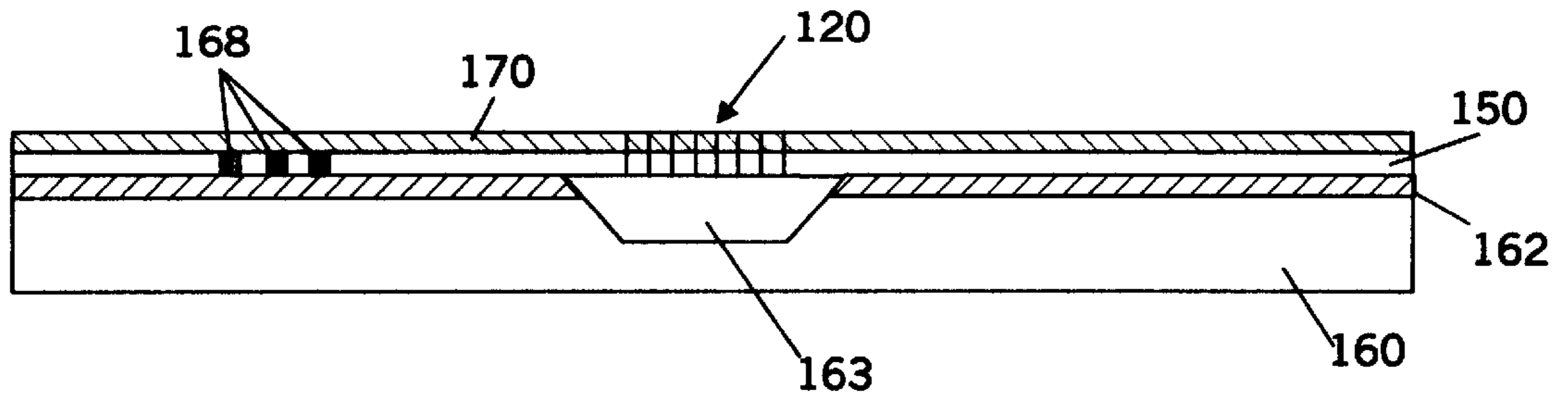
FIG. 3E
