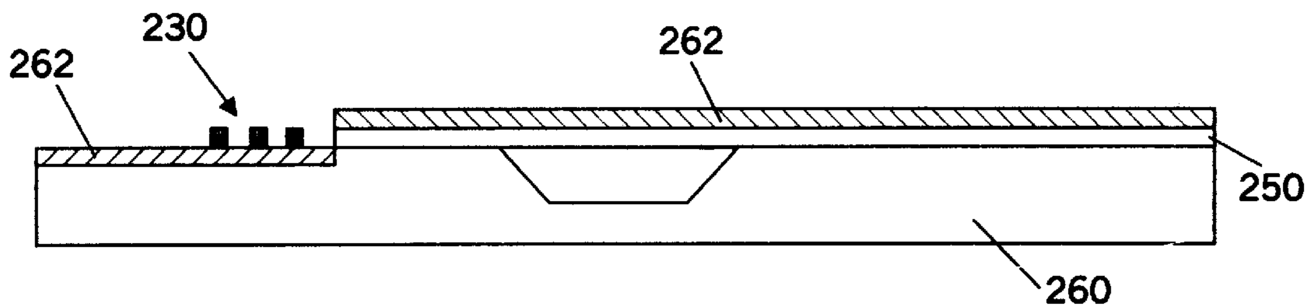
FIG. 4E
