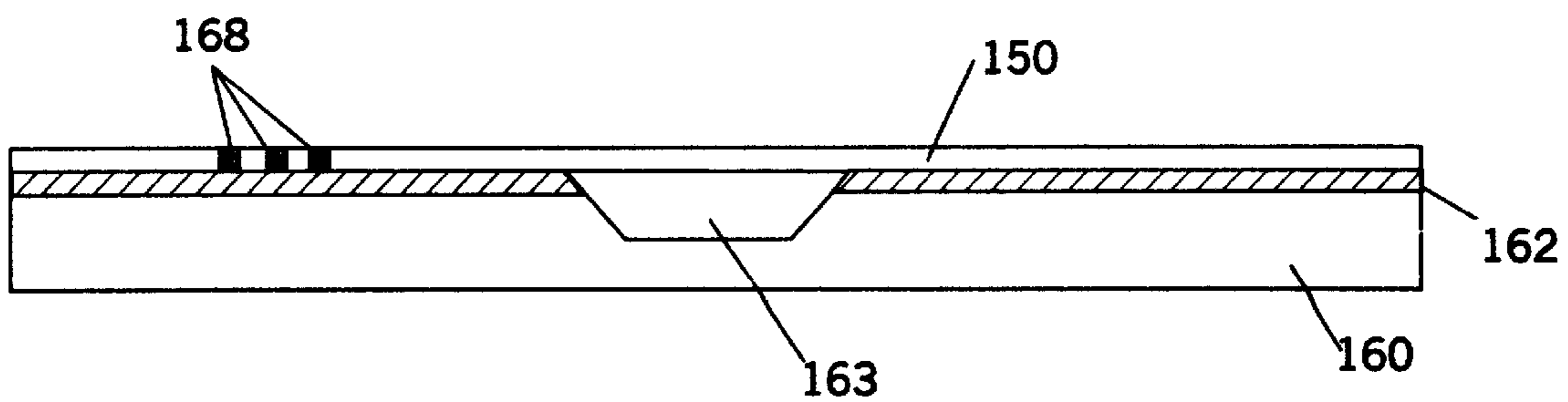
FIG. 3C
