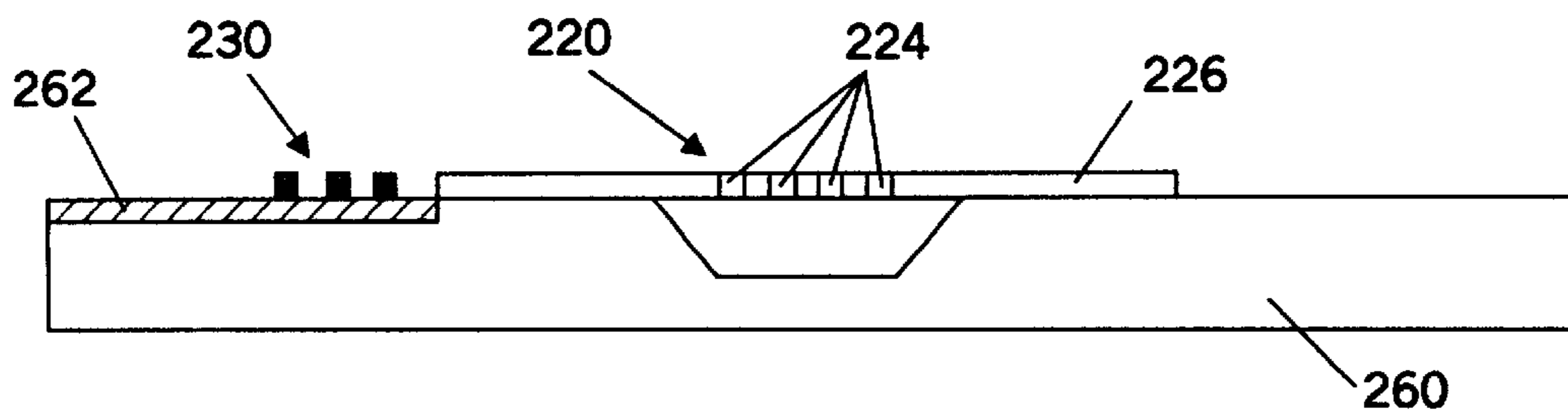
FIG. 4F
