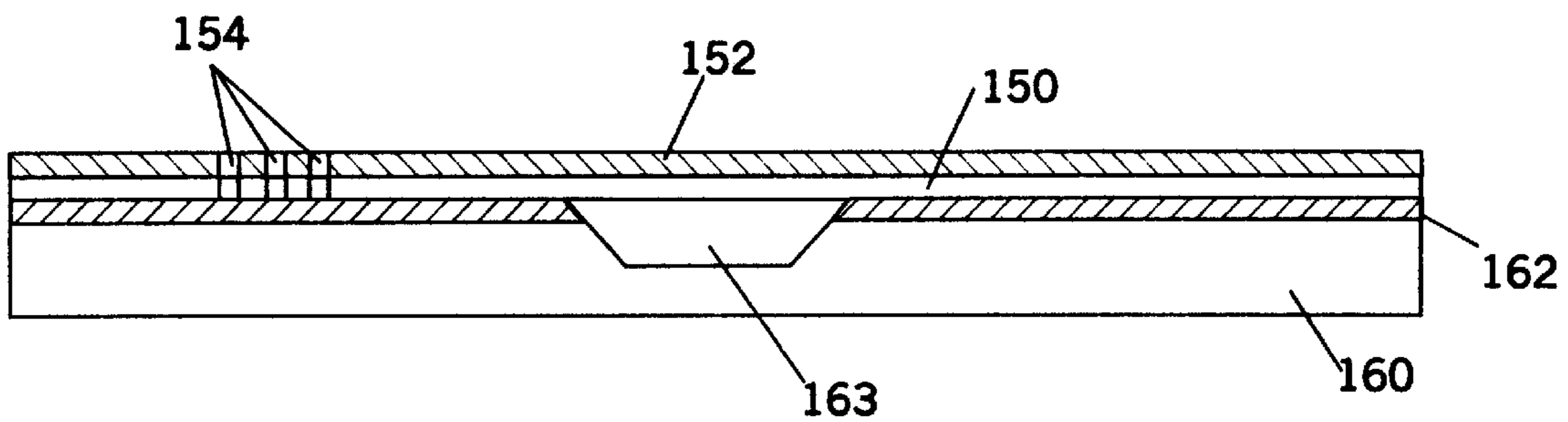
FIG. 3C
