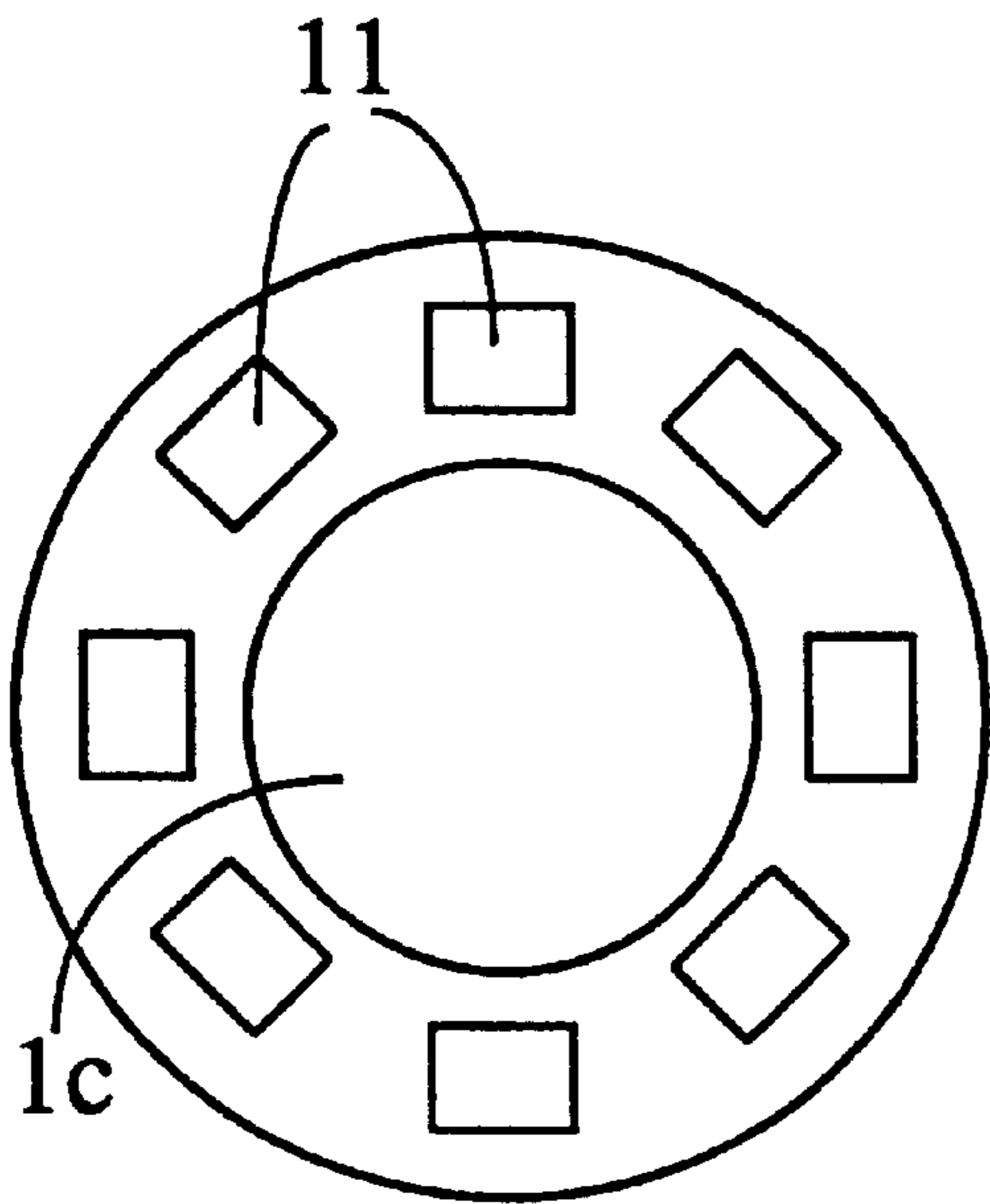
FIG. 19A
