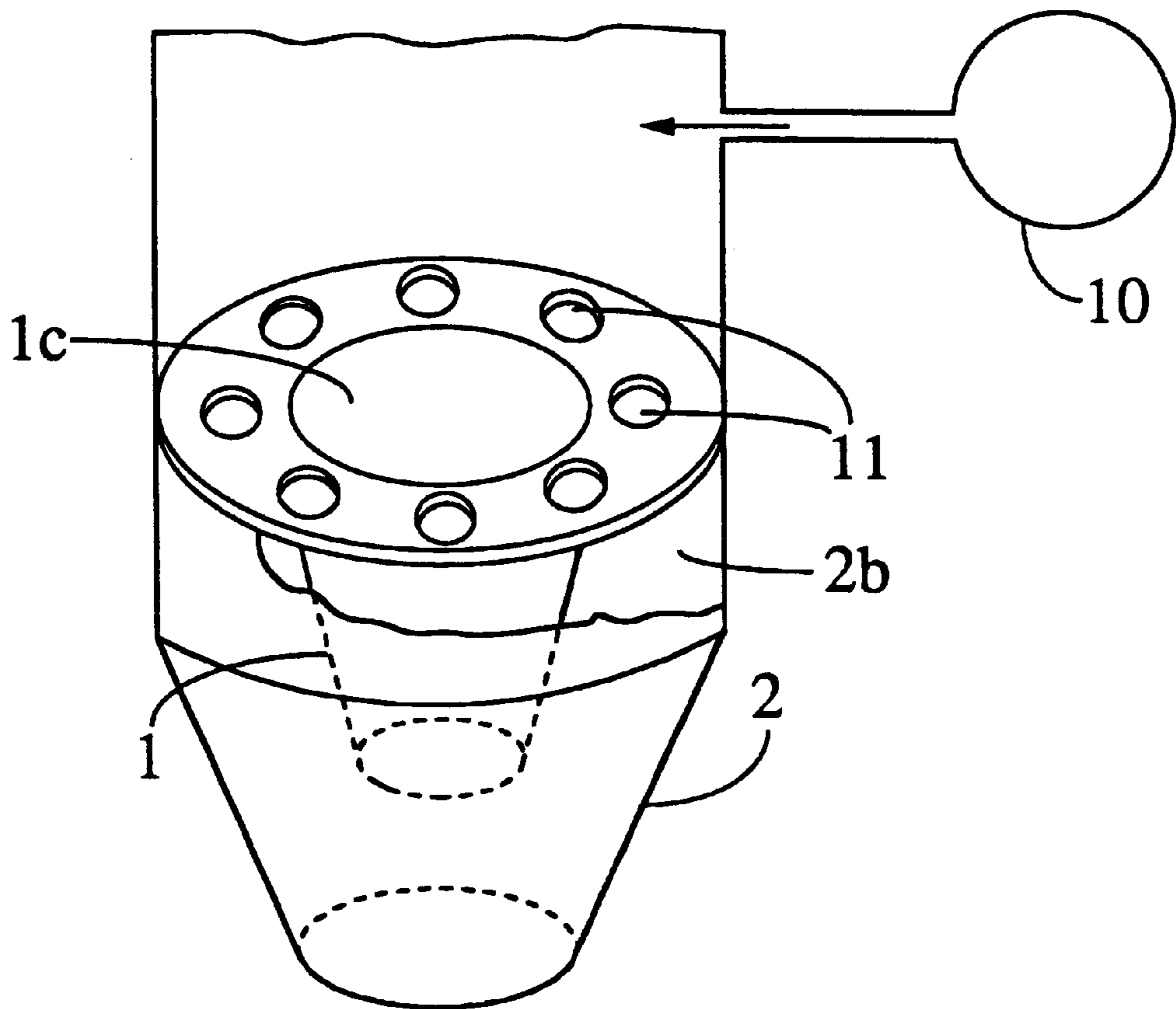
FIG. 18
