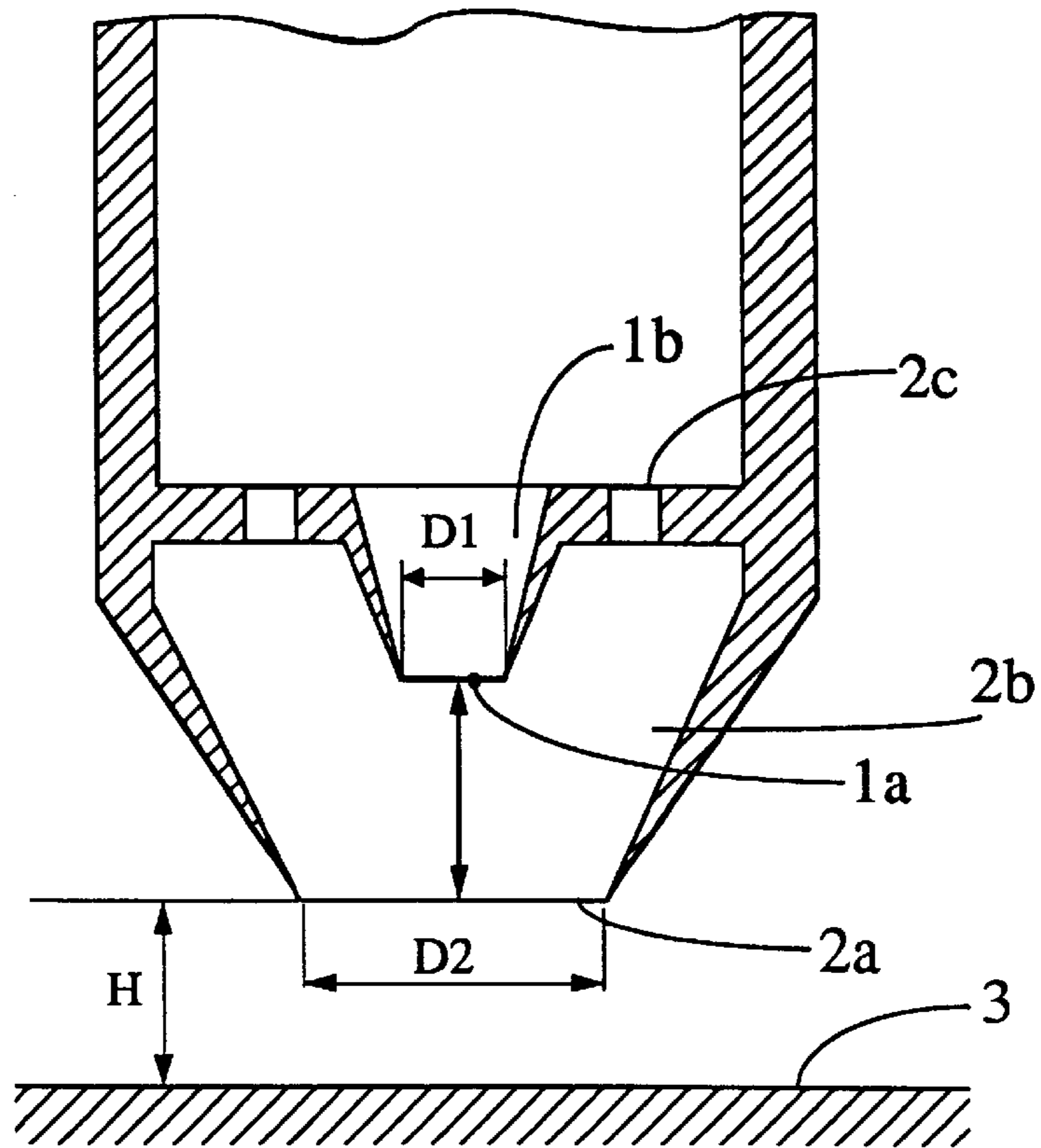
FIG. 7
