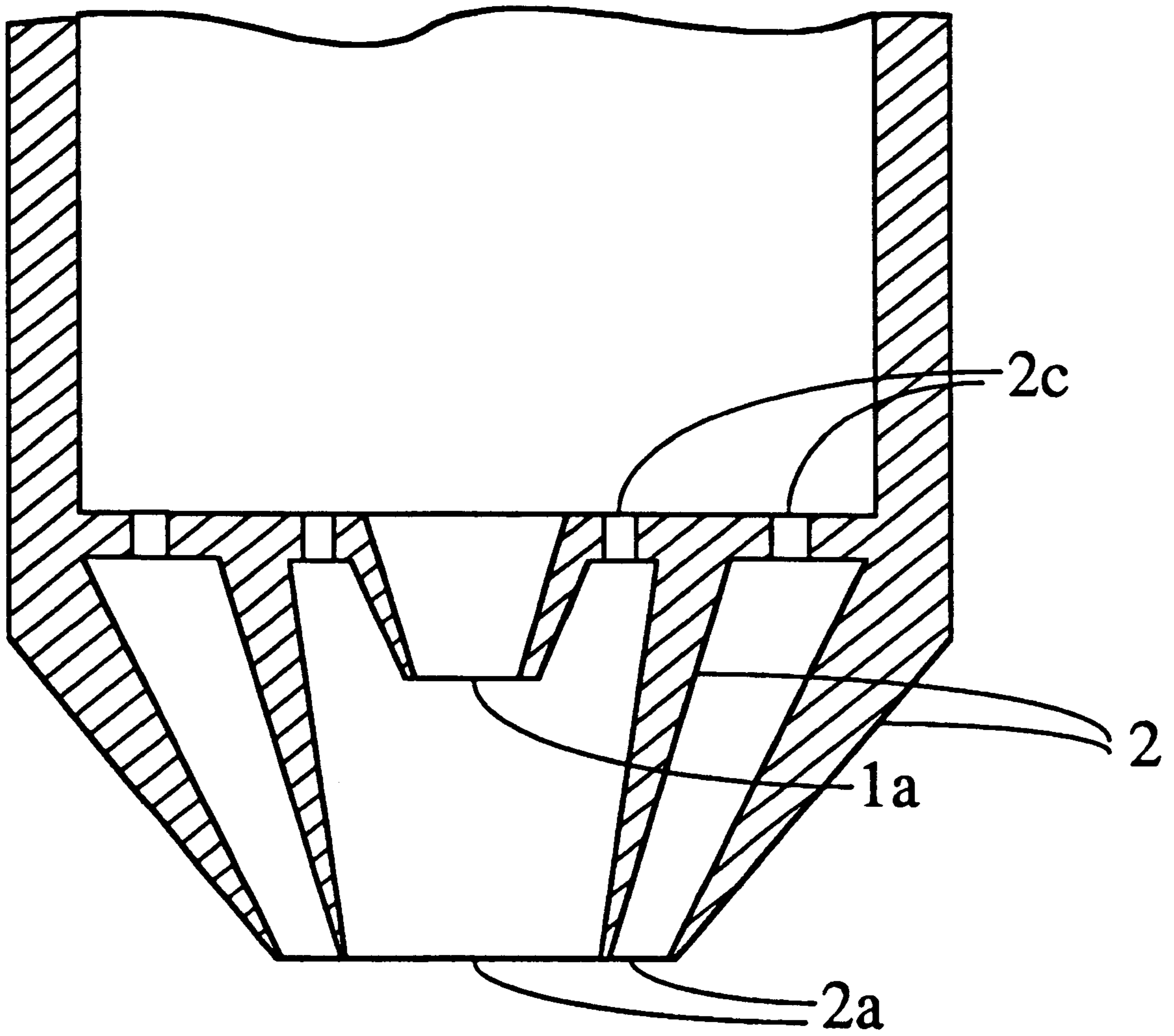
FIG. 9
