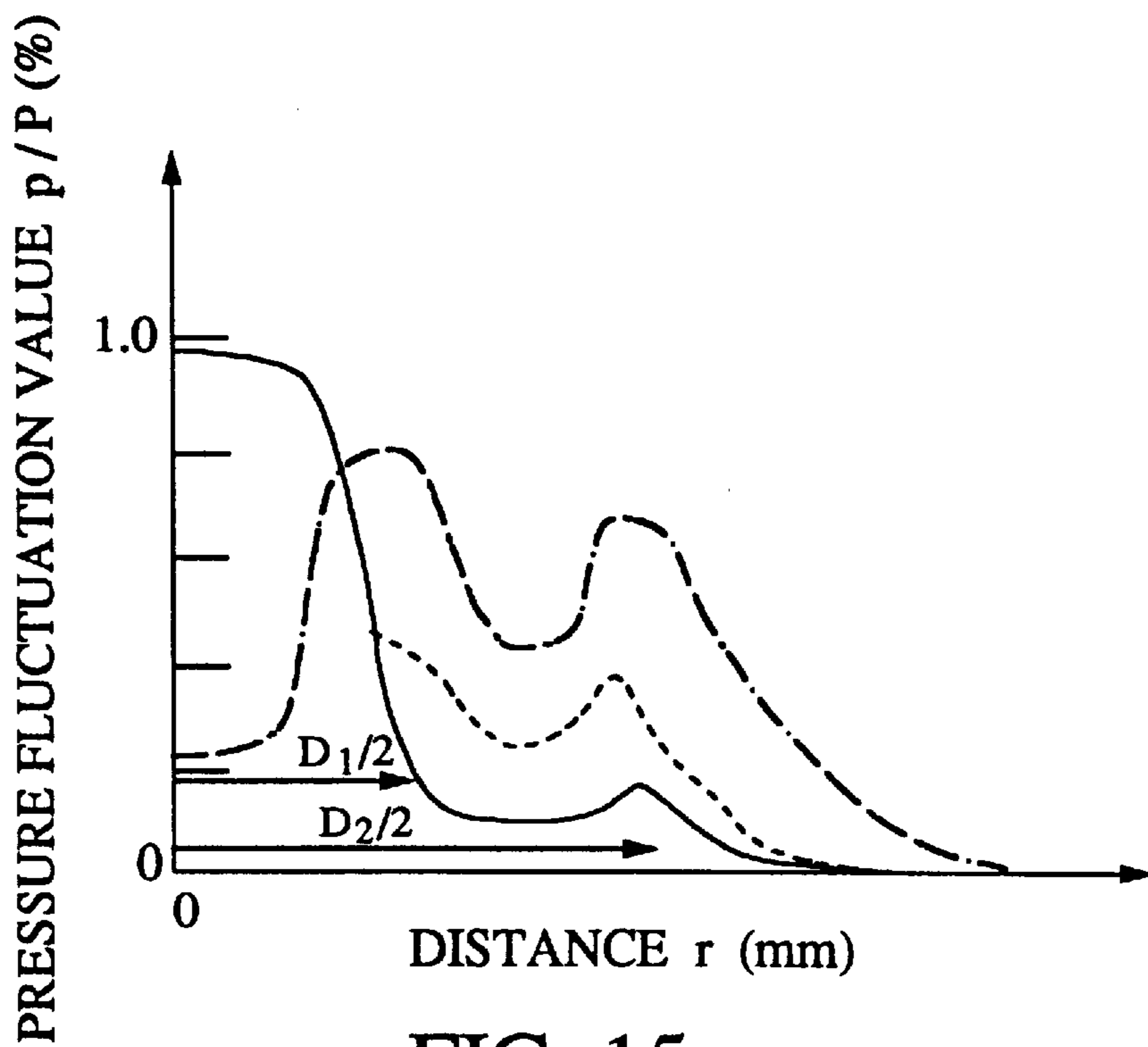
FIG. 15
