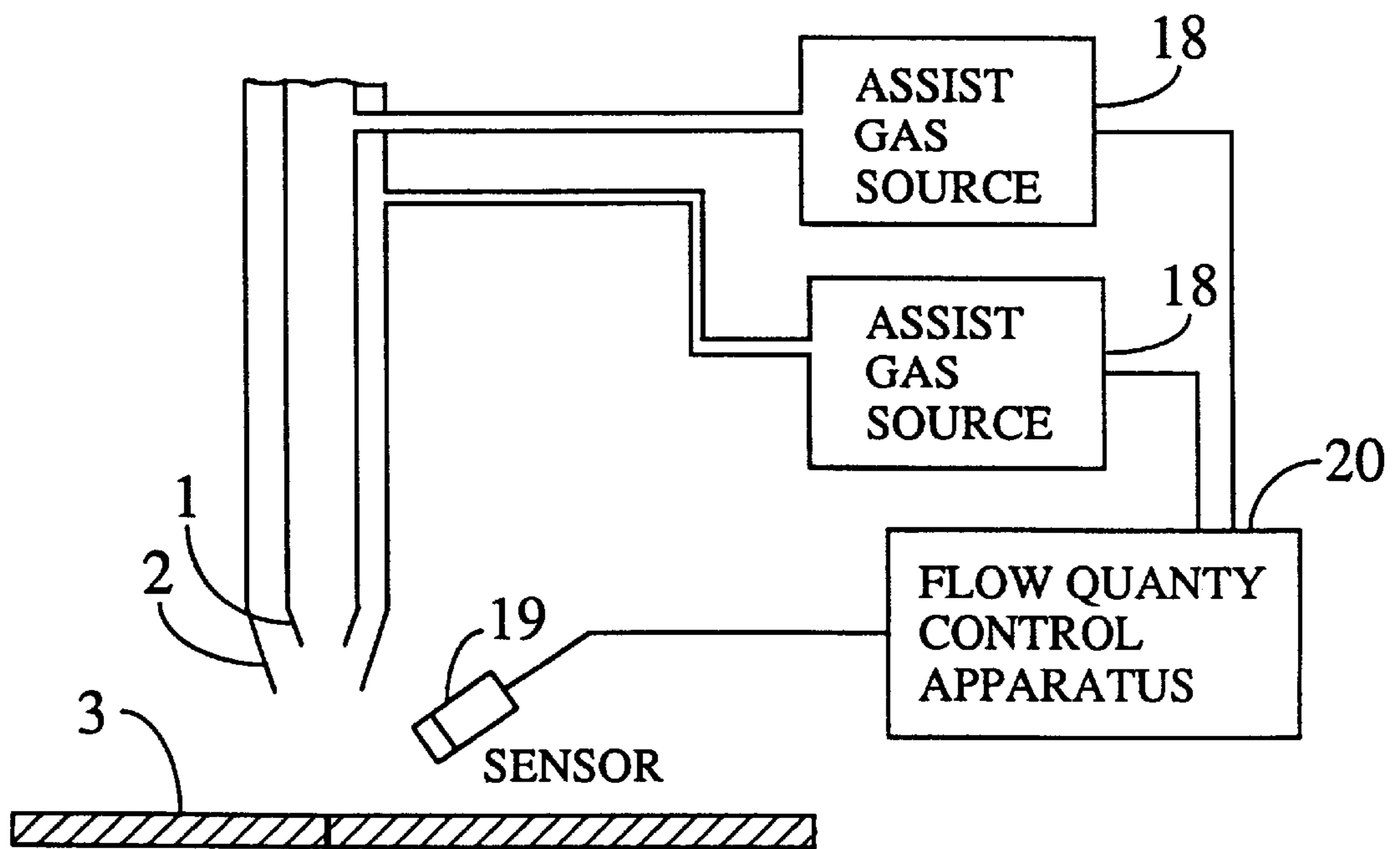
FIG. 26
