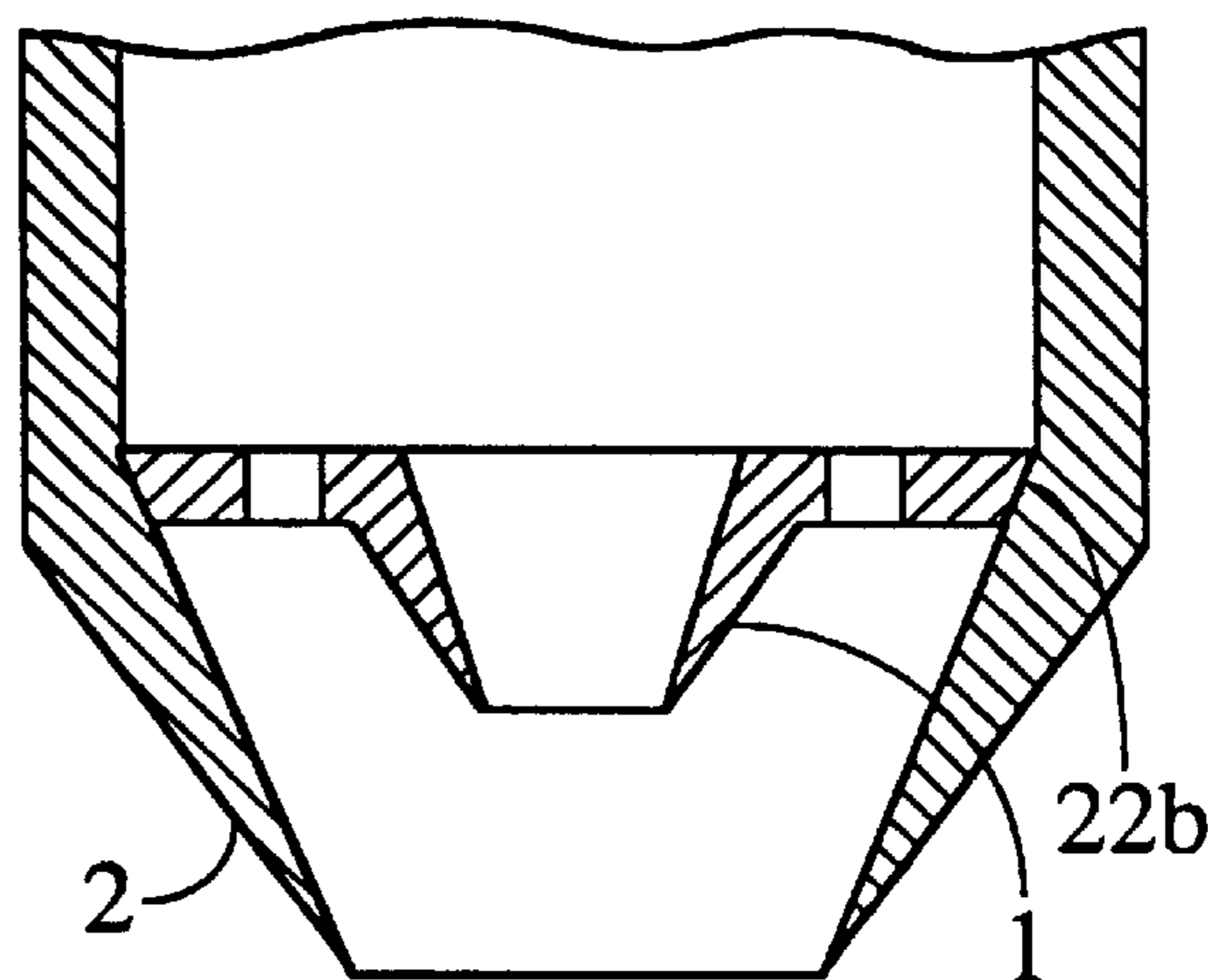
FIG. 29B
