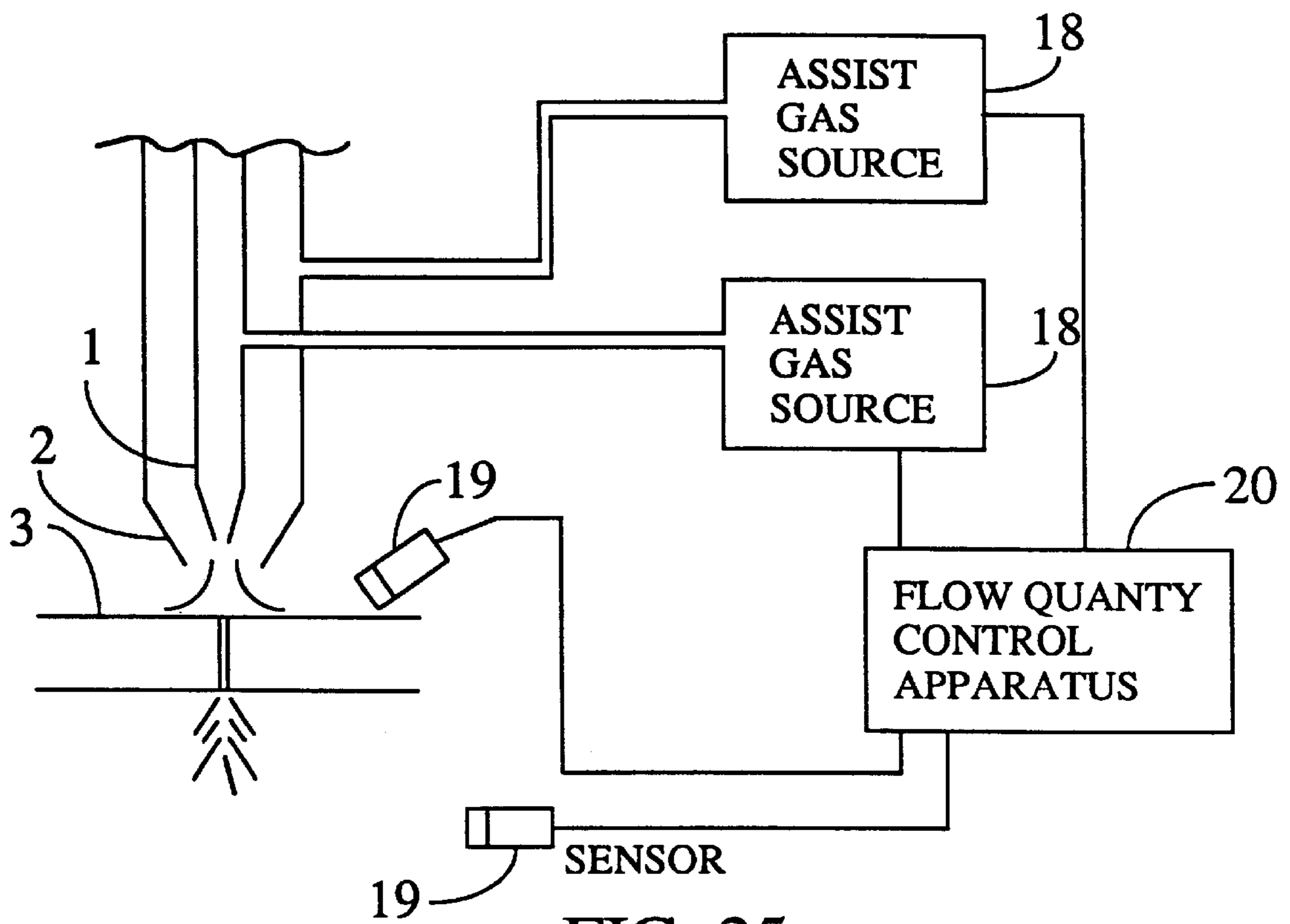
FIG. 25
