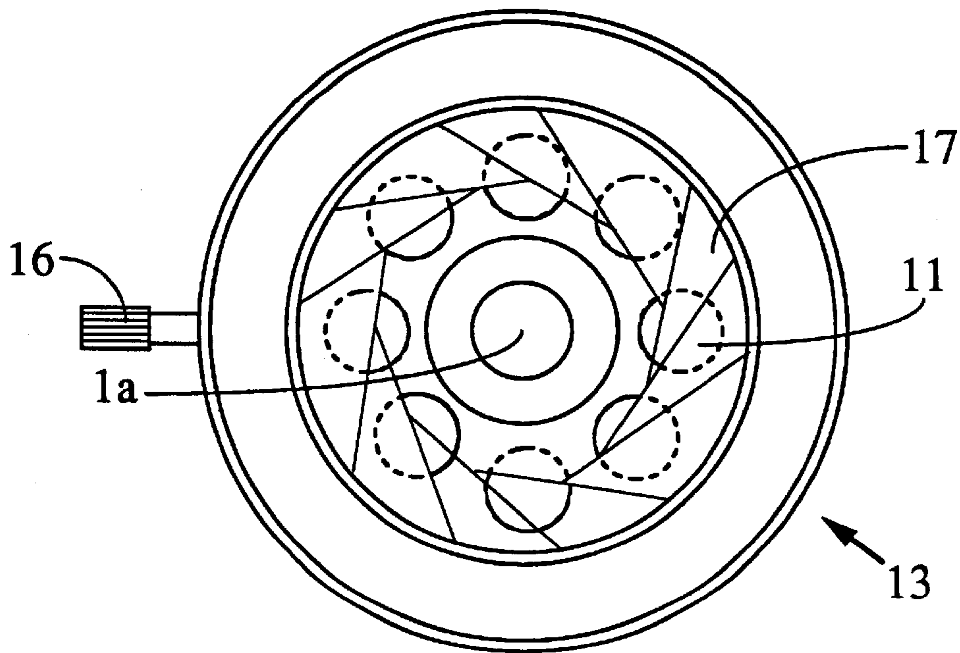
FIG. 23
