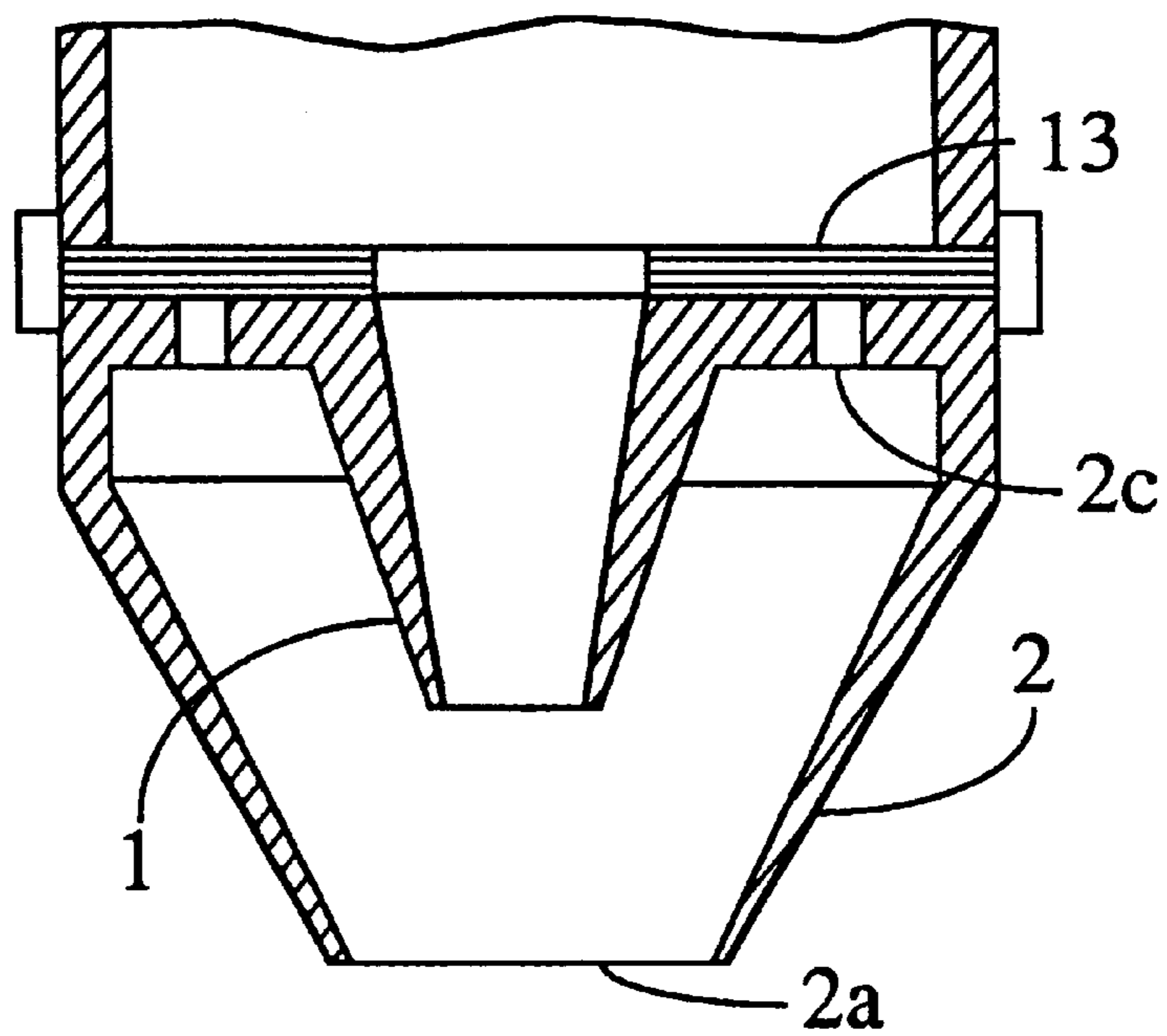
FIG. 21
