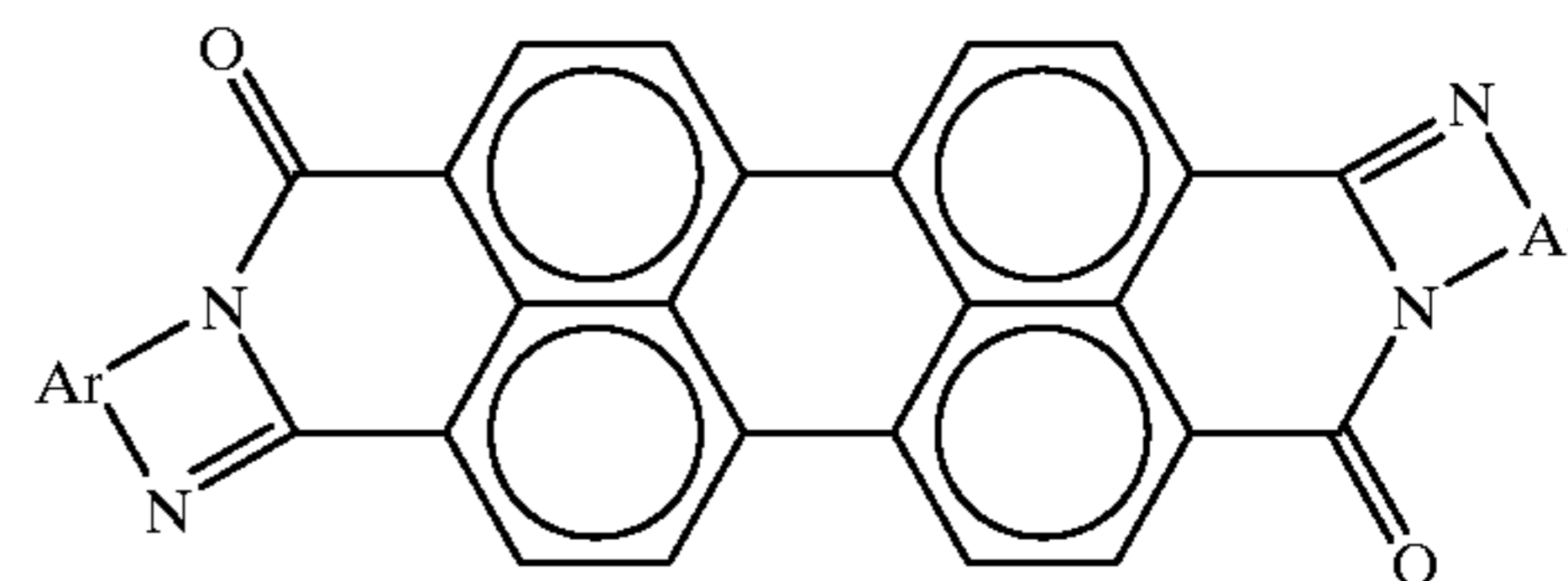
4b. Bisimidazo
