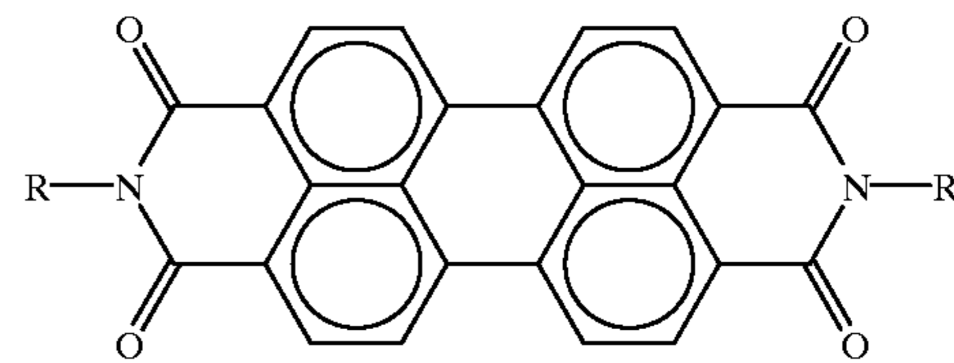
4a. Bisimide
