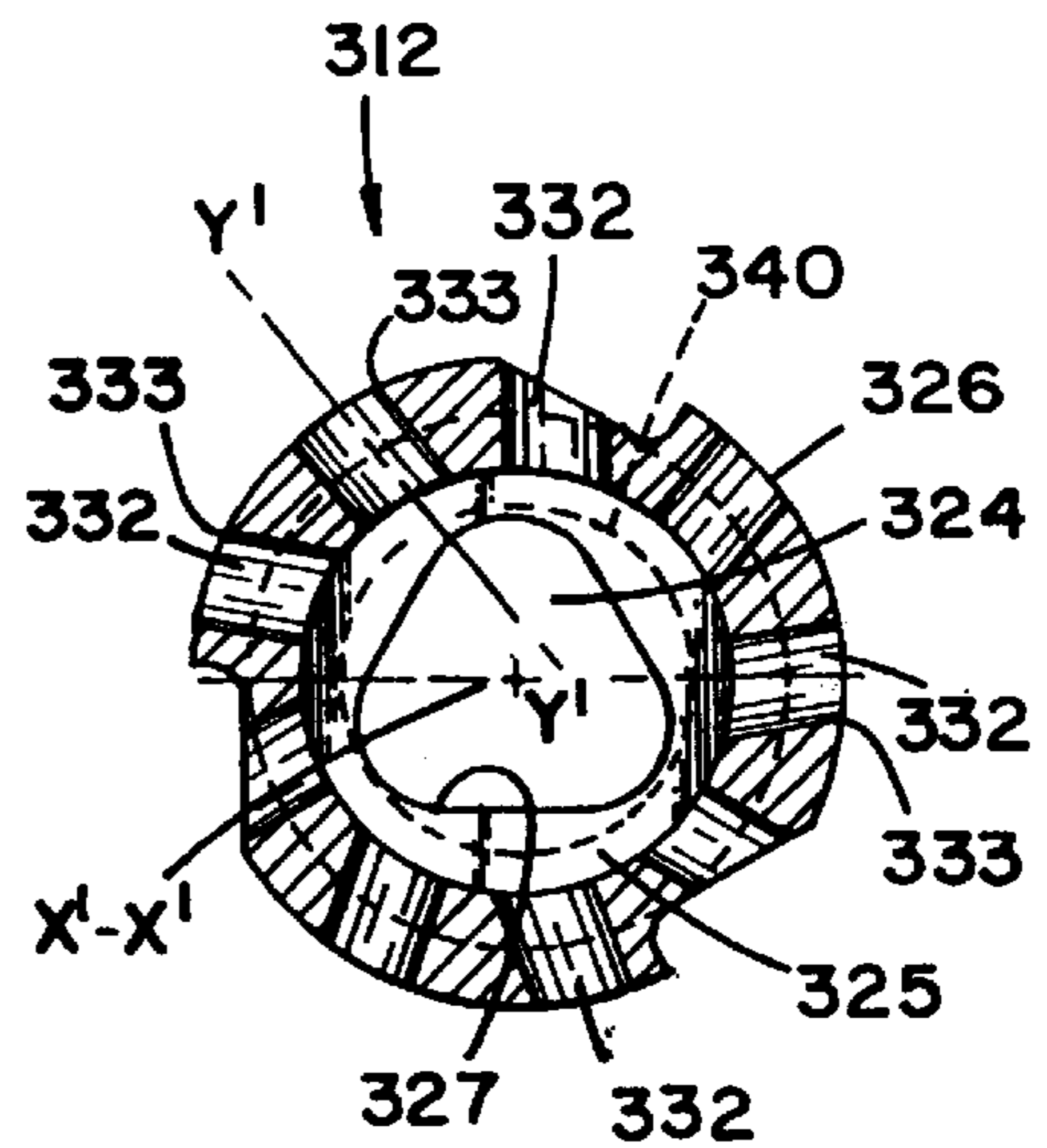
FIG. 27
