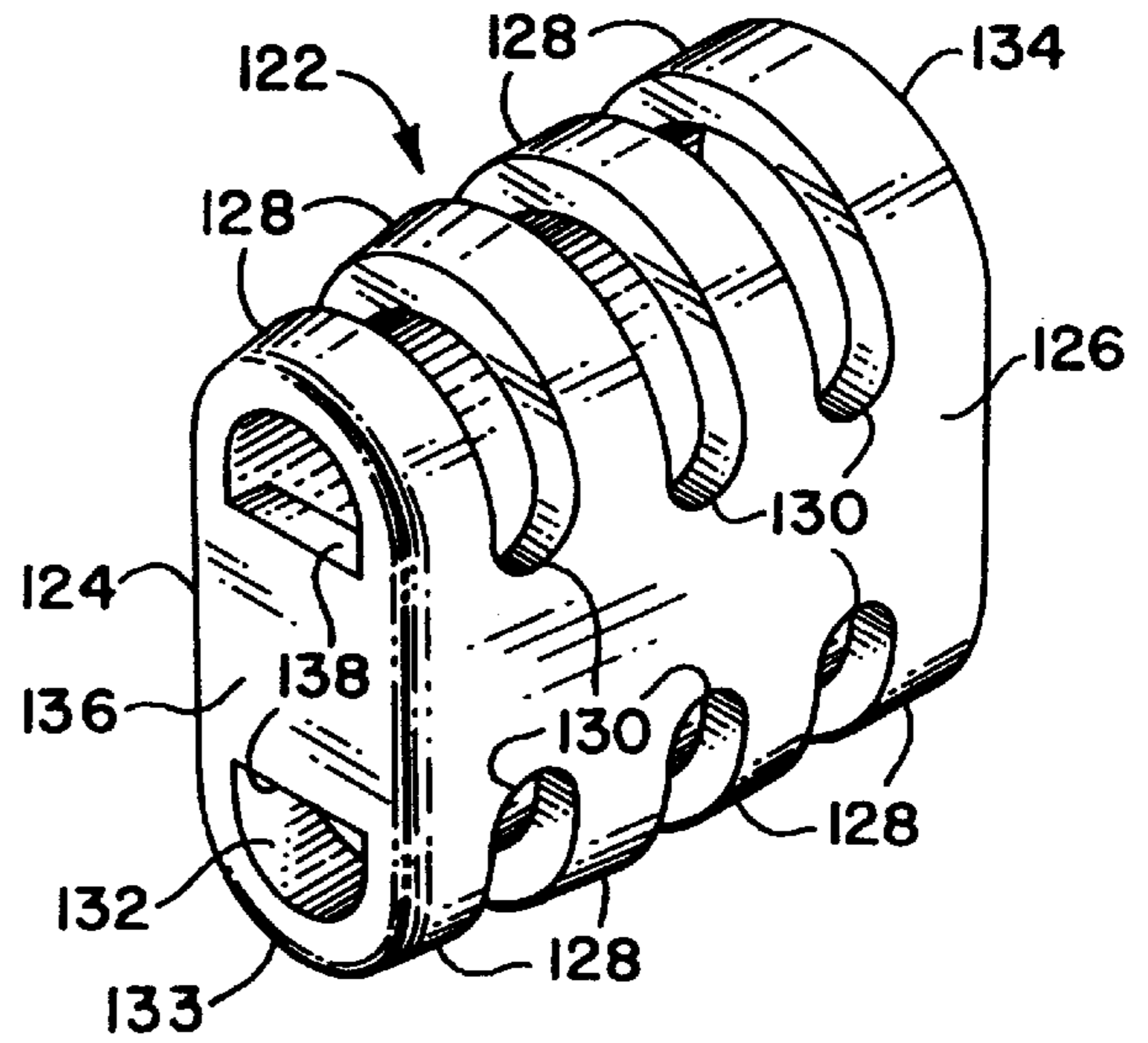
FIG. 15
