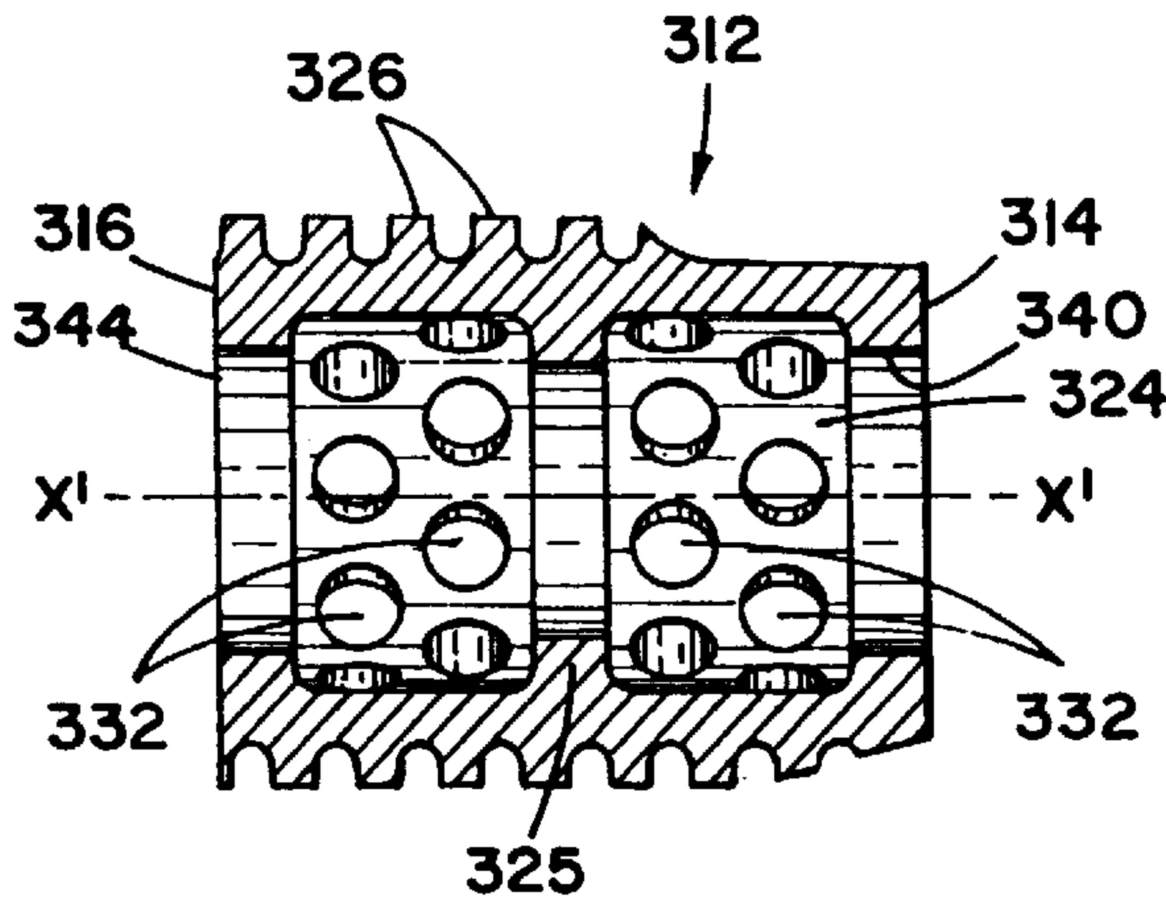
FIG. 26
