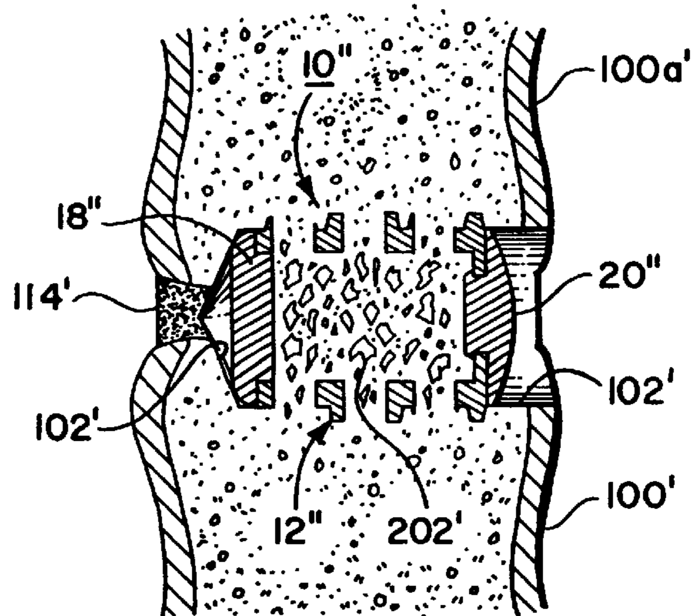
FIG. 13A
