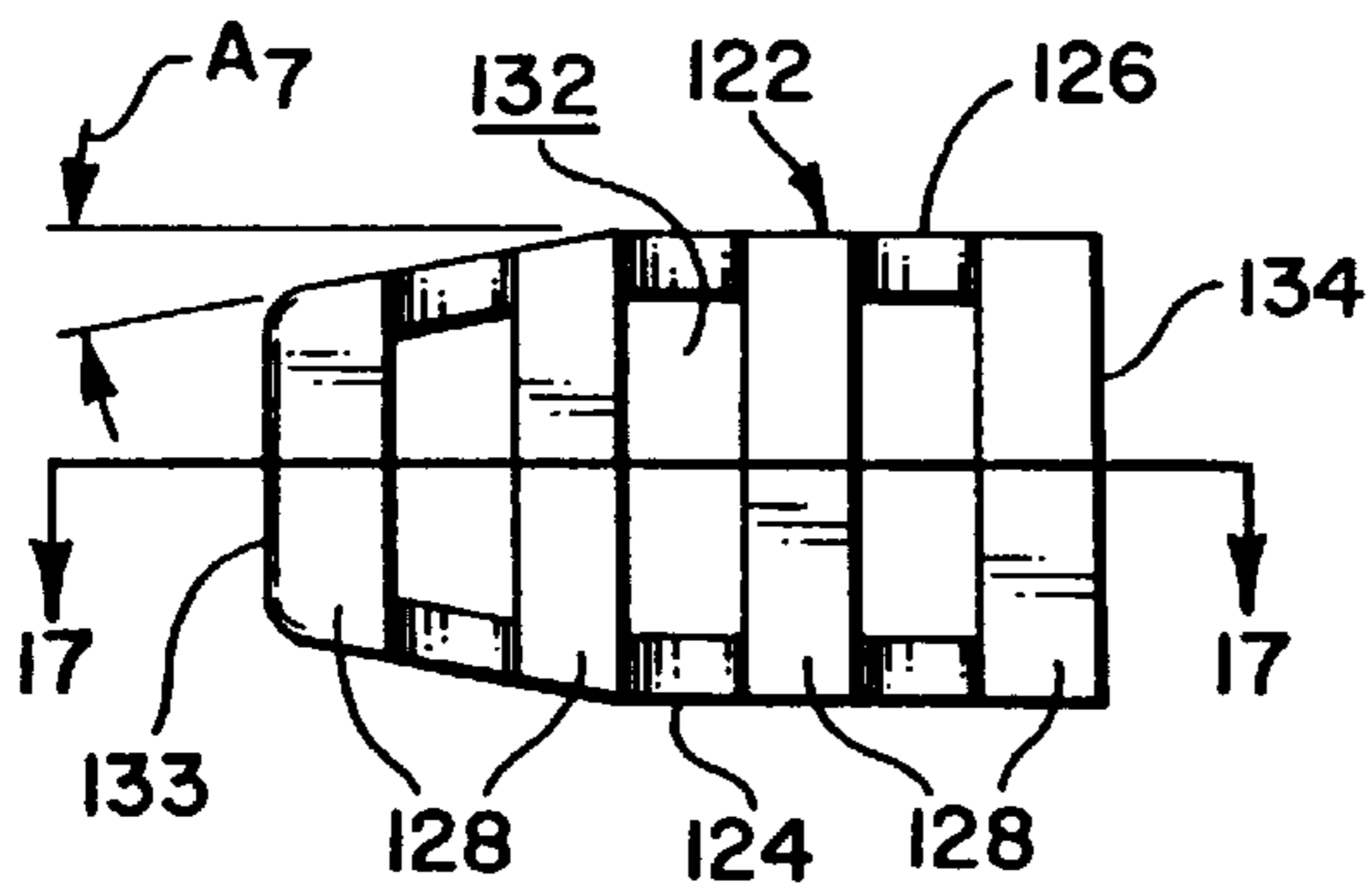
FIG. 16
