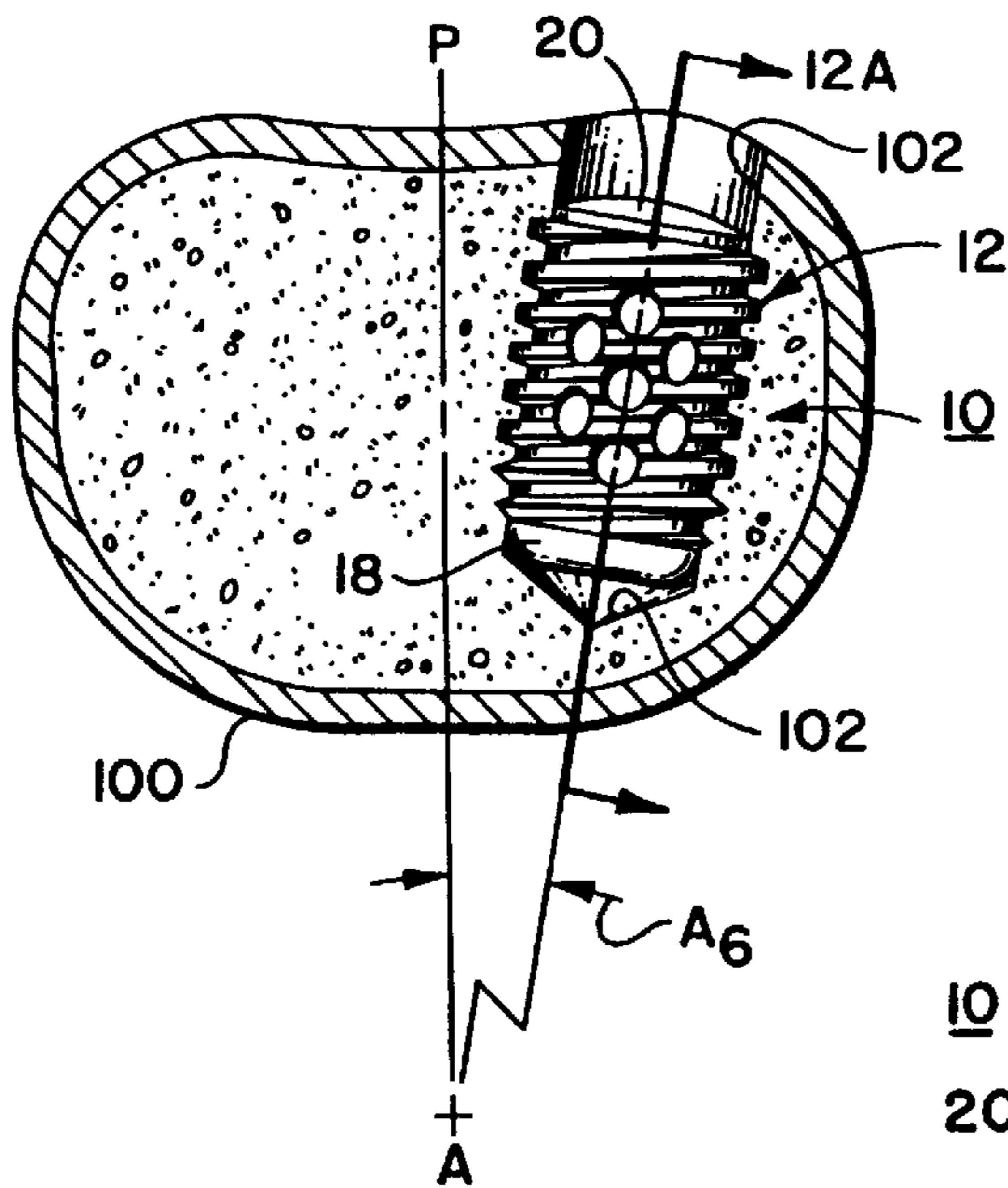
FIG. 12
