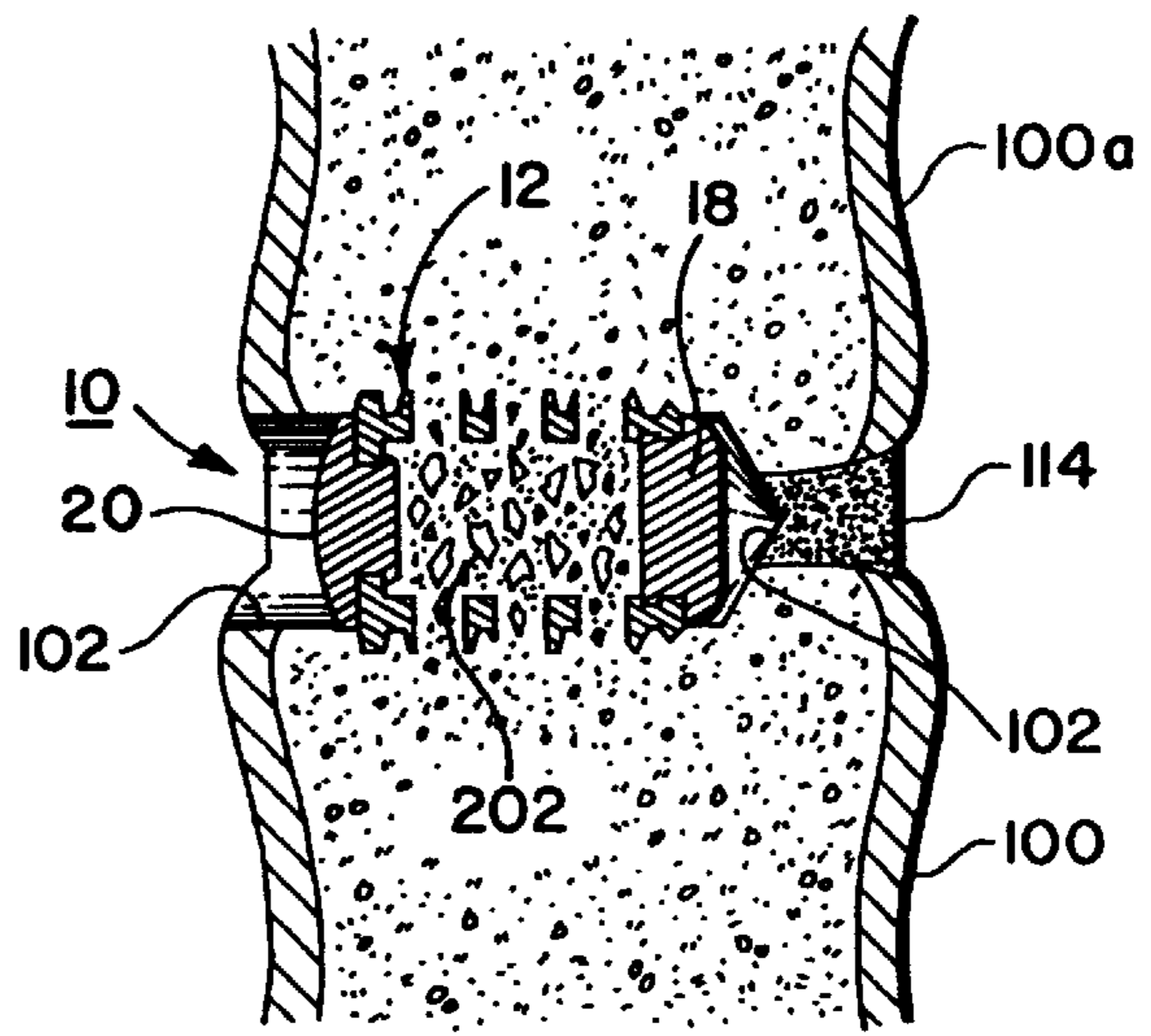
FIG. 12A
