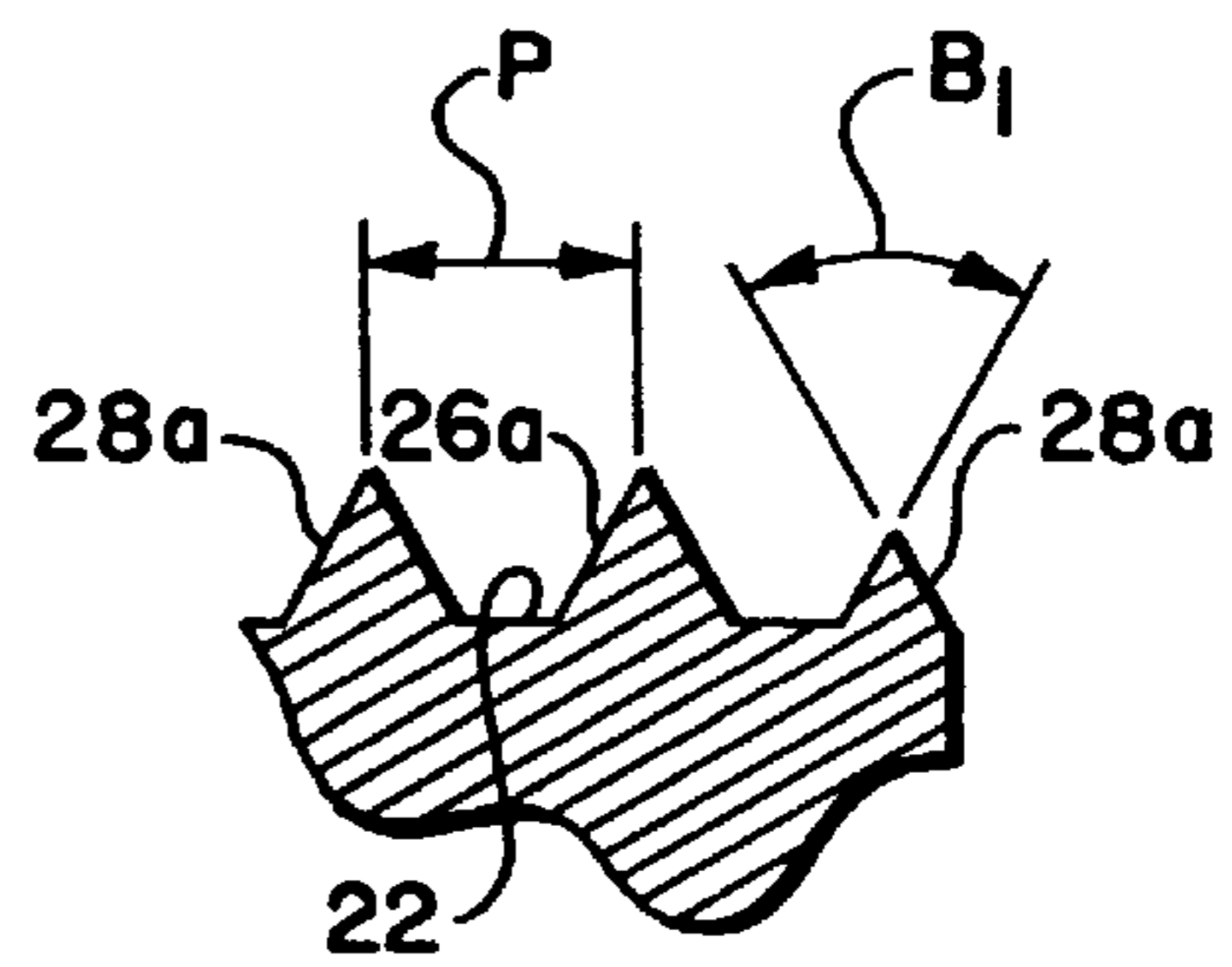
FIG. 7A
