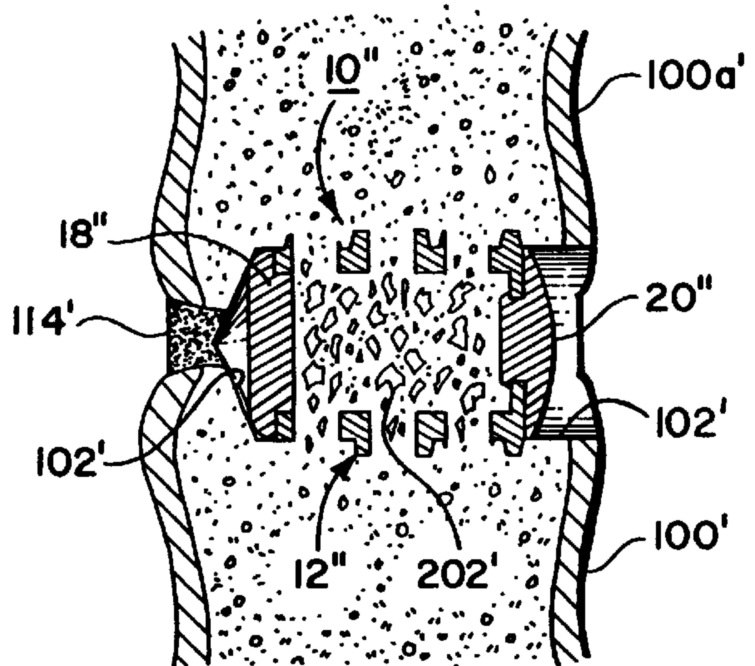
FIG. 13A
