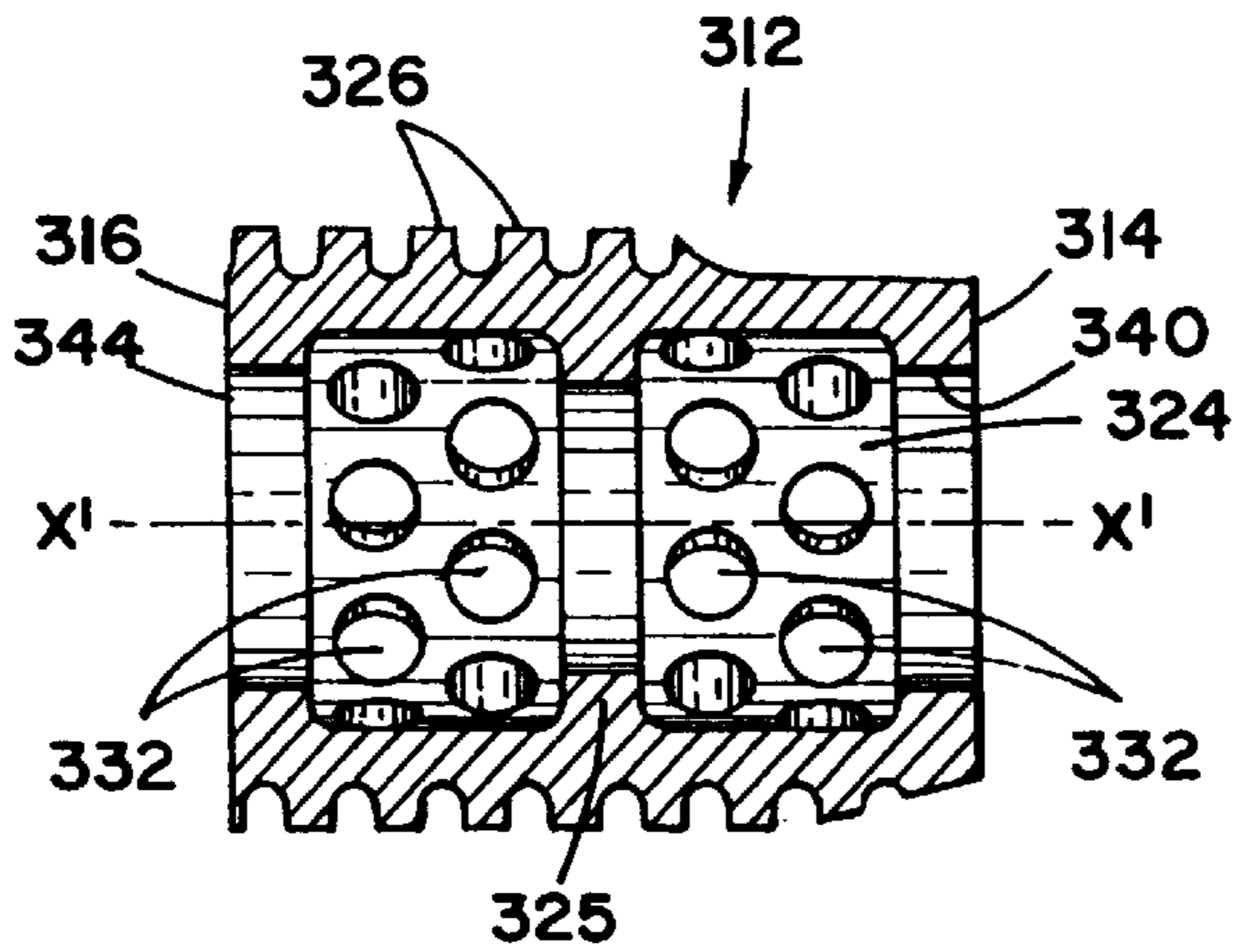
FIG. 26
