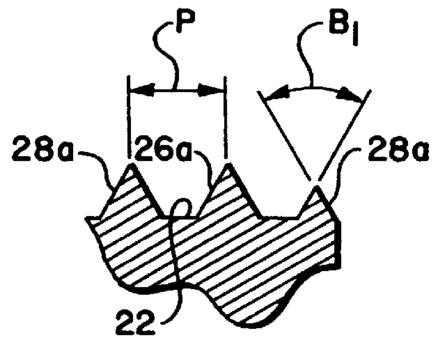
FIG. 7A
