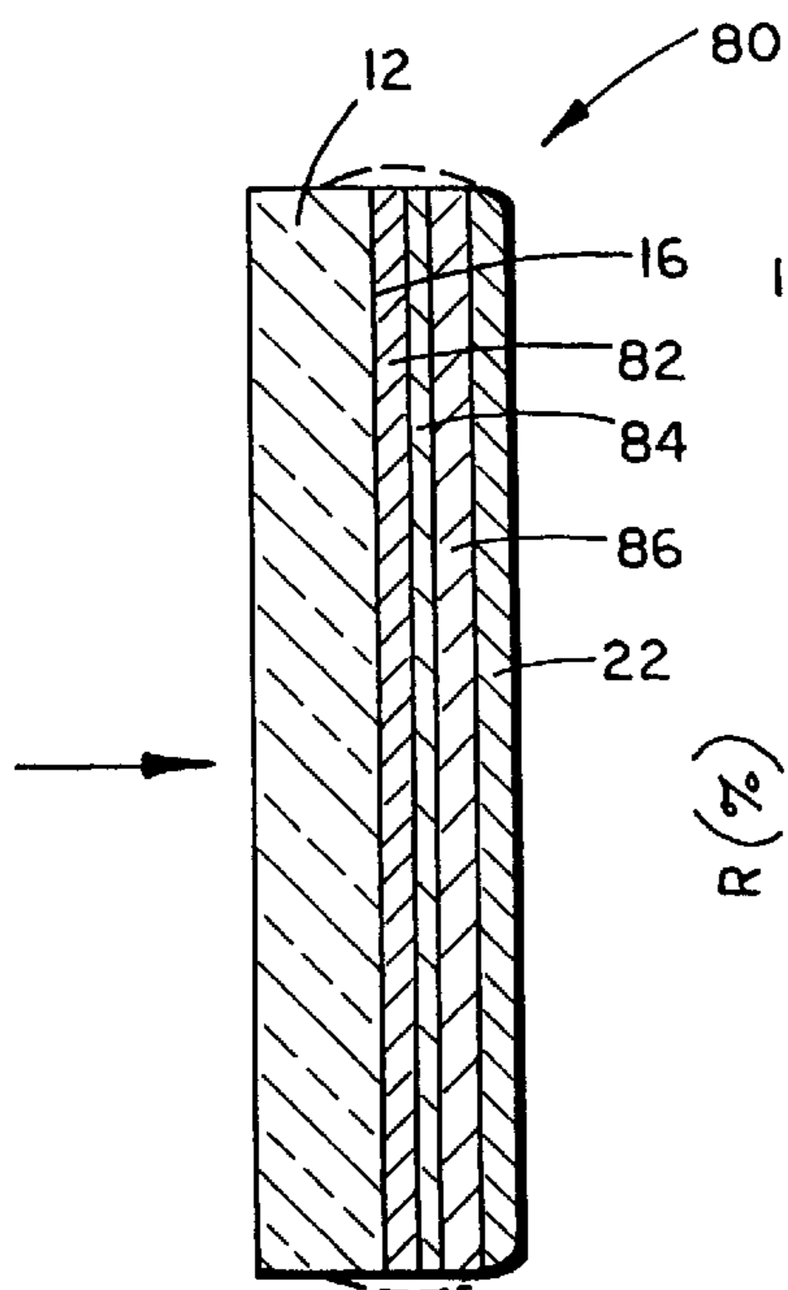
FIG. 16
