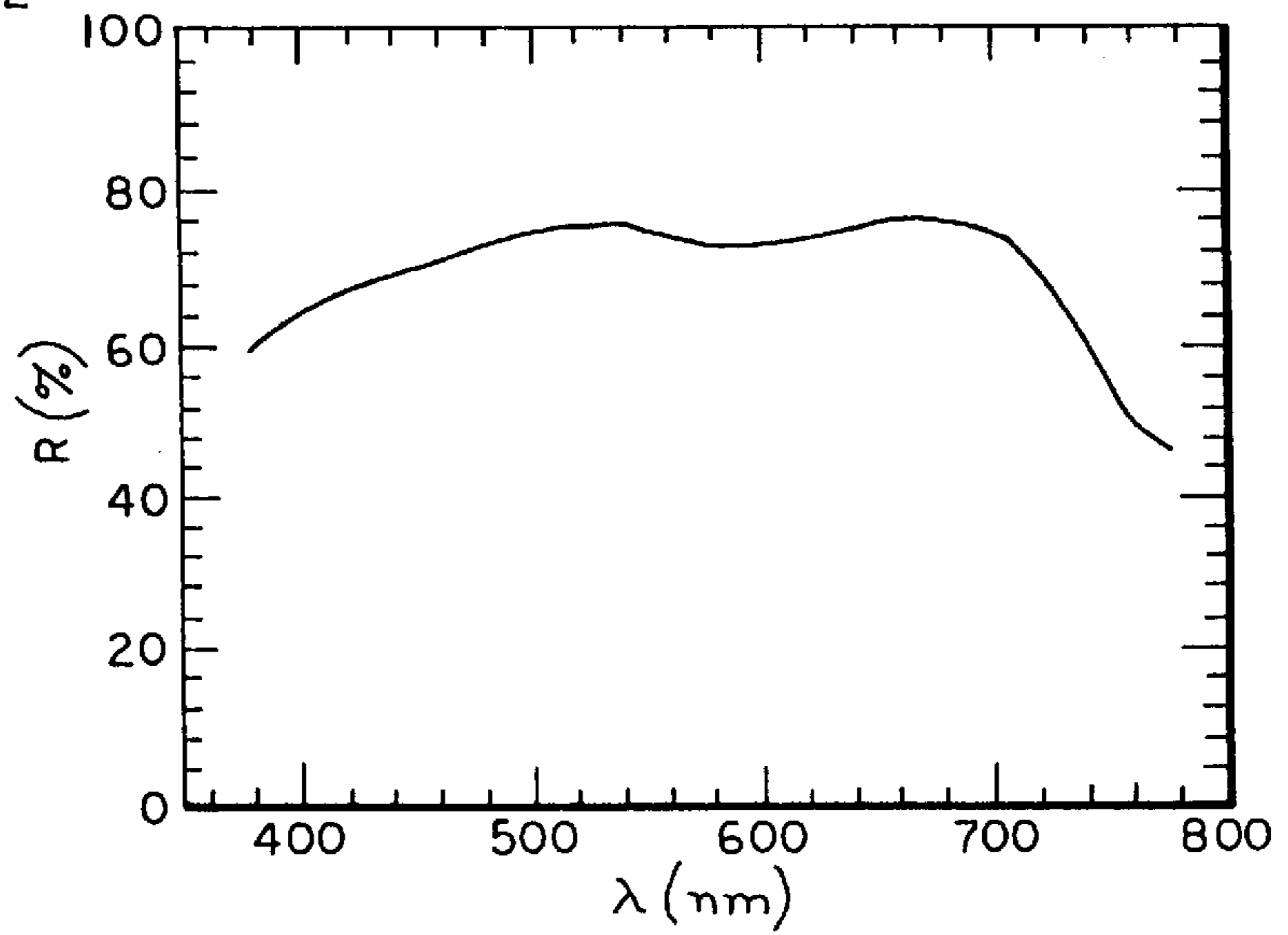
FIG. 9B
