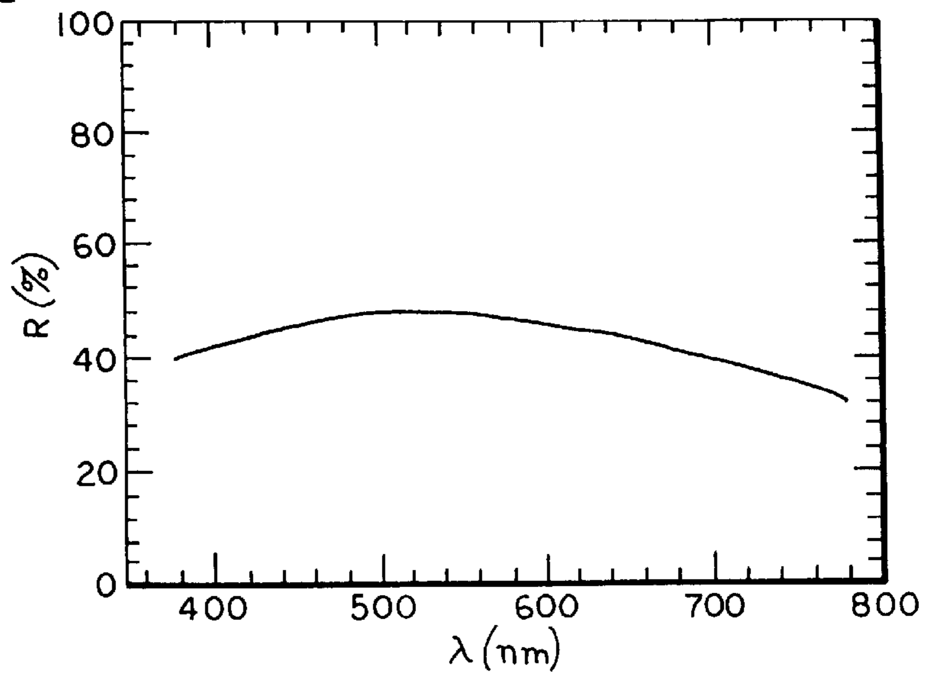
FIG.7
