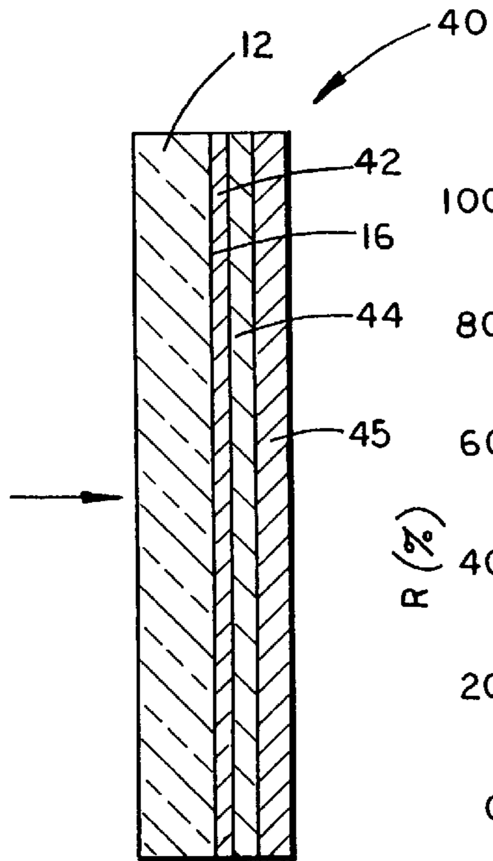
FIG. 8
