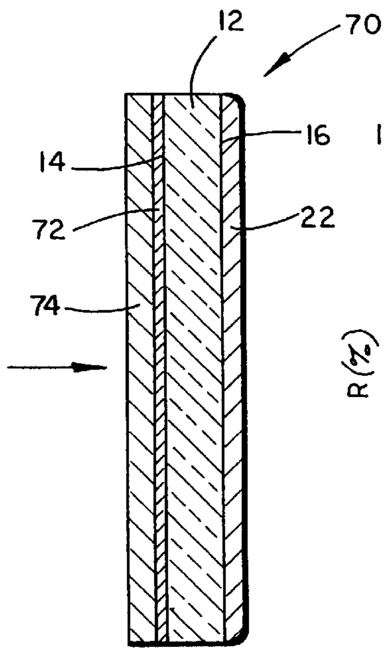
FIG. 14
