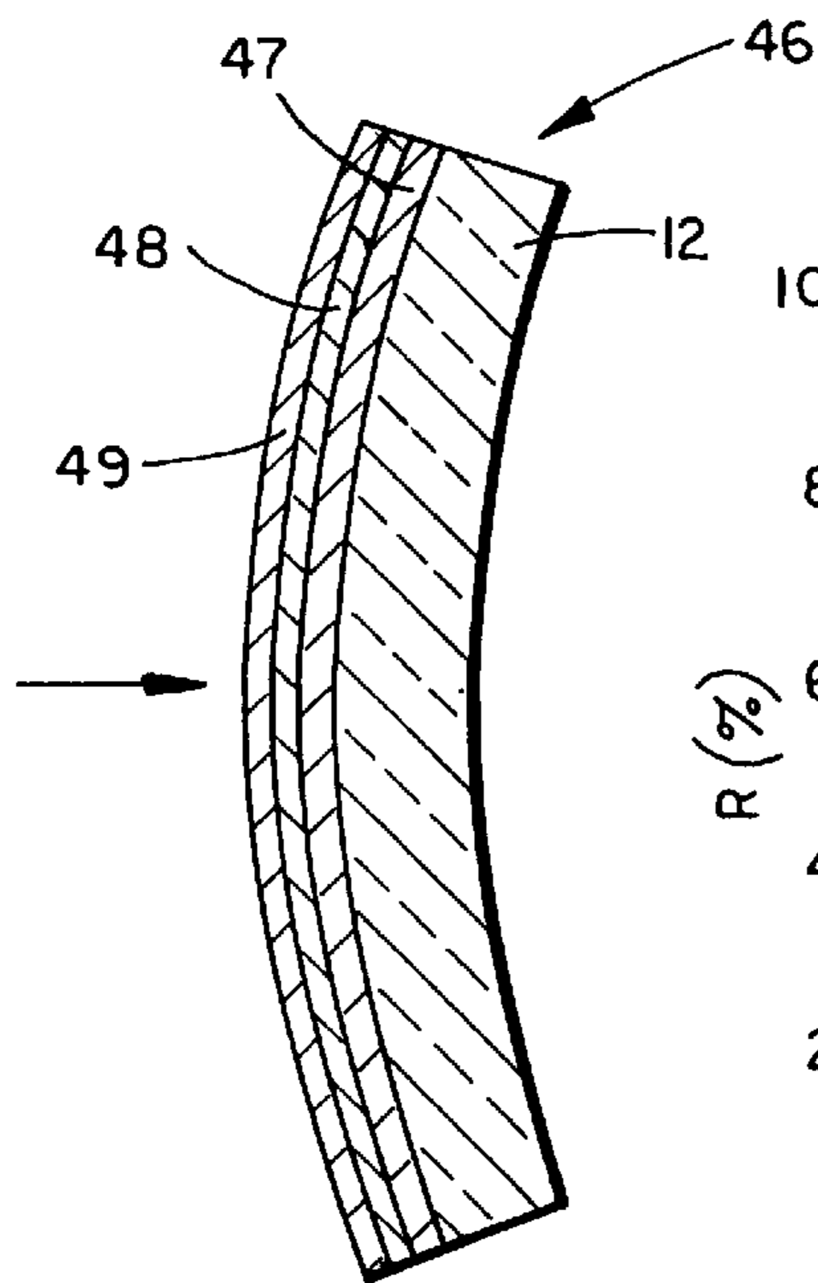
FIG. 9A
