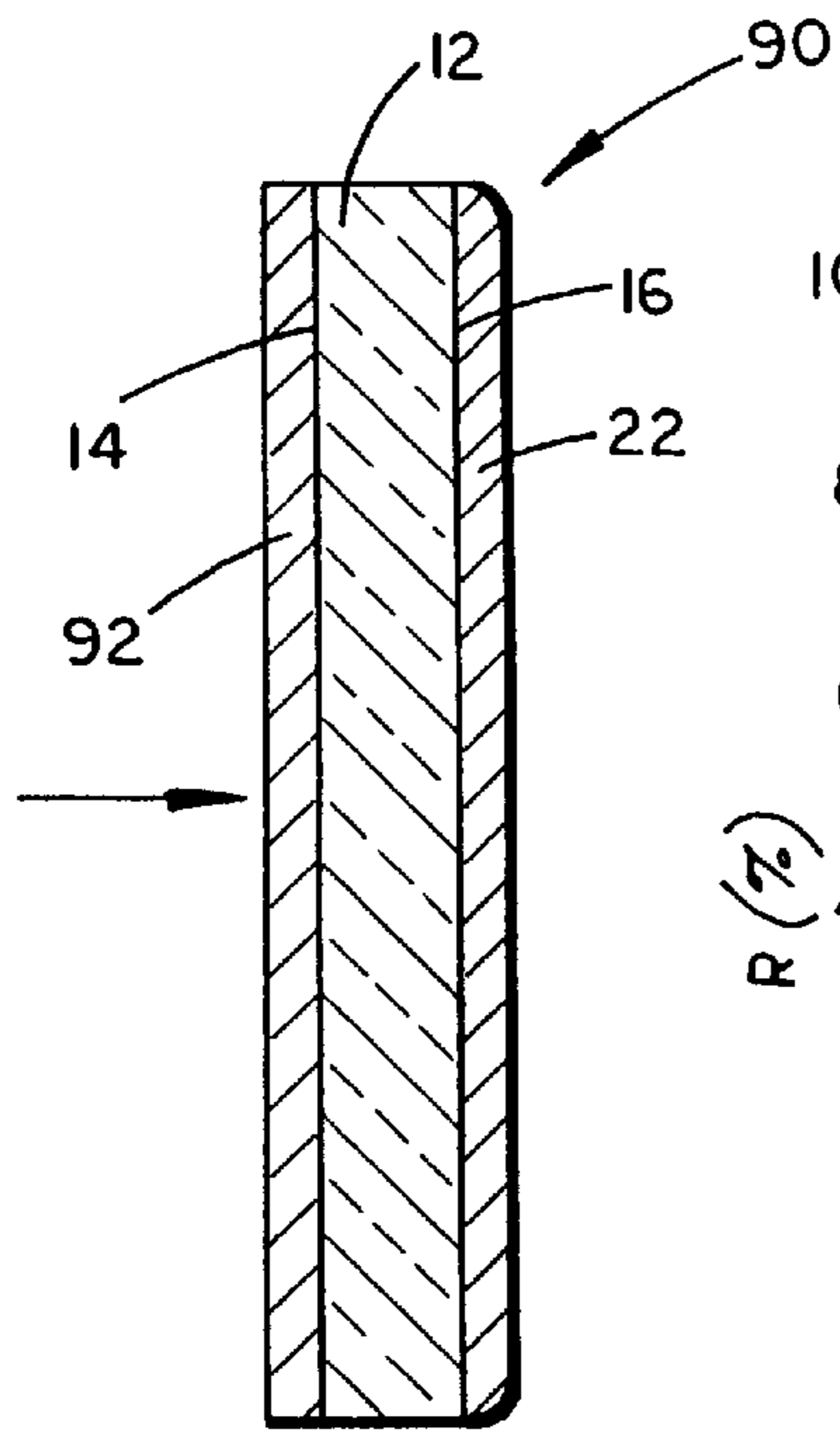
FIG. 18
