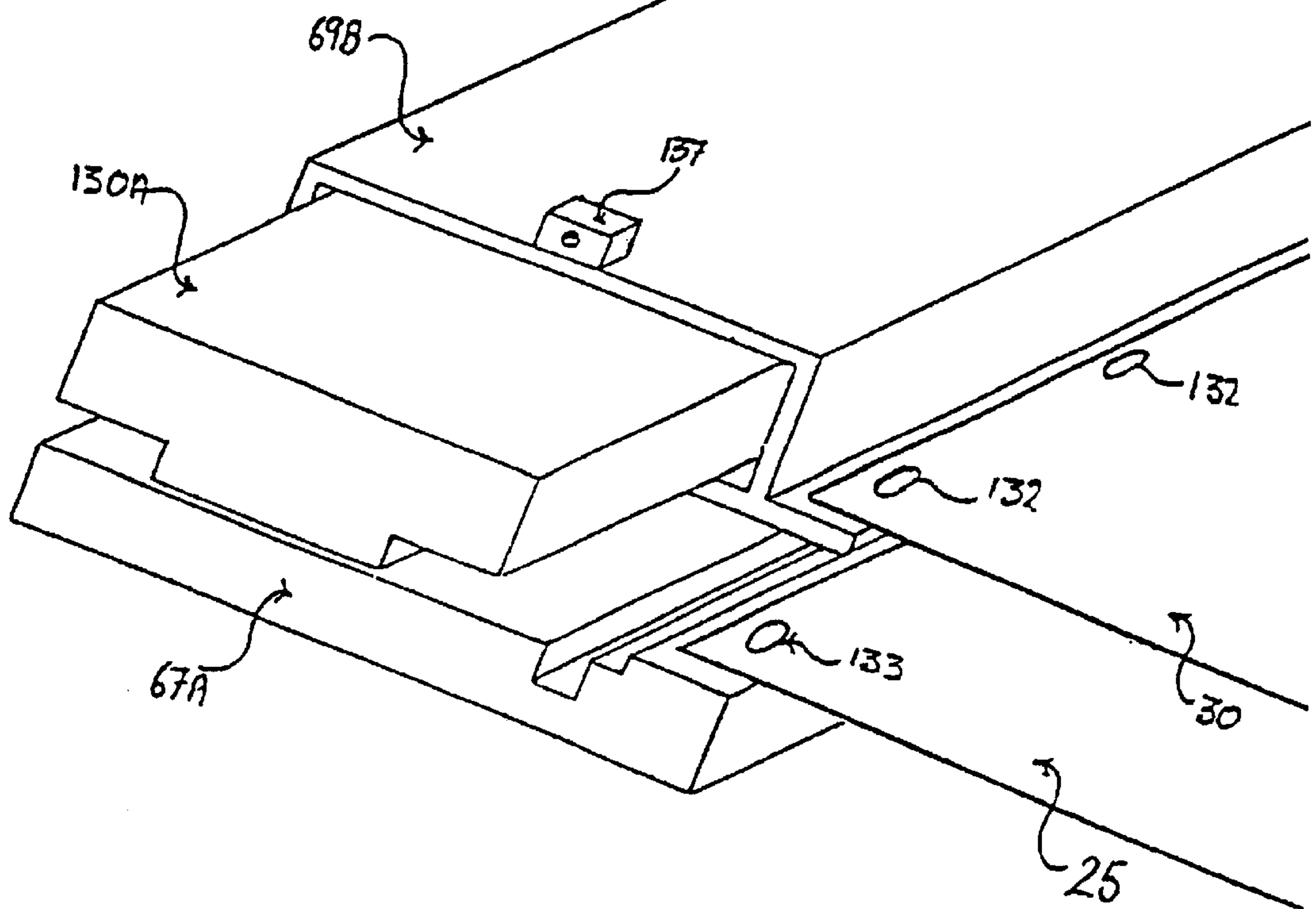
FIG. 14B
