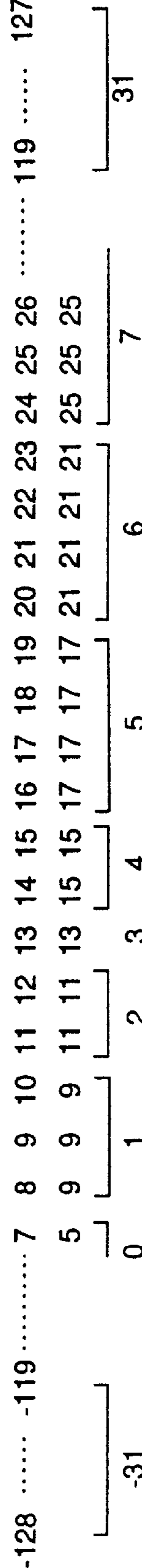
Fig.32 (d) quantization
