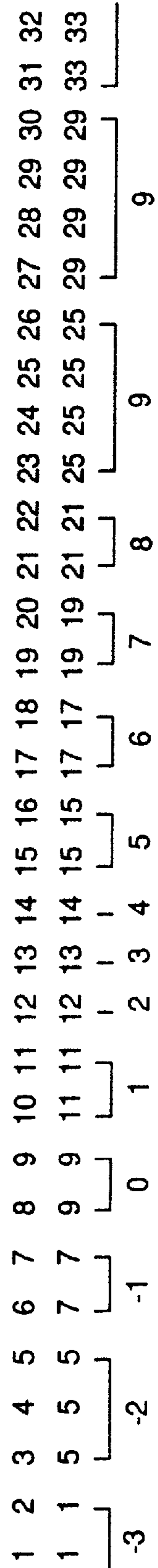
Fig.23 (d) quantization
