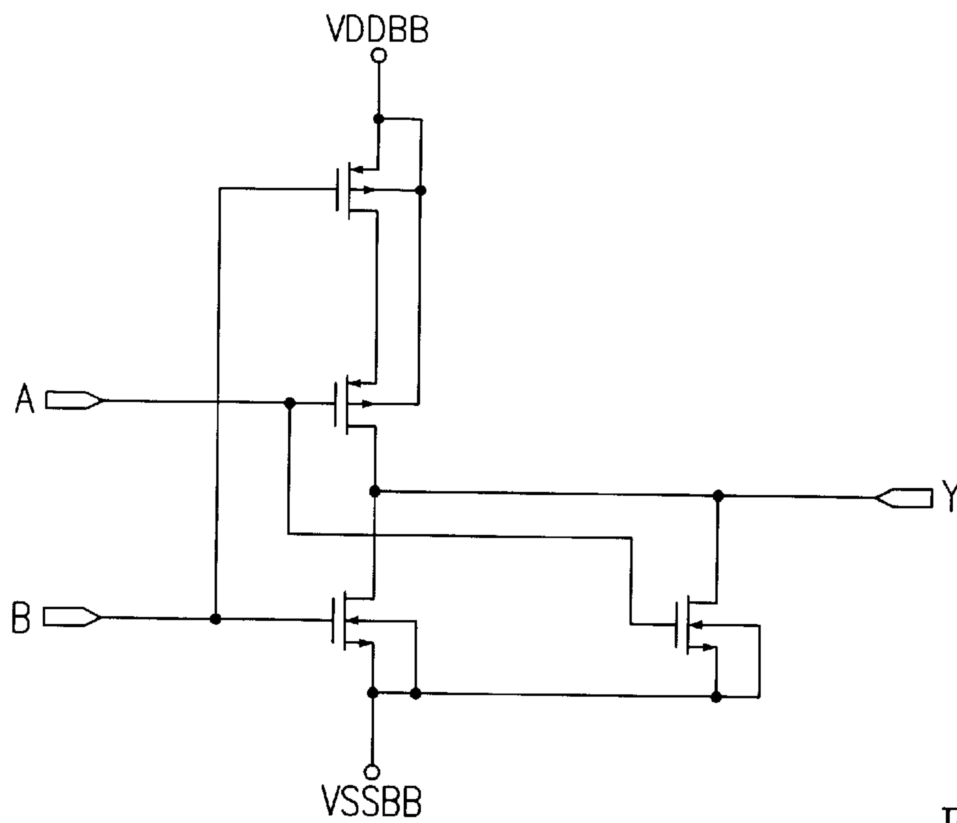
NOR2
