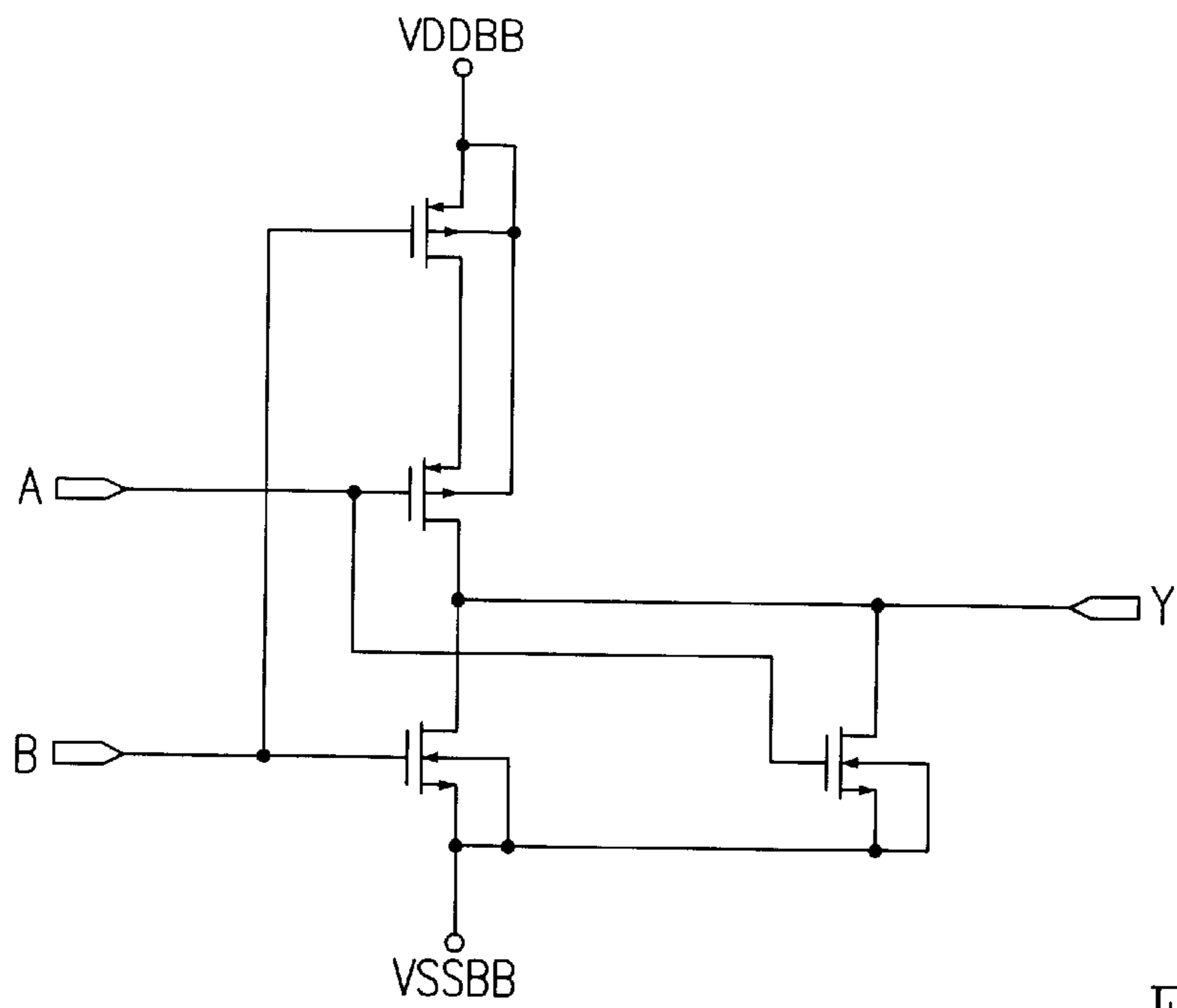
NOR2
