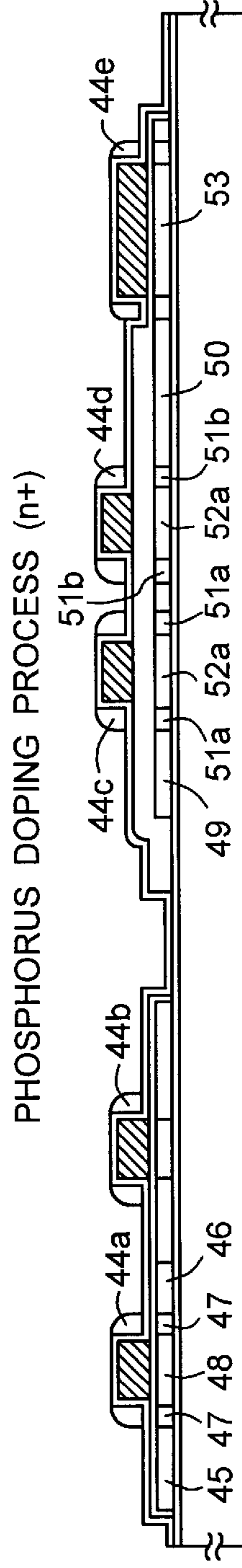
FIG. 12C
