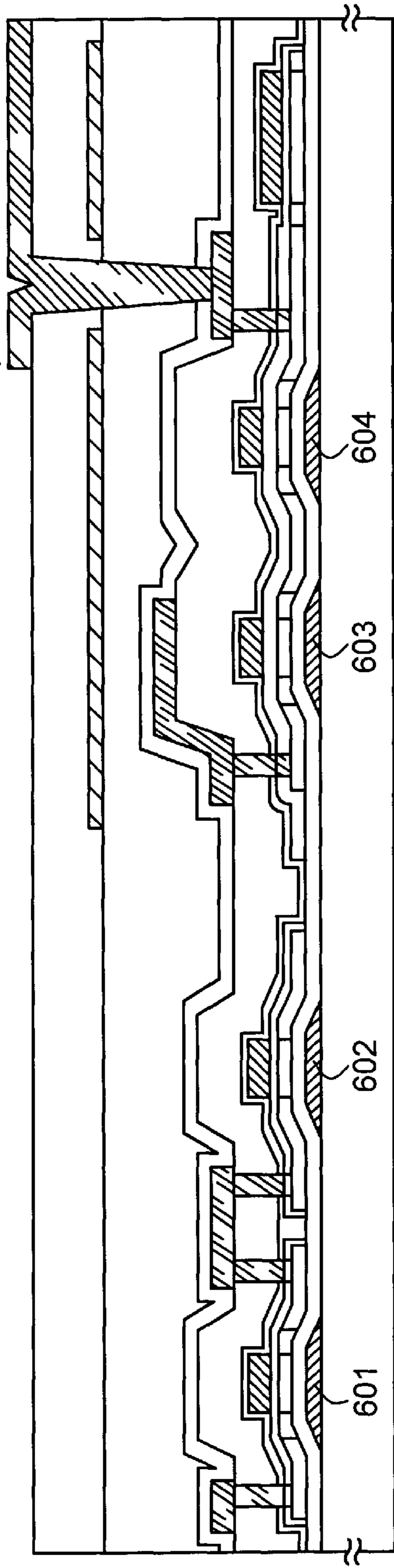
FIG. 6A
