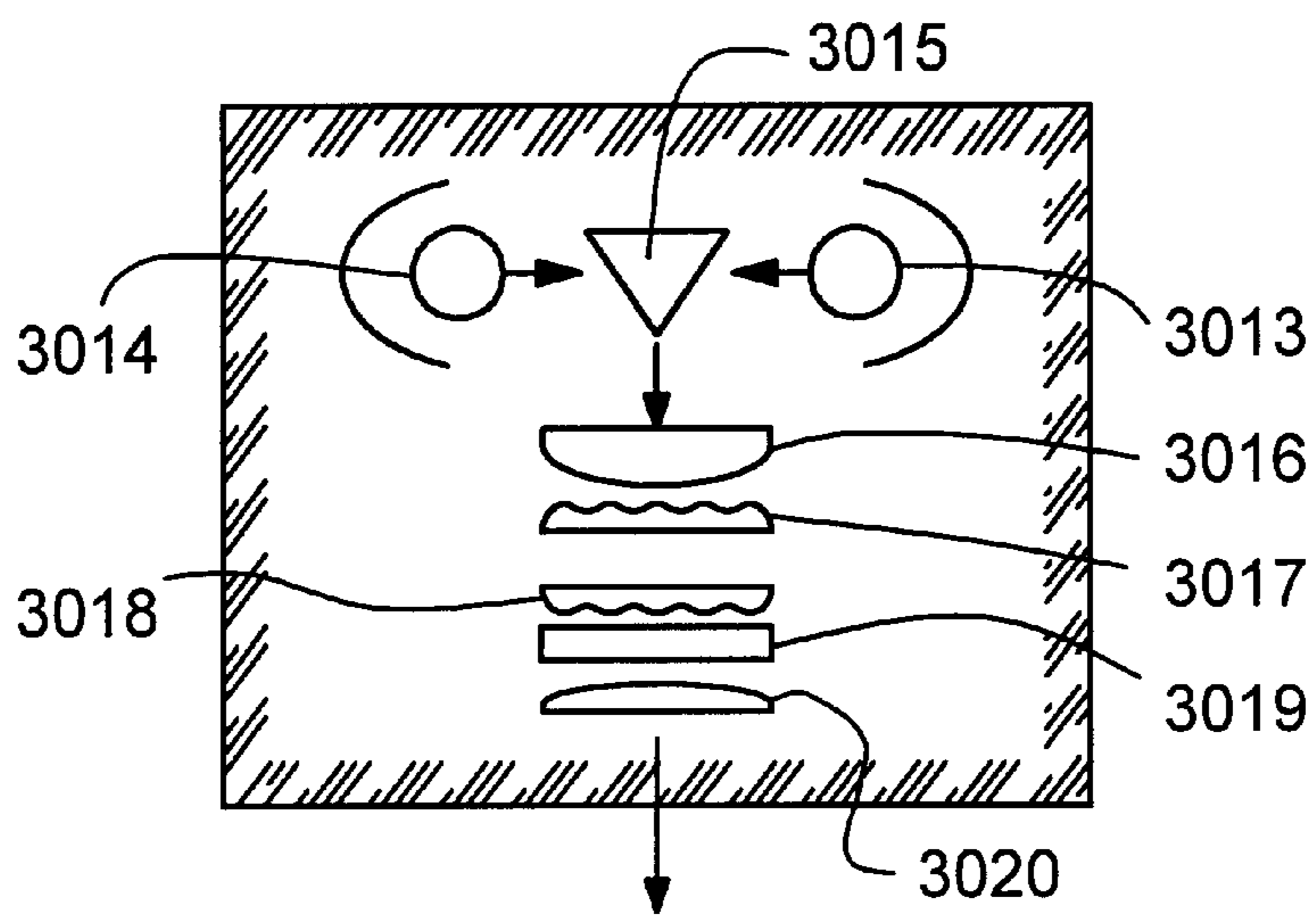
FIG. 23B
