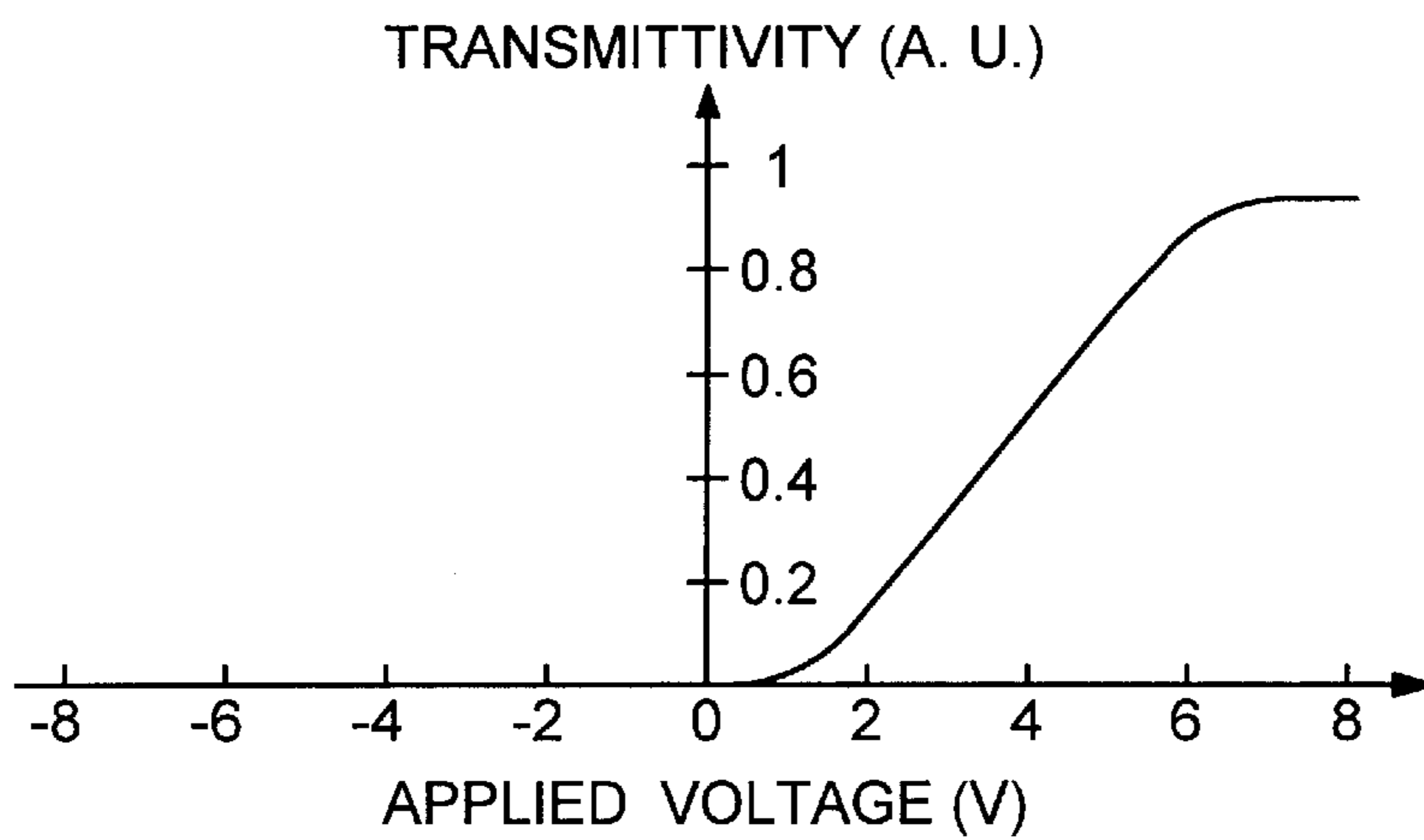
FIG. 20
