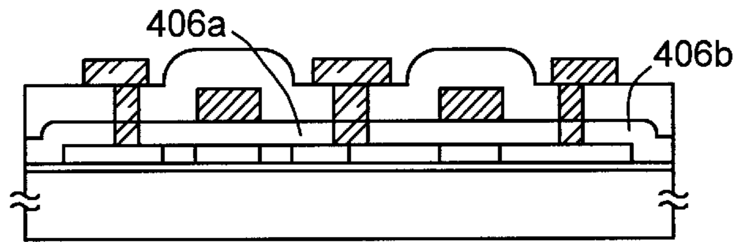
FIG. 4C
