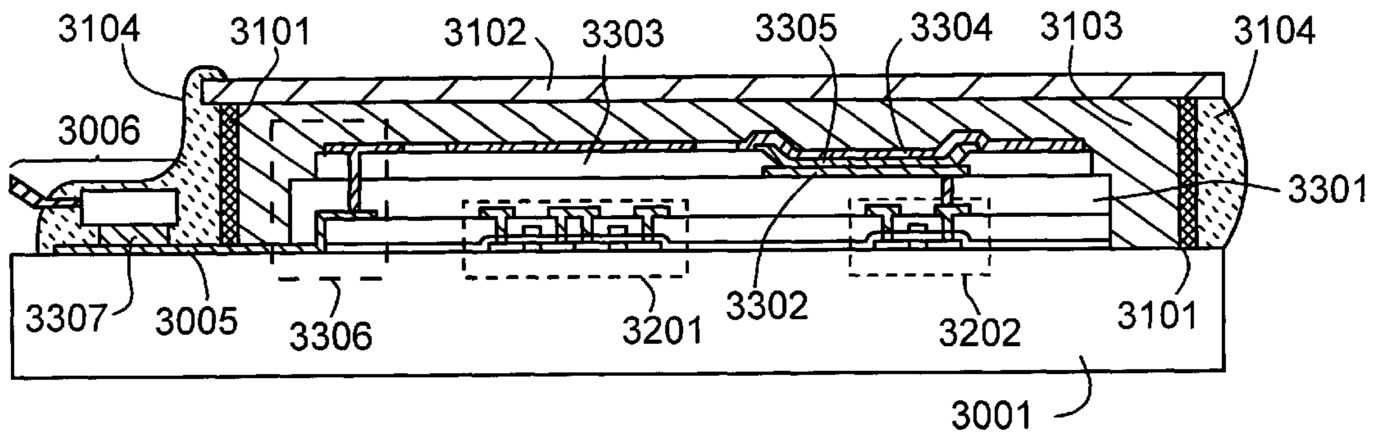
FIG. 18B
