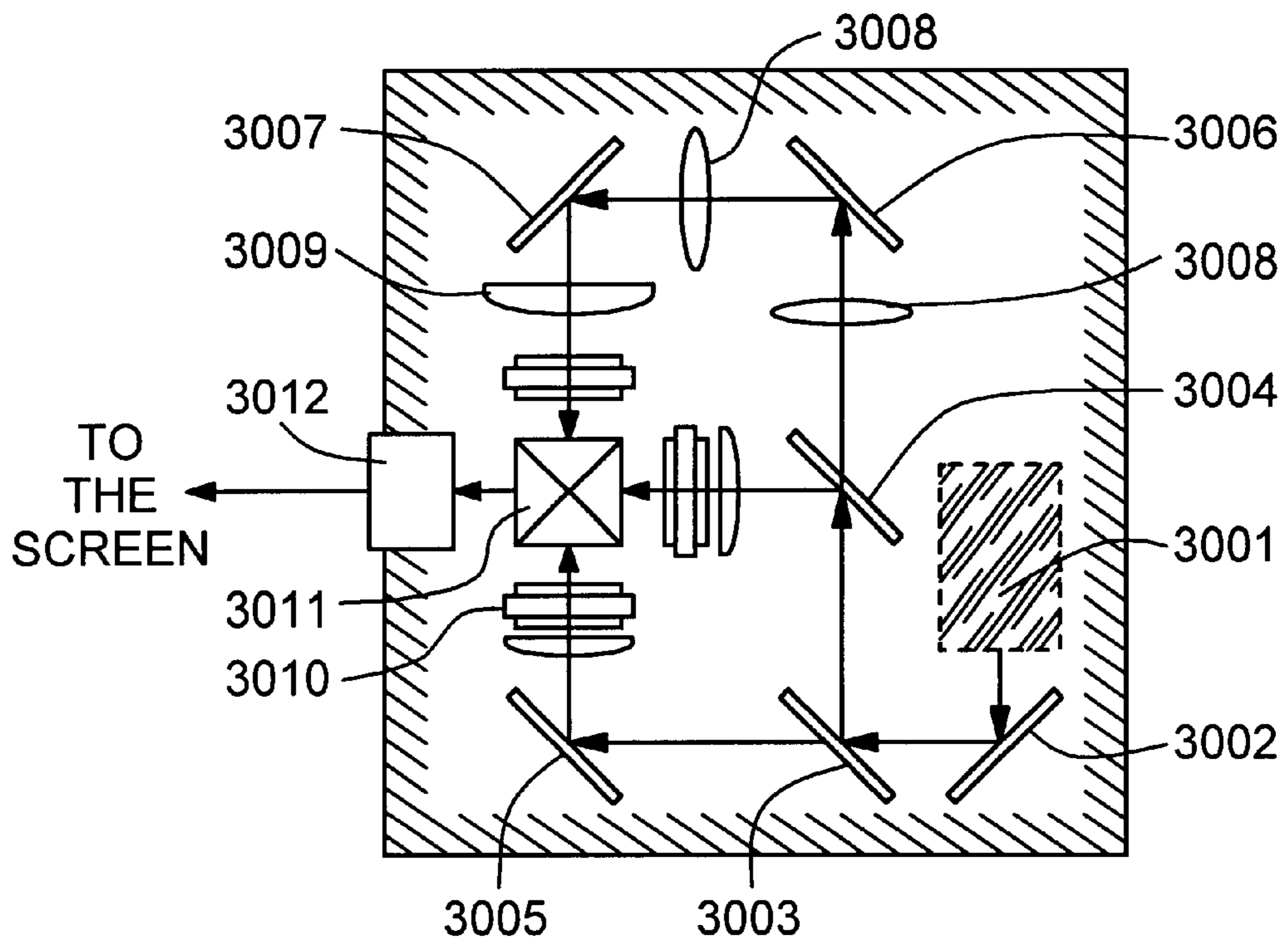
FIG. 23A
