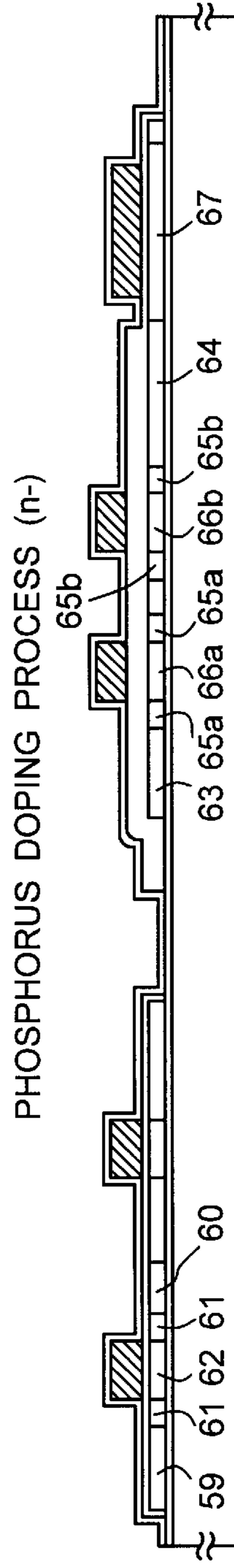
FIG. 13C
