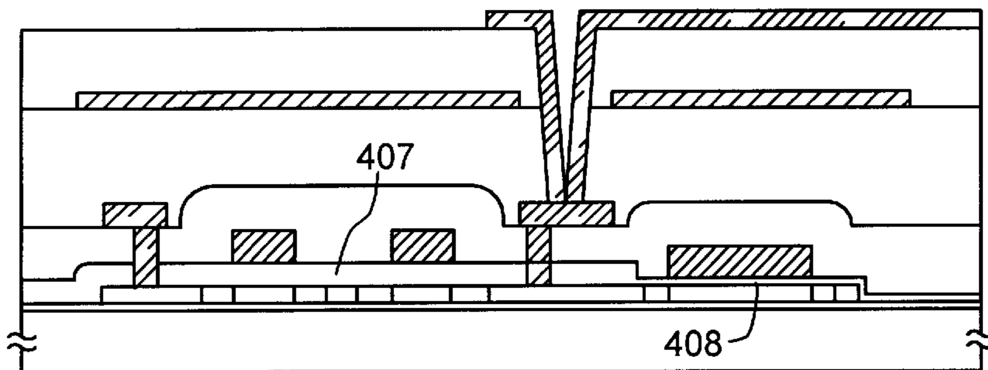
FIG. 4D
