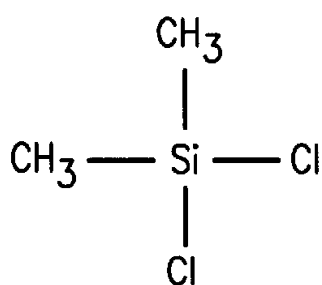
DMS
