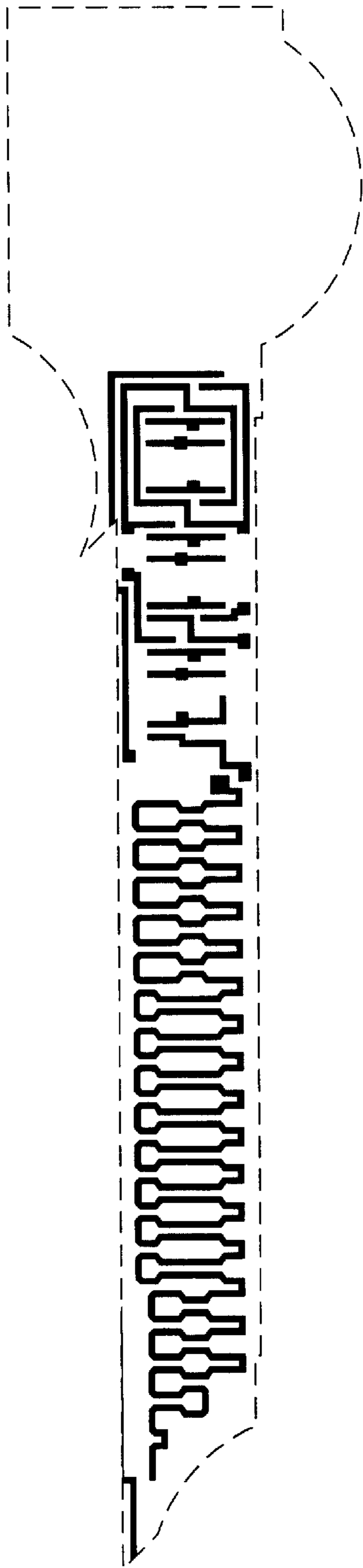
Poly mask
