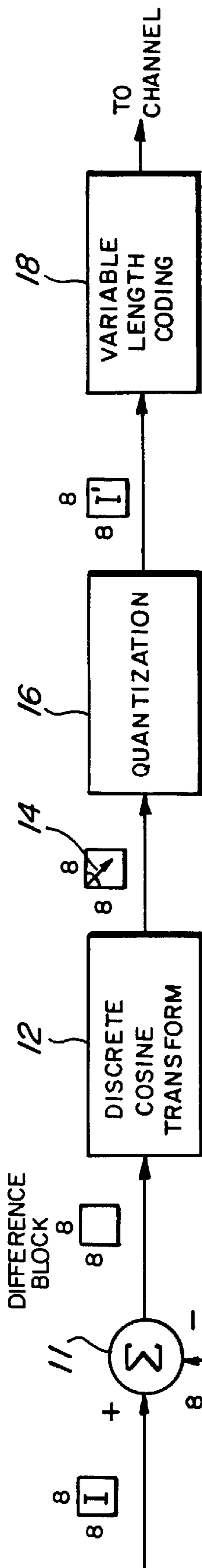
FIG. 2b
