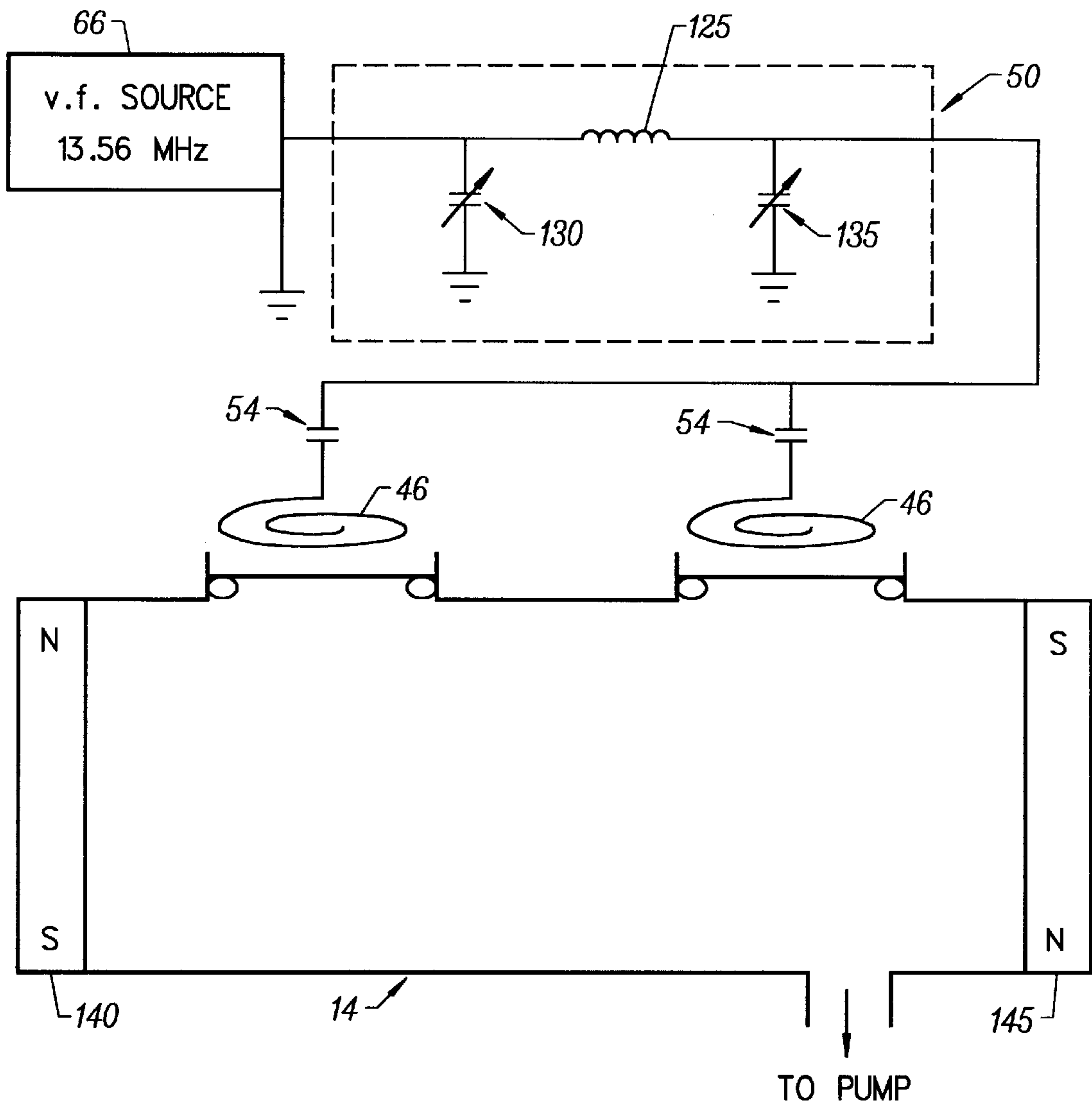
FIG. 8
