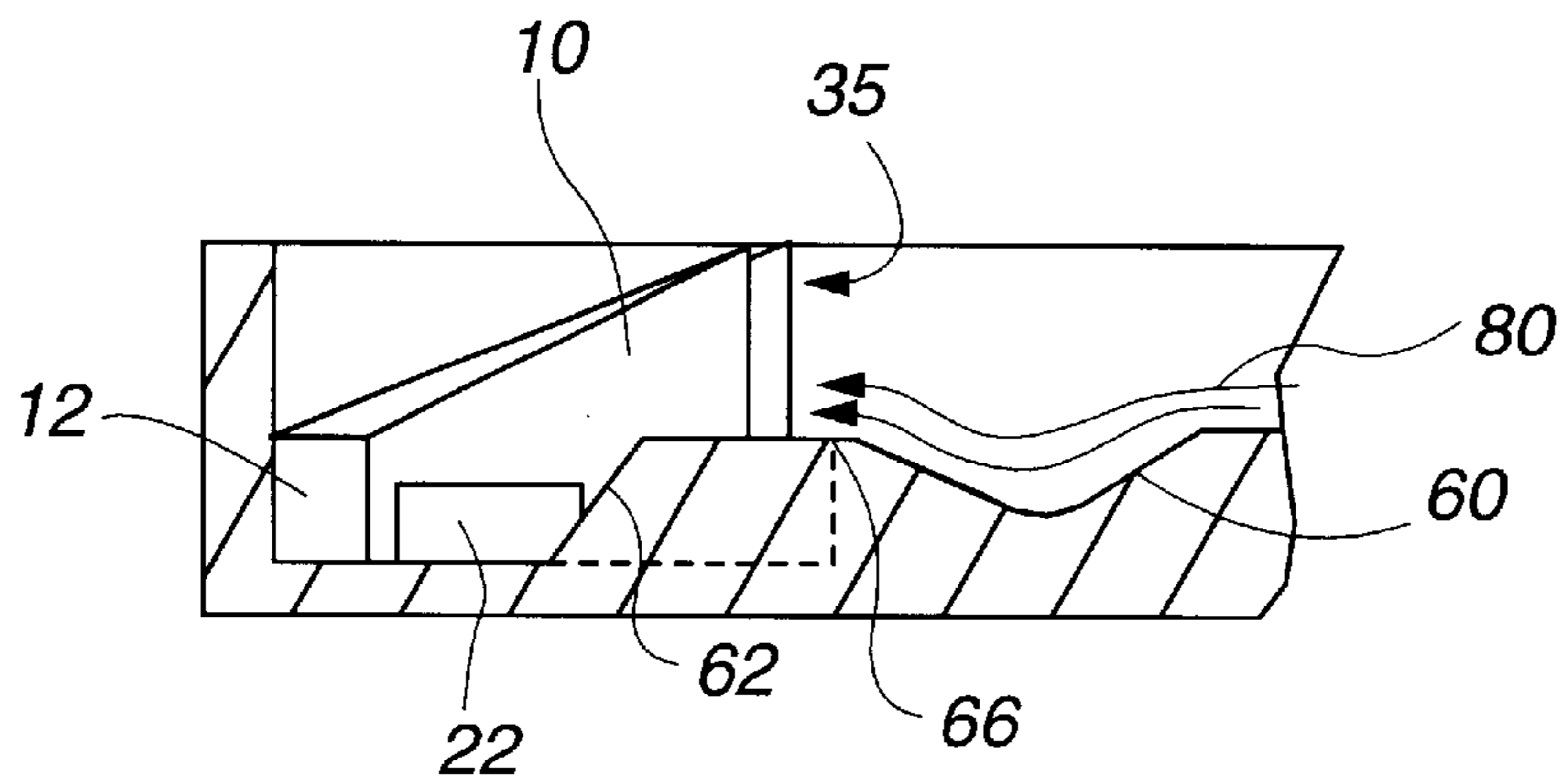
VIEW A-A
