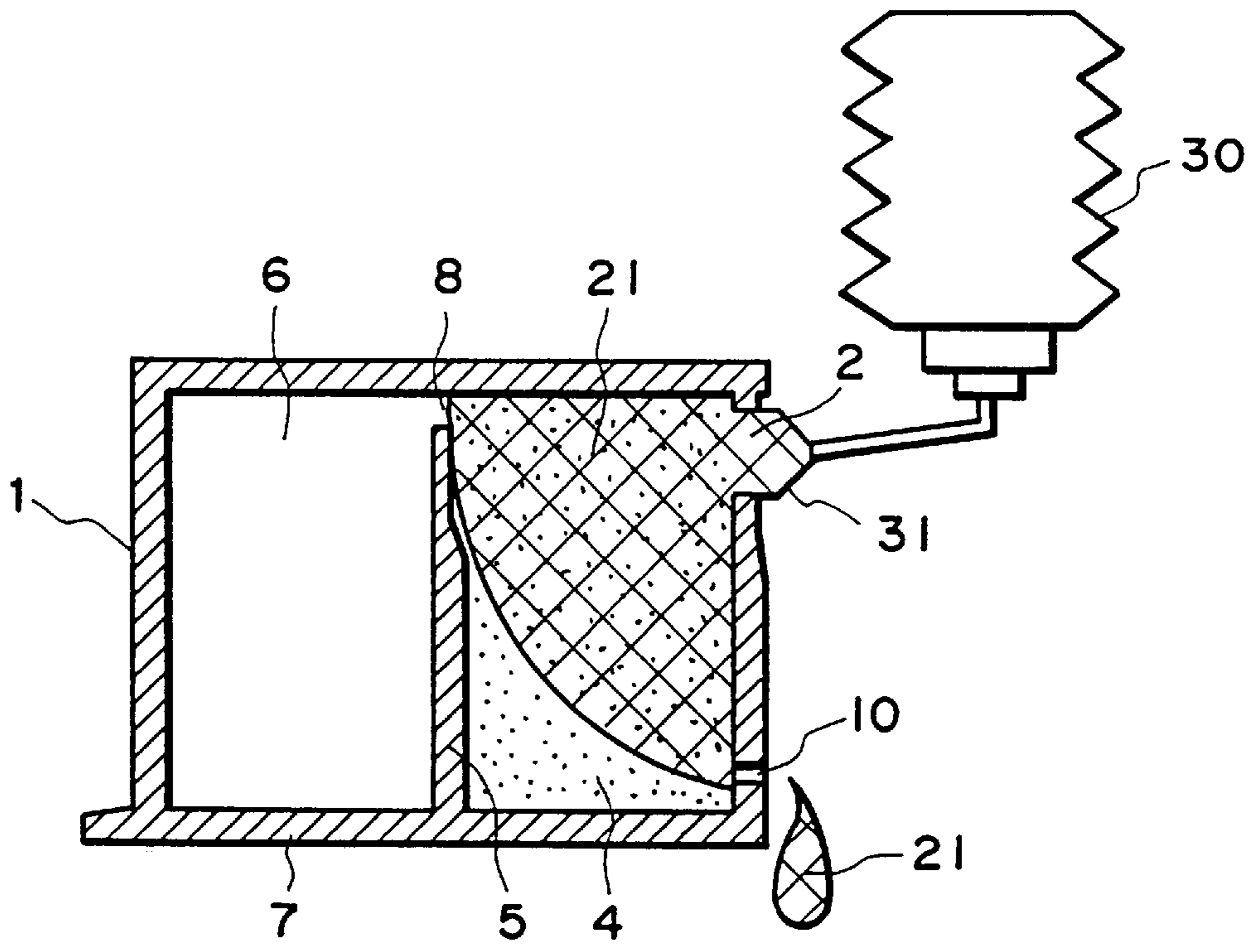
FIG. 13B
