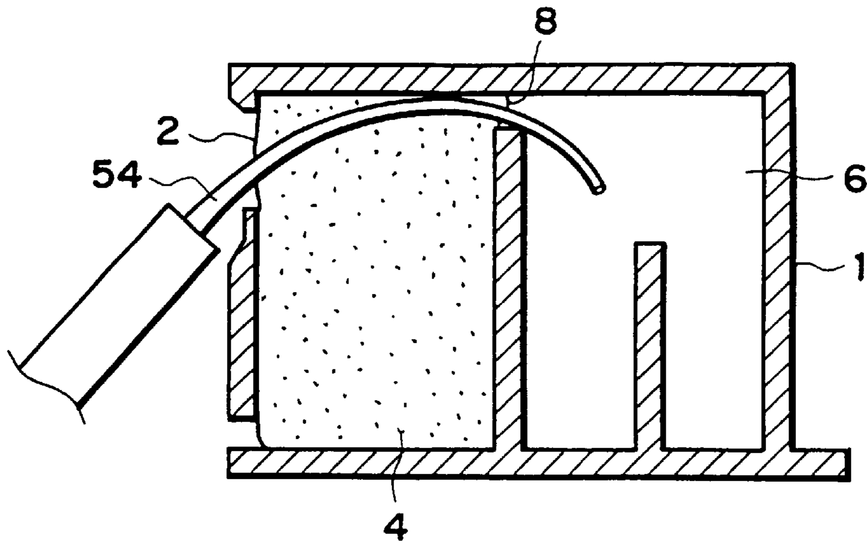
FIG. 31A
