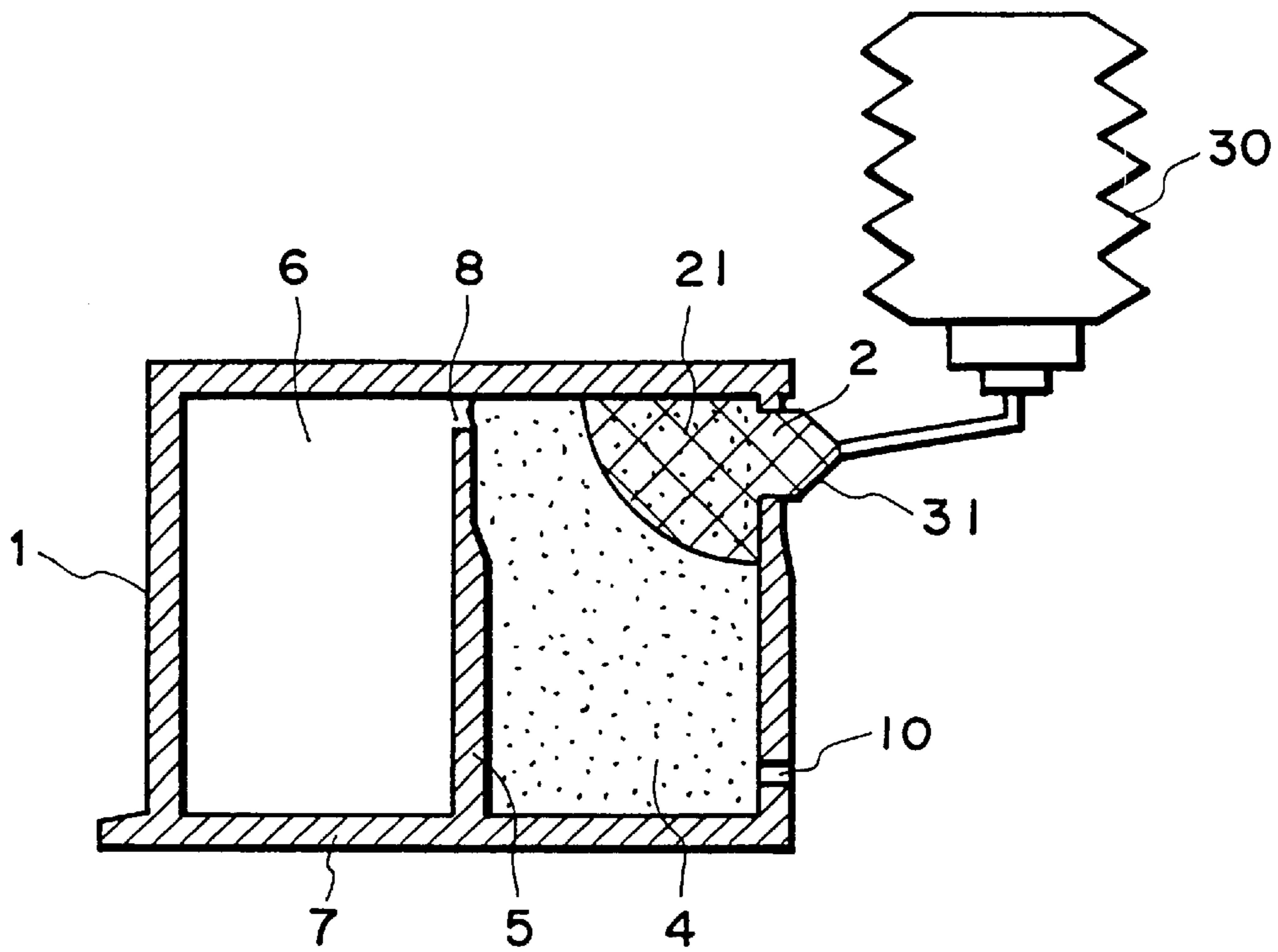
FIG. 13A
