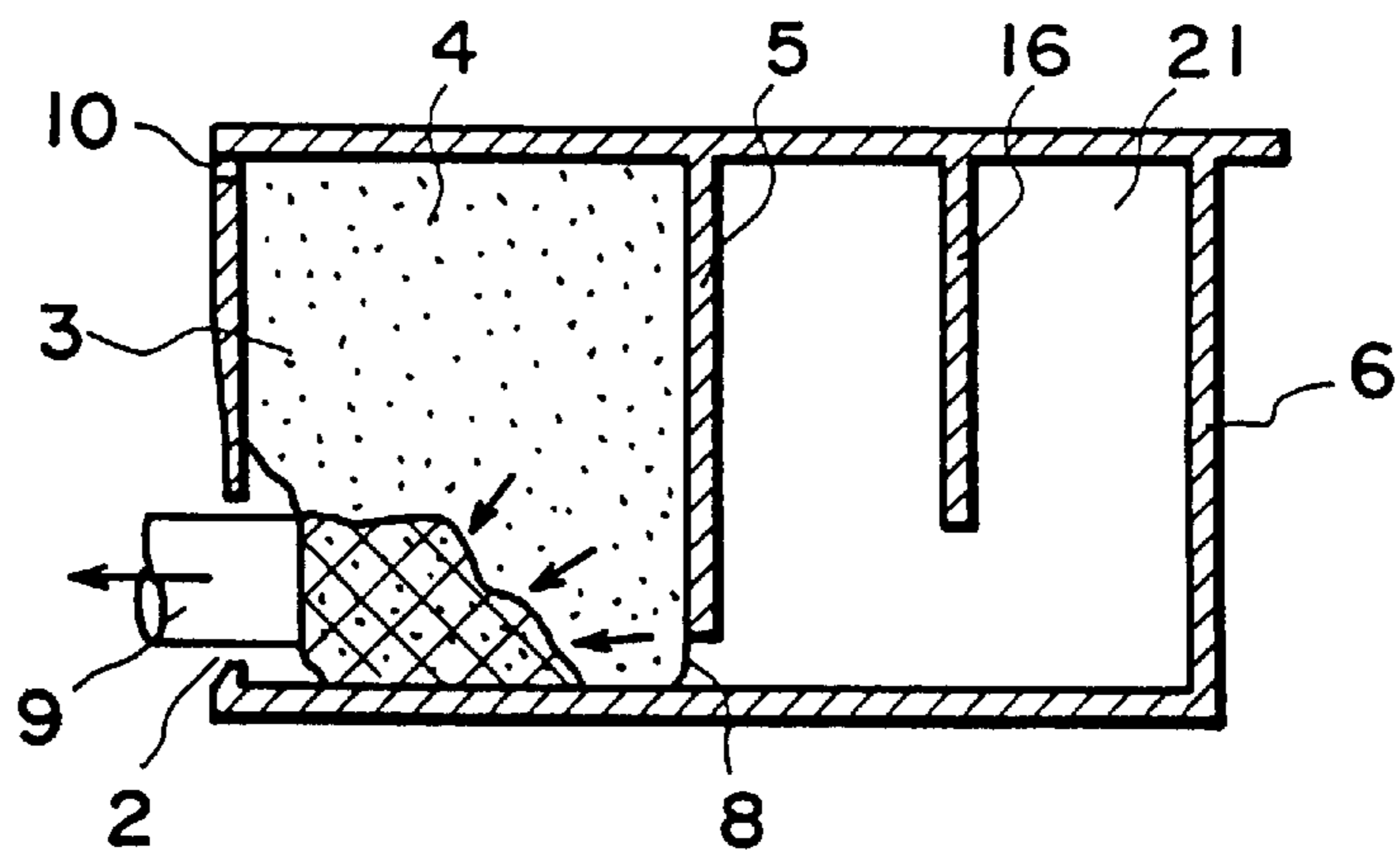
FIG. 3C
