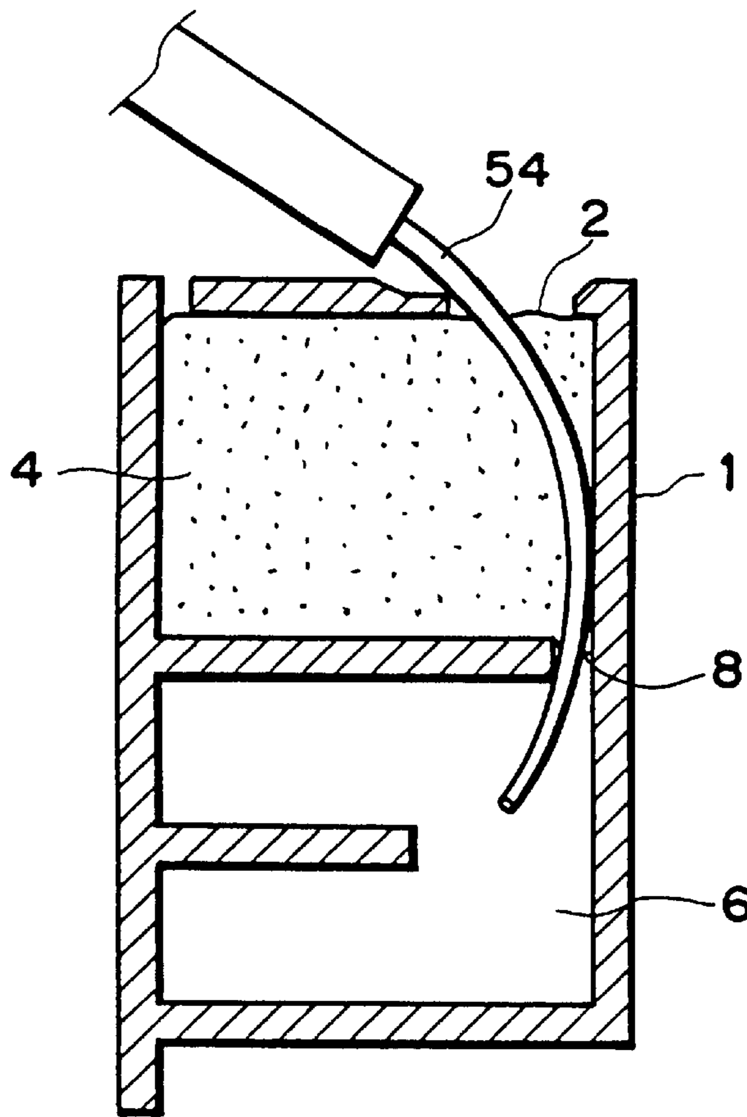
FIG. 31B
