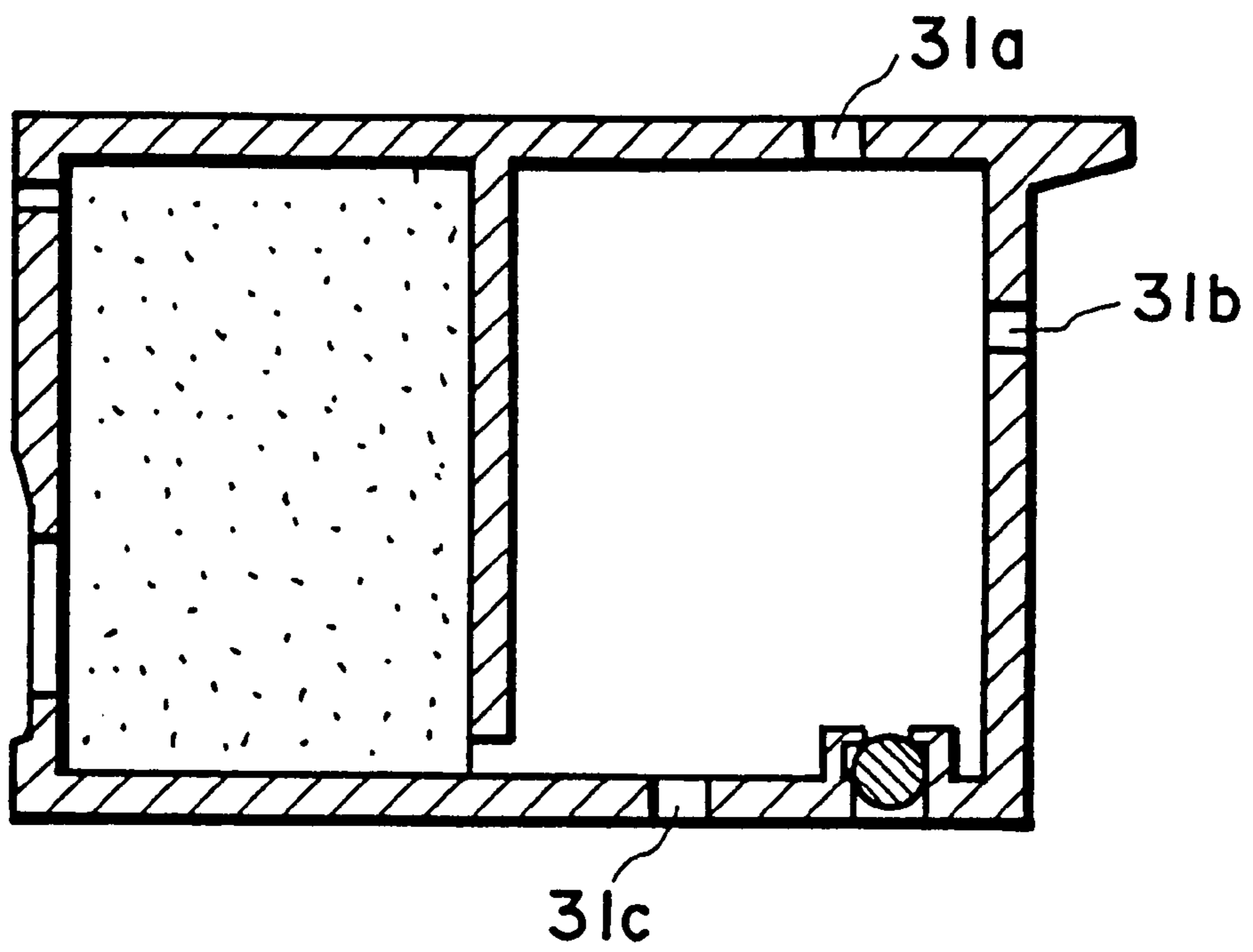
FIG. 14
