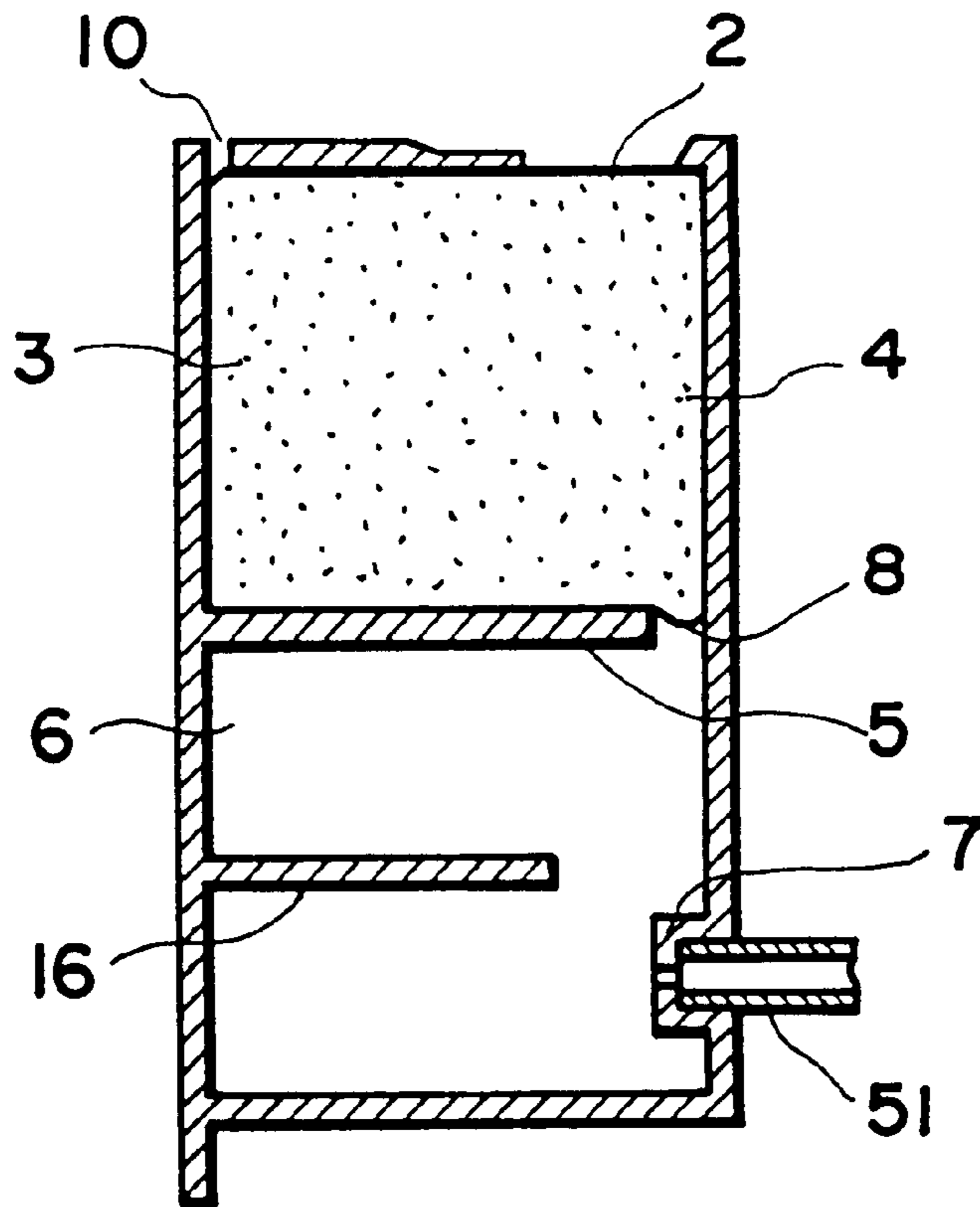
FIG. 24B
