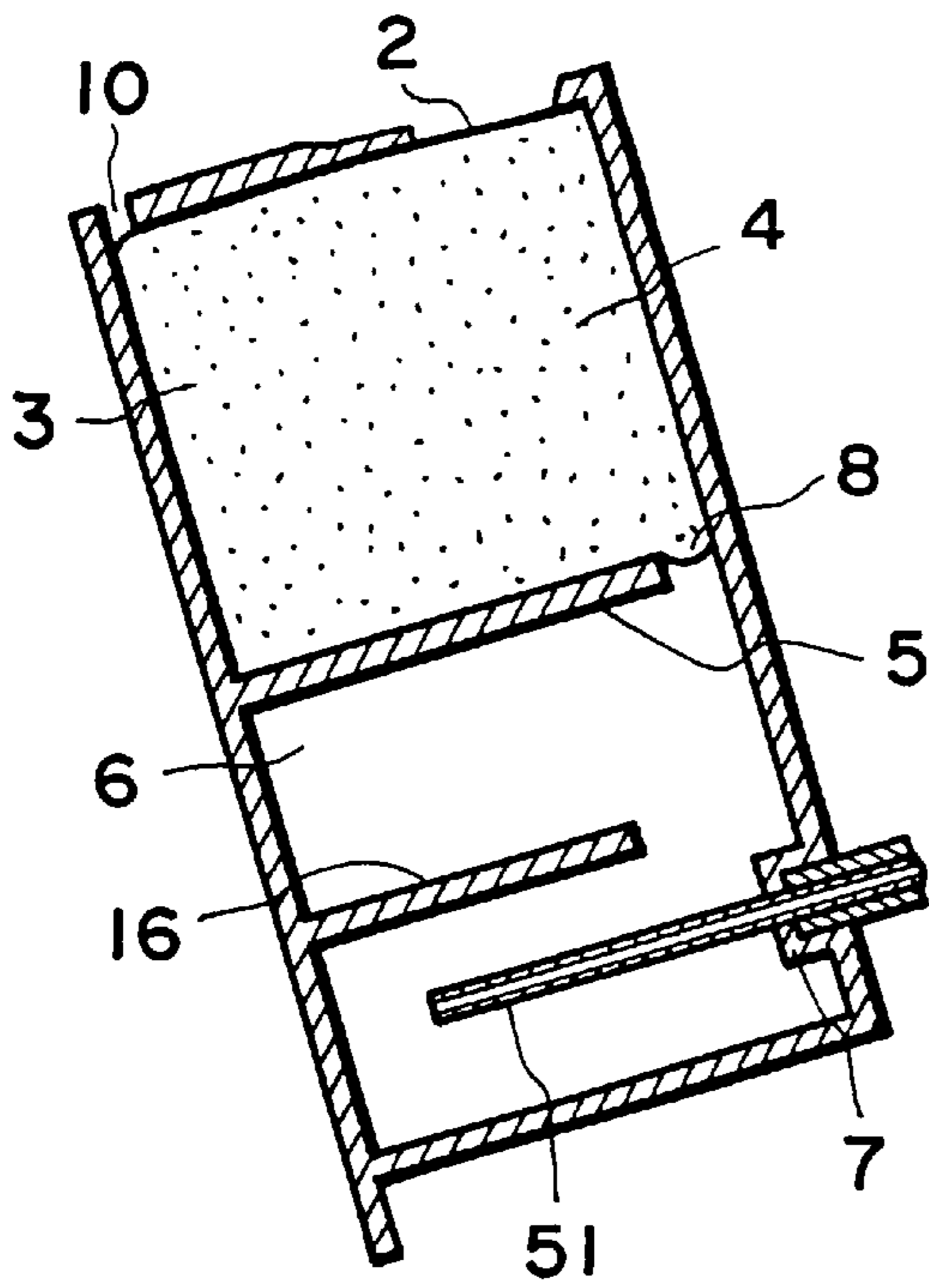
FIG. 25A
