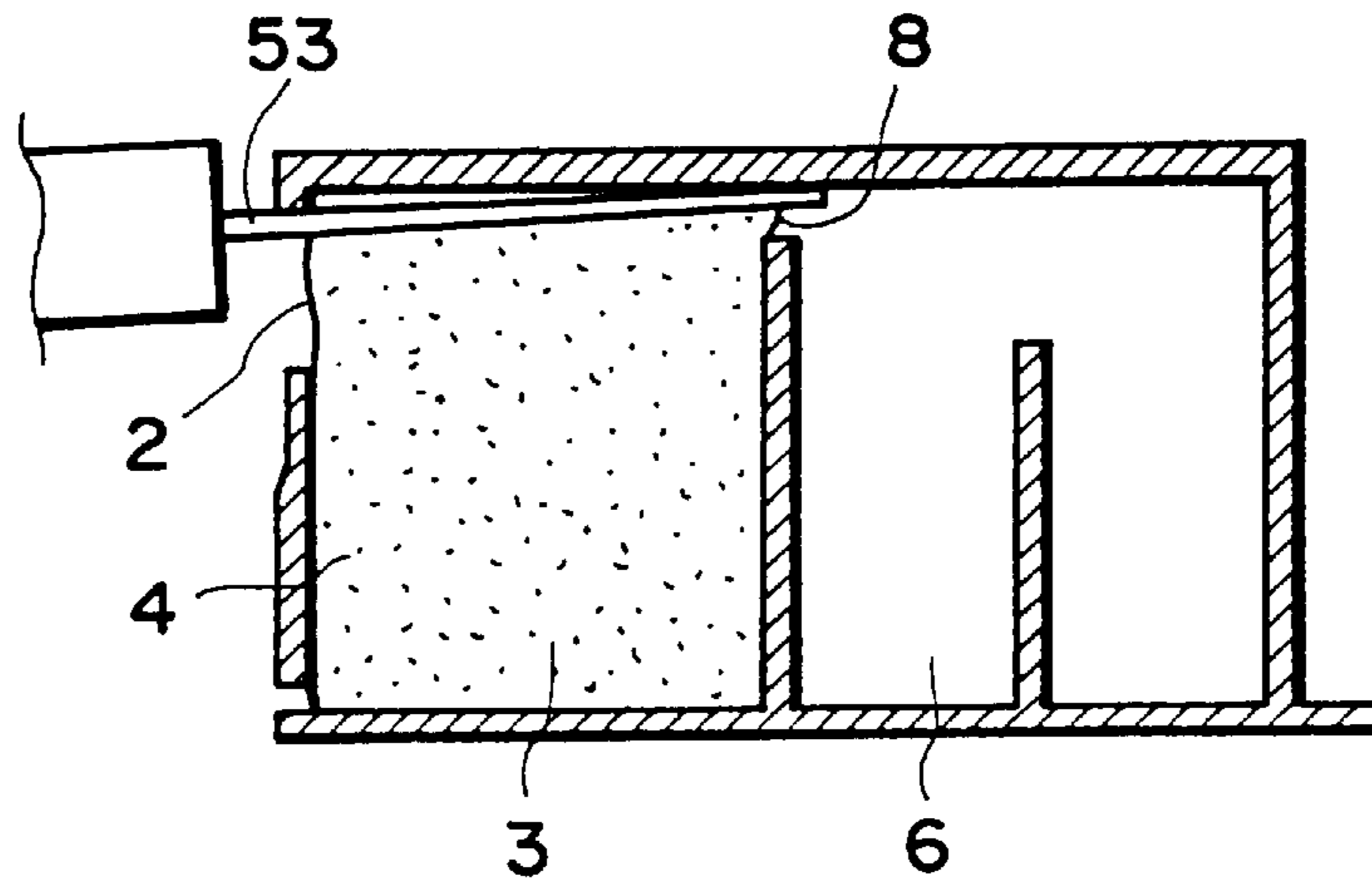
FIG. 30B
