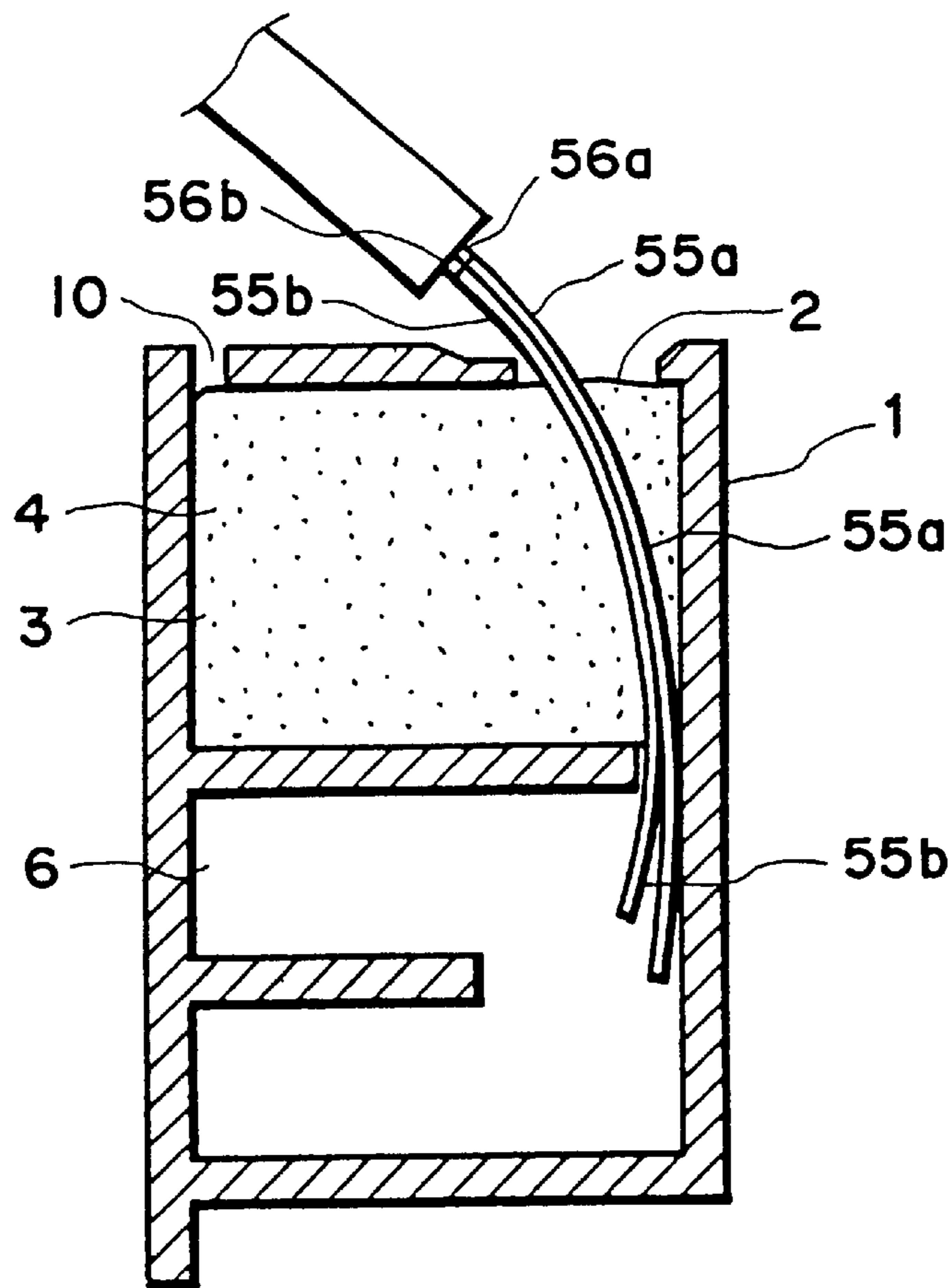
FIG. 32B
