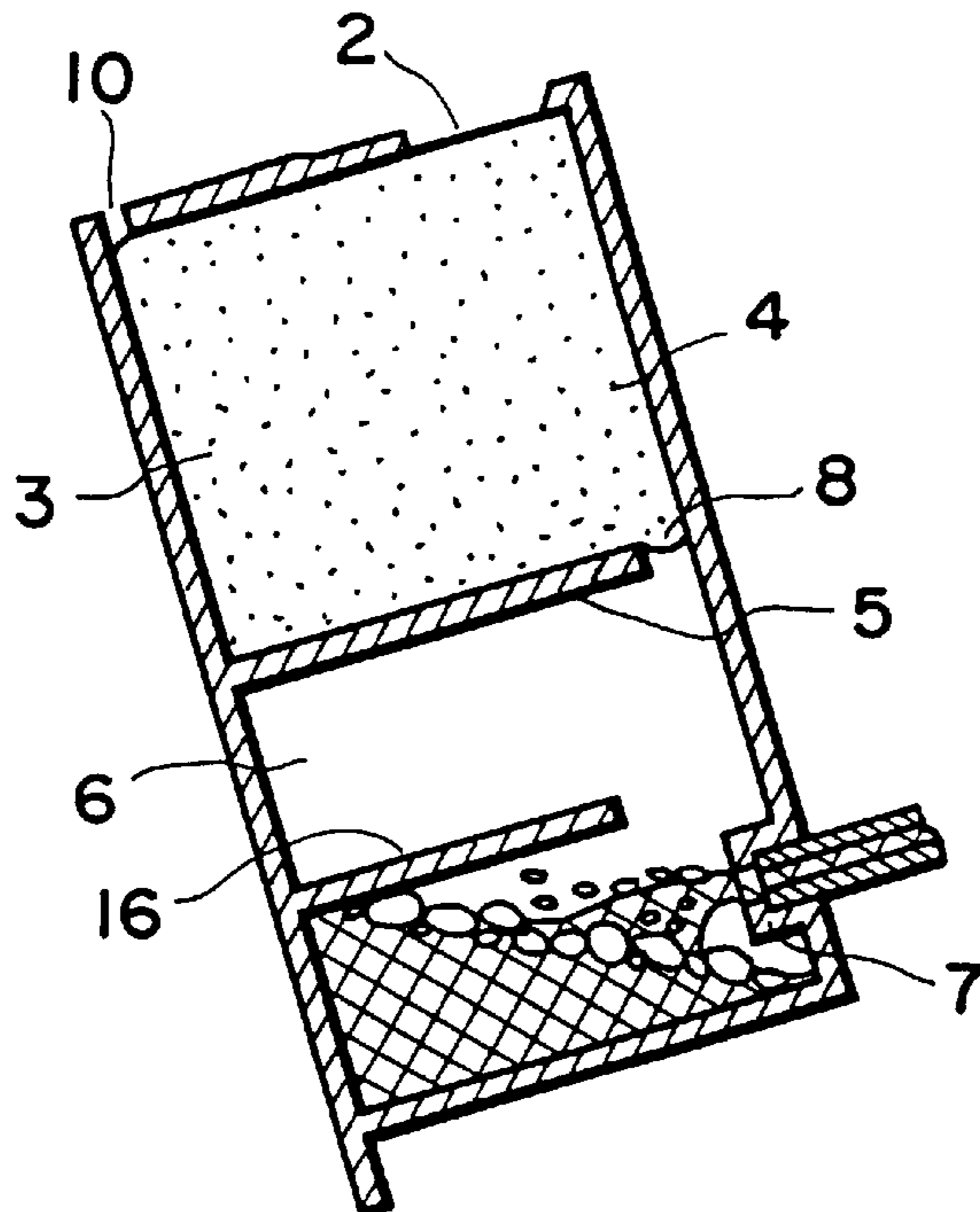
FIG. 26
