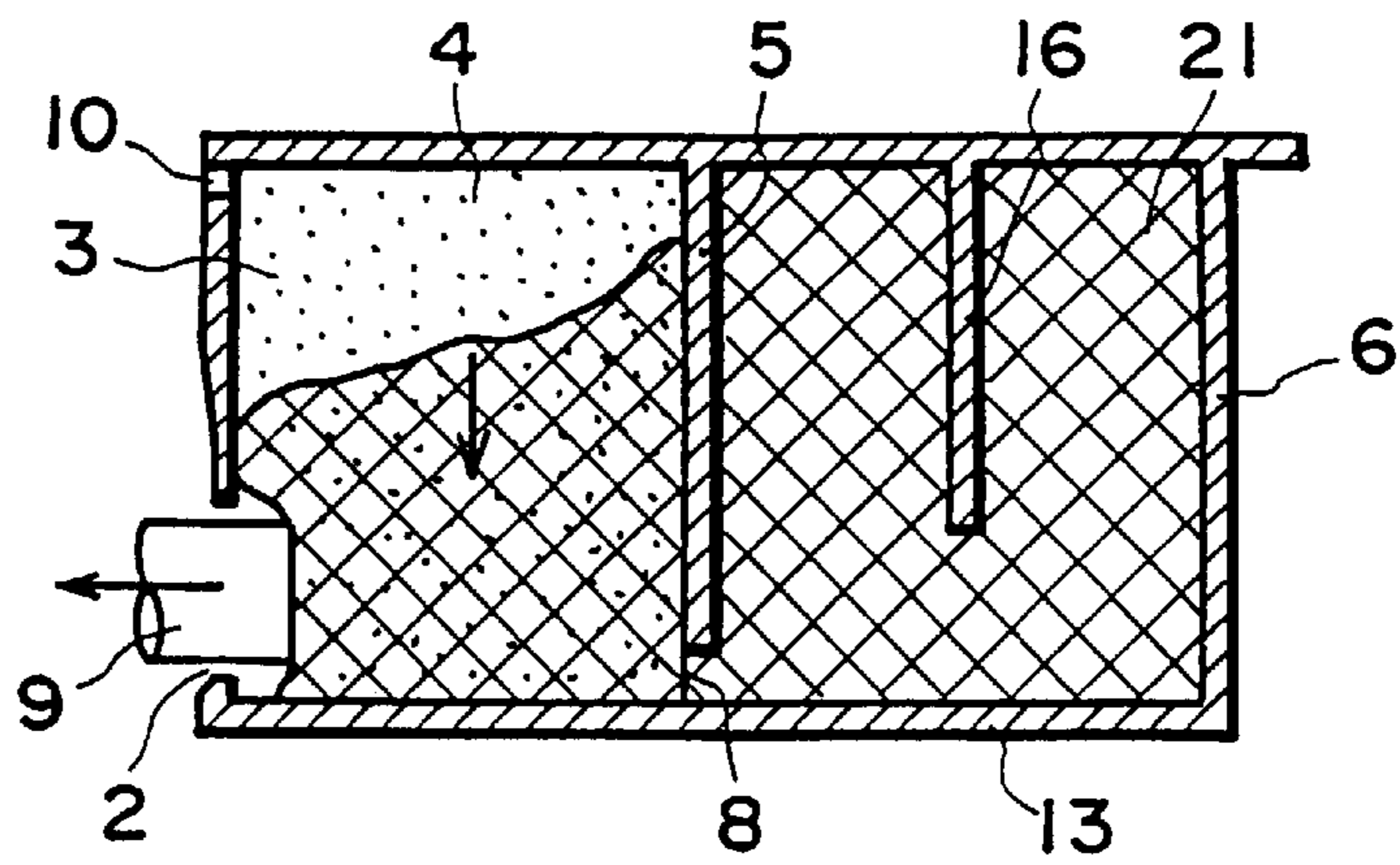
FIG. 3A
