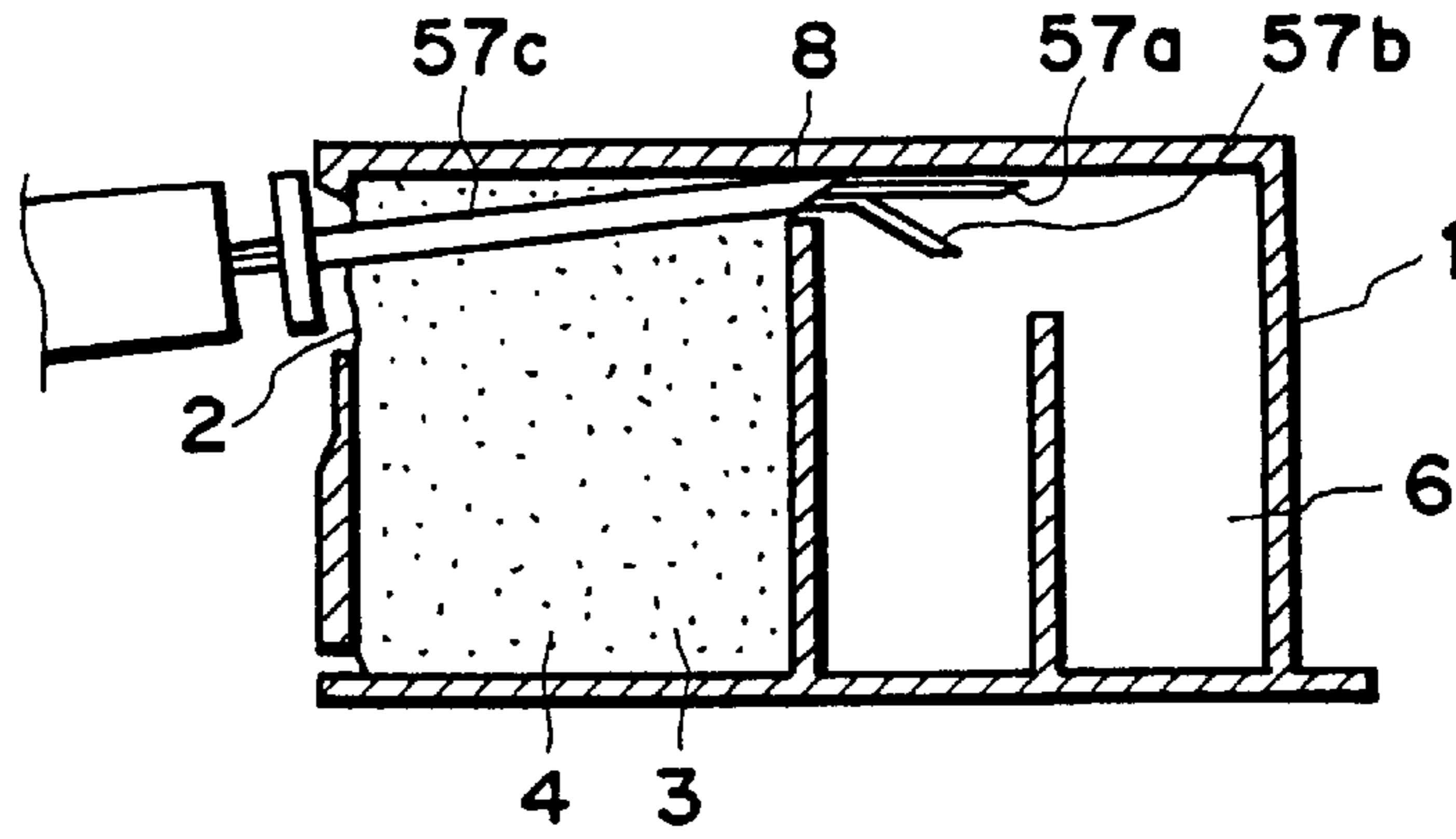
FIG. 33A
