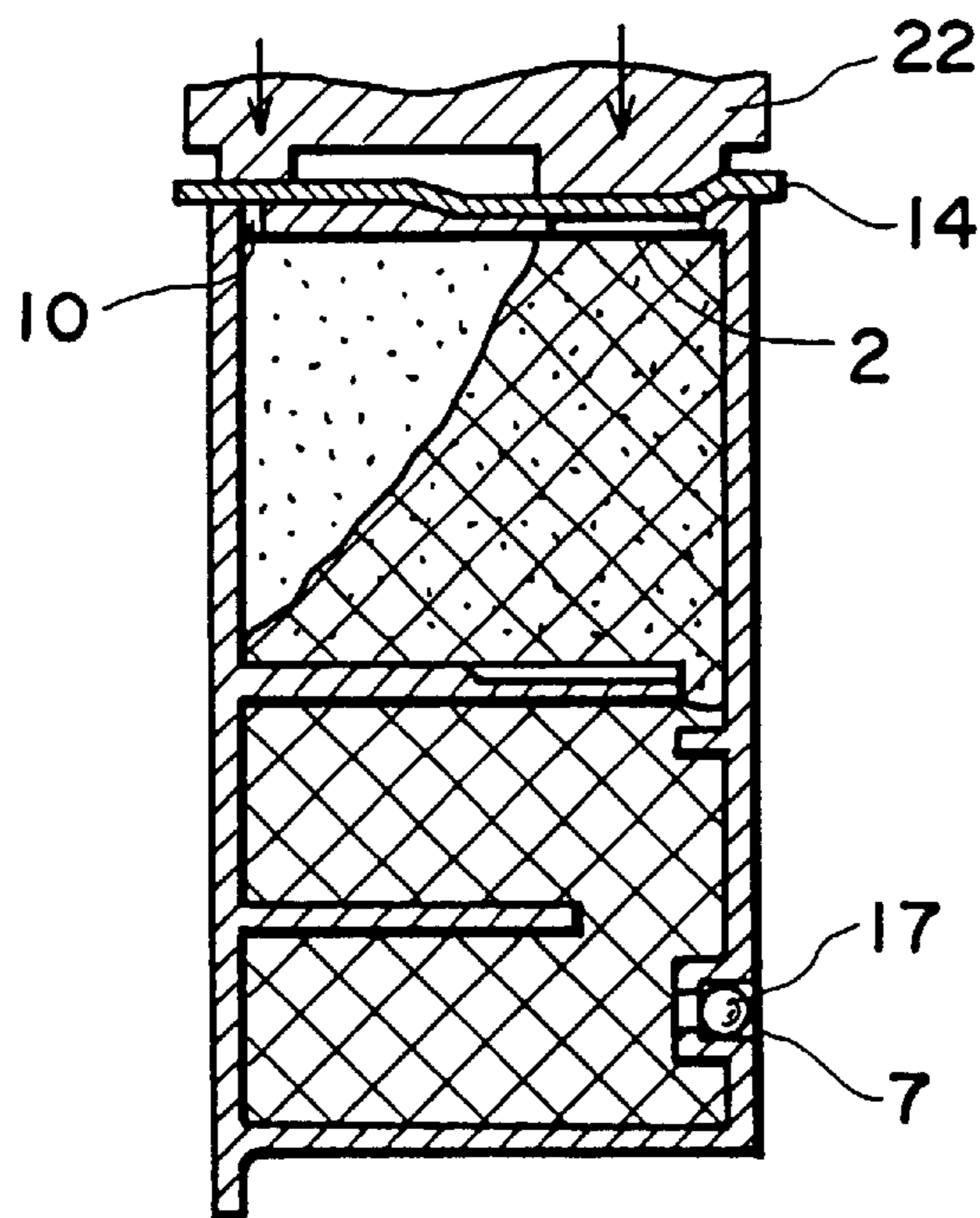
FIG. 10
