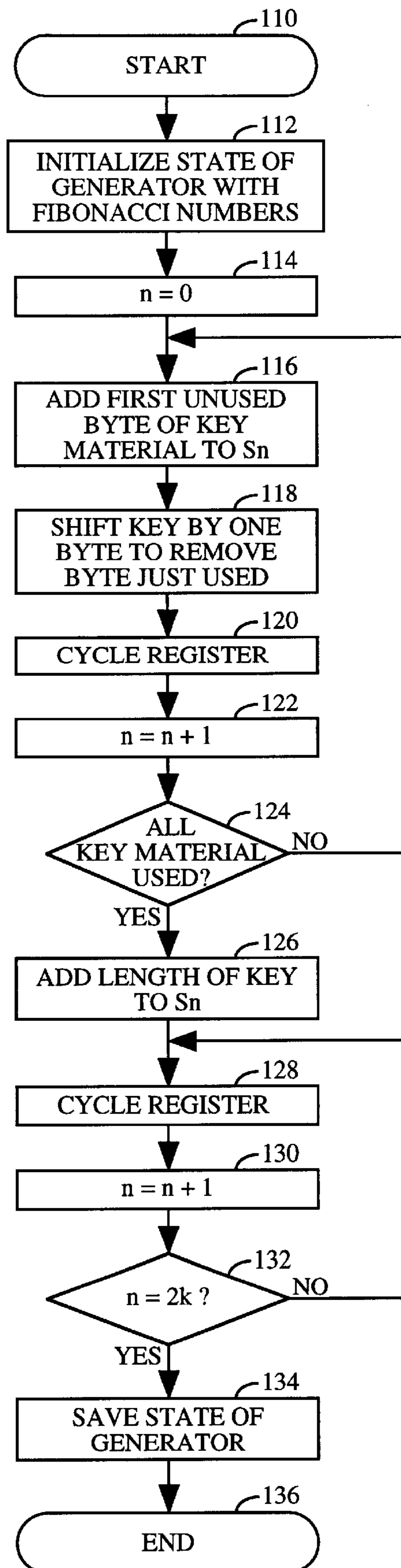
FIG. 5
