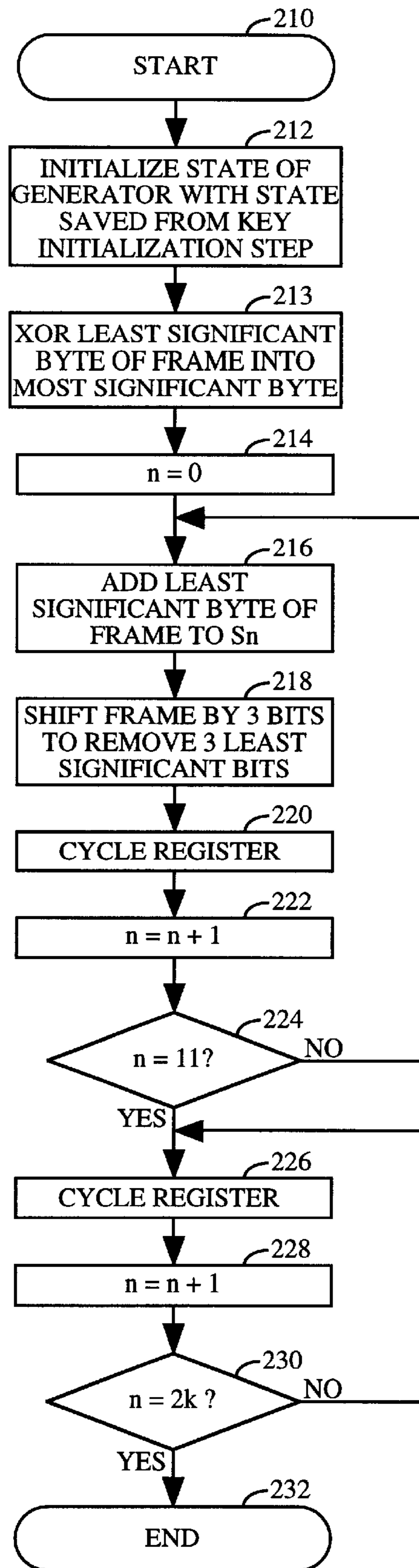
FIG. 8
