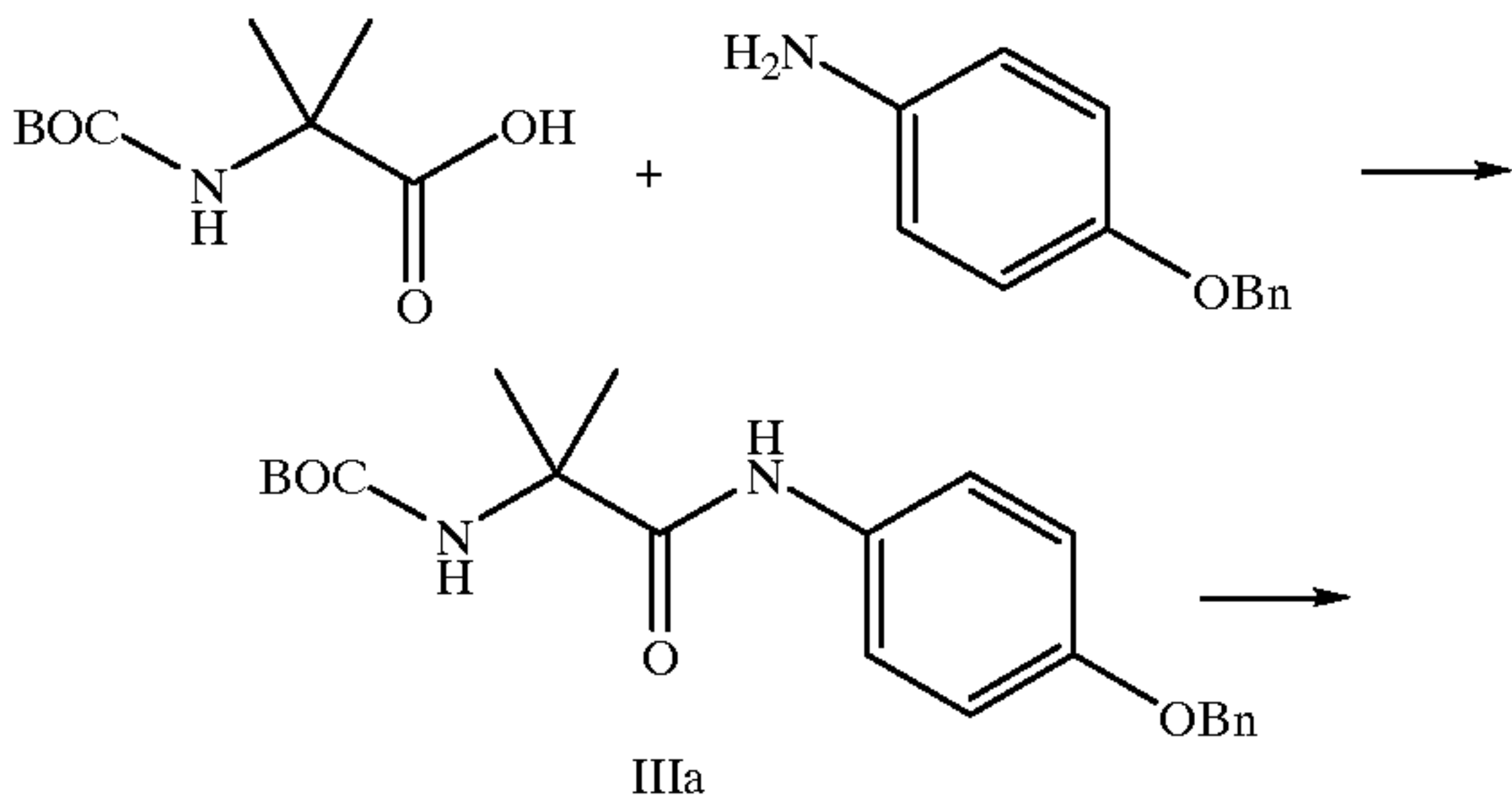
Scheme VI
